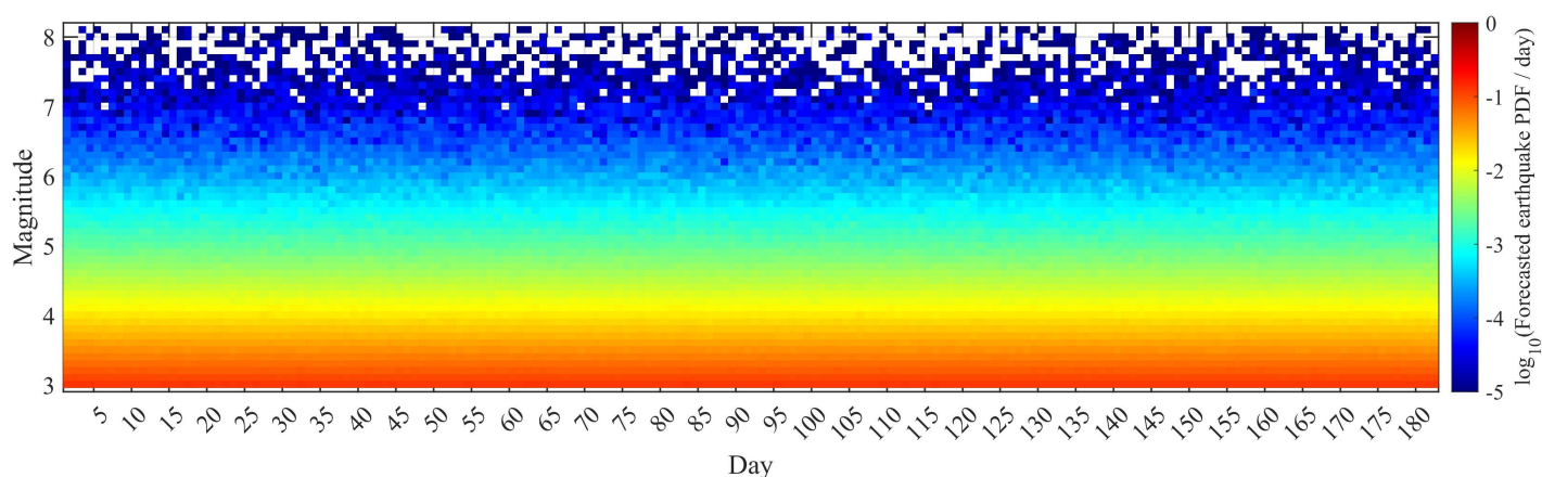
图3. 未来半年中国地震科学实验场内预测地震数目每日的概率密度分布 (PDF)。
