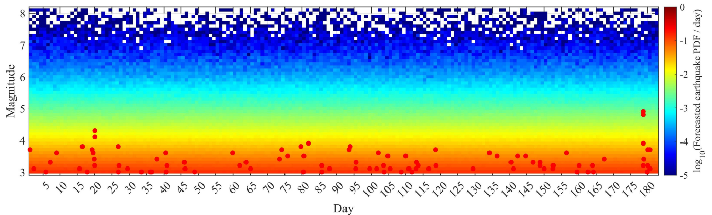
图 8. 过去半年中国地震科学实验场内观测地震活动 (红色实心圆) 的震级时间分布, 背景为半年前预测报告发布的预测地震数目每日概率密度分布 (PDF)。
