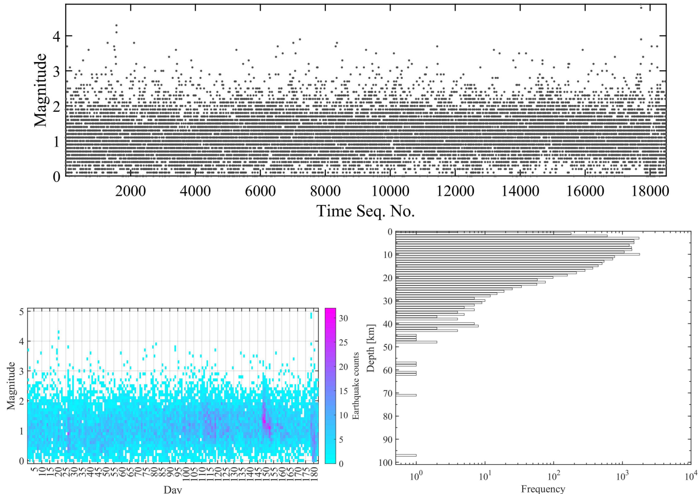
图 4. 过去半年中国地震科学实验场地震活动性的（上）震级-时间序号图；（左下）每 0.1 个震级区间的每日地震数量；（右下）深度-频次分布。
