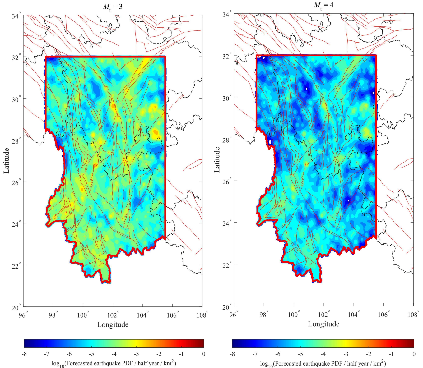
图 2. 未来半年中国地震科学实验场内预测地震数目 ( M \geq M_t ) 每平方公里 ( \text{km}^2 ) 的概率密度分布 (PDF)。
