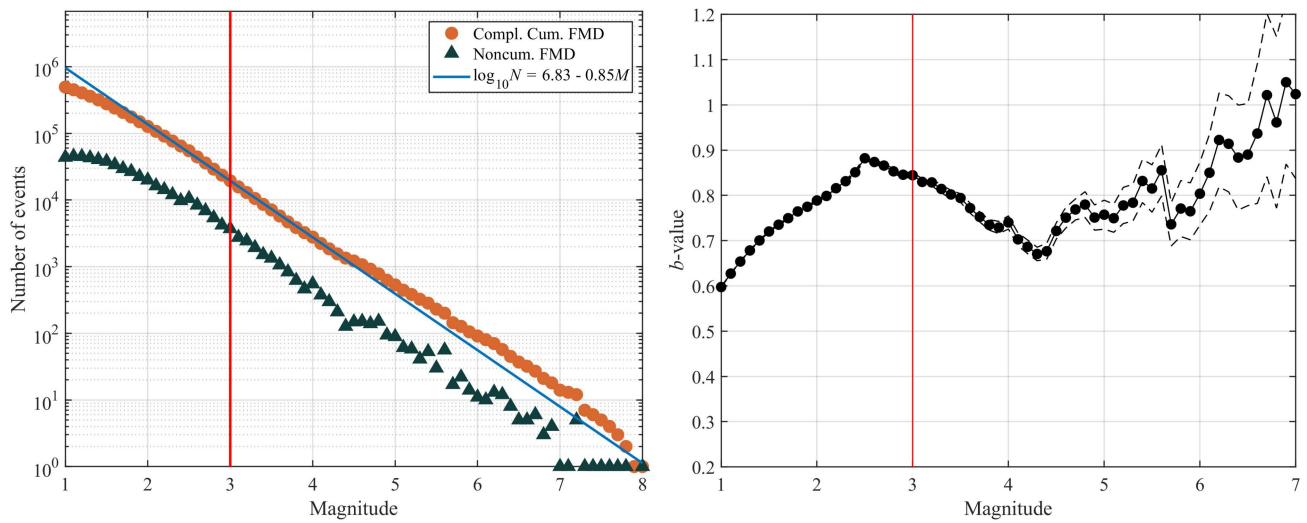
图 12. (左) 1970 年至今中国地震科学实验场内地震事件的互补累积和密度震级-频次分布以及大于目录截止震级 M_{co} = 3.0 (红线) 地震的古登堡-里克特 (GR) 关系拟合结果; (右) 相同地震目录 GR 关系 b 值随 M_{co} 变化的曲线, 其中细虚线表示 \pm 1\sigma 的标准差。估计 b 值和拟合 GR 关系的方法详见 Li 等 (2024) 补充材料。
