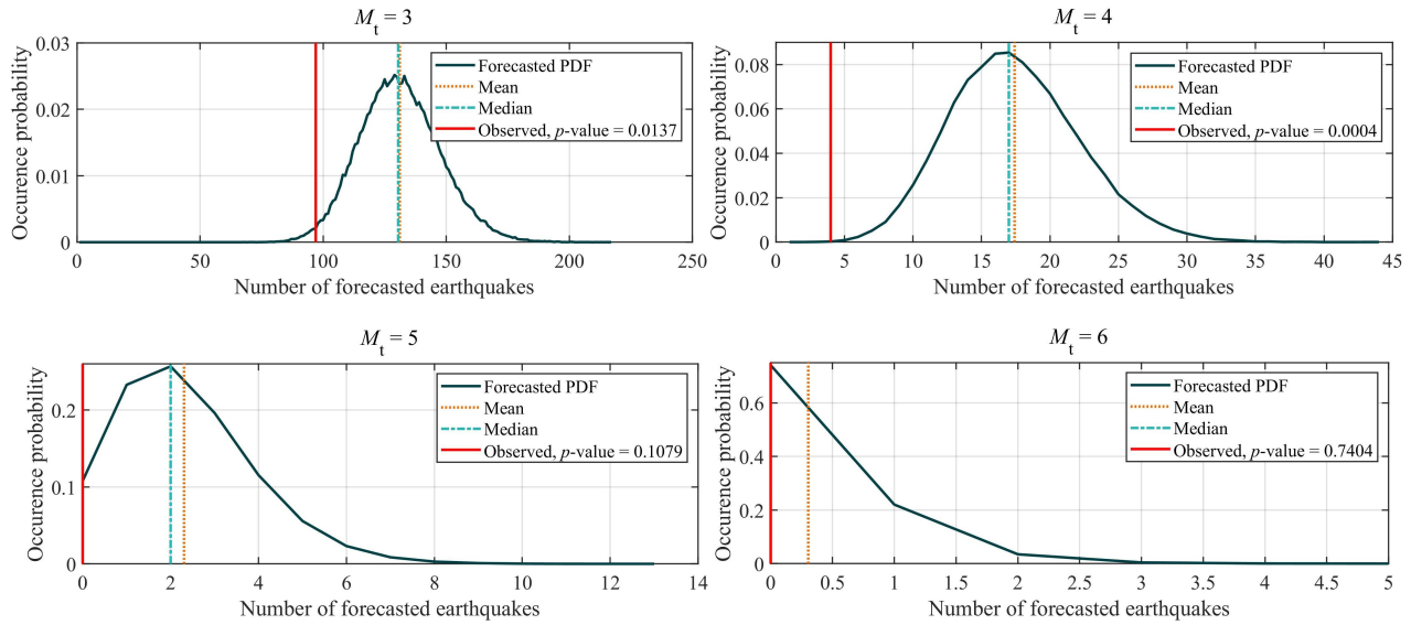
图 6. 过去半年中国地震科学实验场内观测到的不同震级范围 ( M \geq M_t ) 地震数量 (红竖线) 以及半年前发布的地震数目预测概率。 p 值是观测地震数目的累积分布函数。
