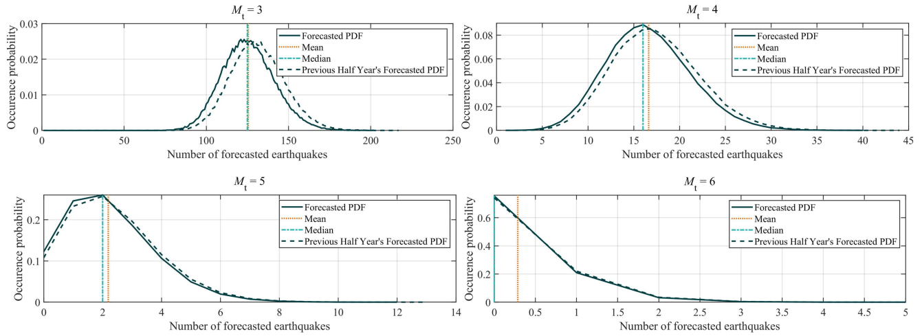
图 1. 未来半年中国地震科学实验场（川滇地区）内不同震级范围 ( M \geq M_t ) 的地震数目预测概率。
