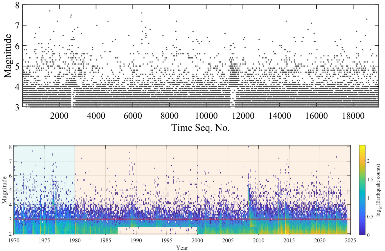
图 10. 中国地震科学实验场内自 1970 年以来地震活动性的 (上) 震级序号图及 (下) 每 0.1 个震级区间的每月地震数量。红线表示截止震级 M_{co} = 3.0 。浅红色和浅蓝色背景区域分别为主时段和辅助时段。截止震级 M_{co} 、主时段和辅助时段等参数均用于 ETAS 模型参数反演和预测模拟的构建。
