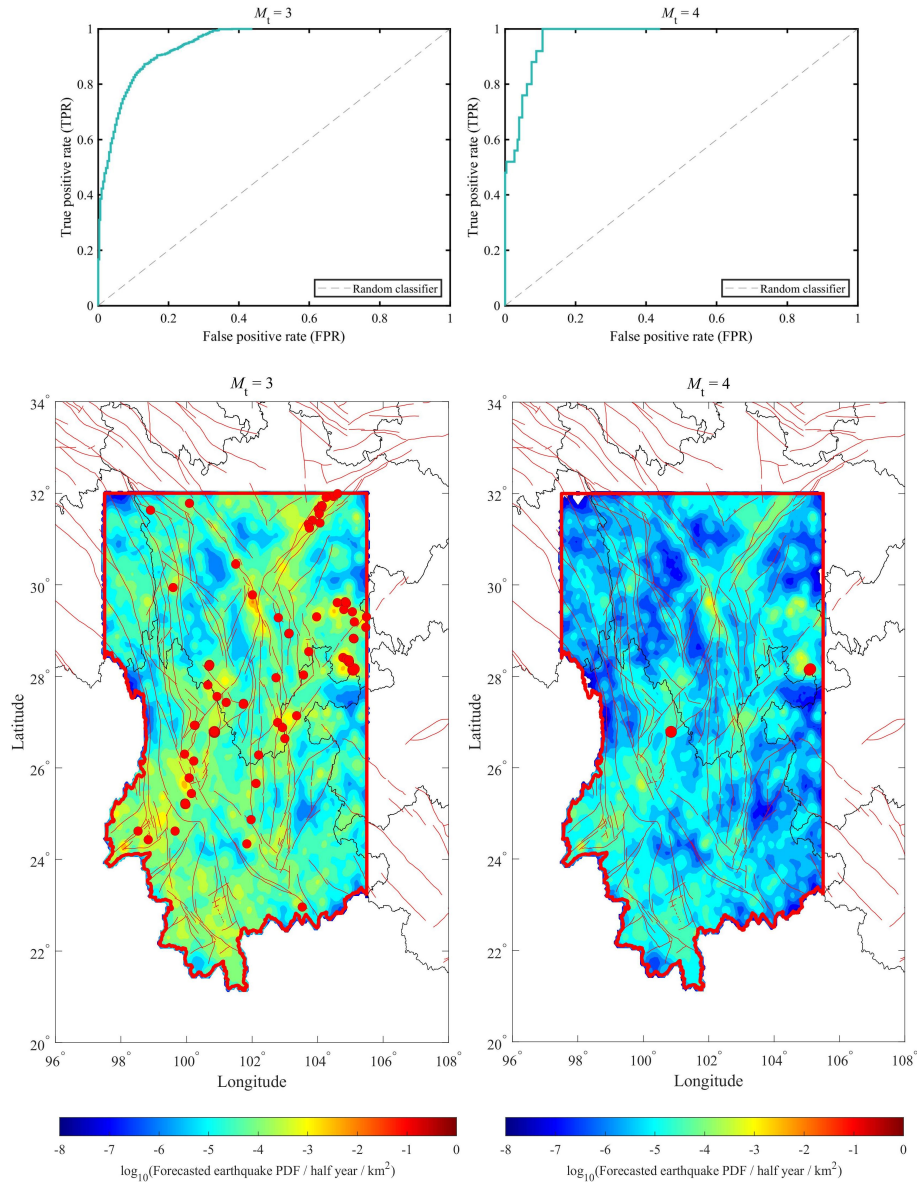
图 7. (上图) 受试者操作特征 (ROC) 曲线和 (下图) 为半年前预测报告发布的预测地震数目 ( M \geq M_t ) 每平方公里 ( \text{km}^2 ) 概率密度分布 (PDF)。红色实心圆为过去半年中国地震科学实验场内观测的地震活动。
