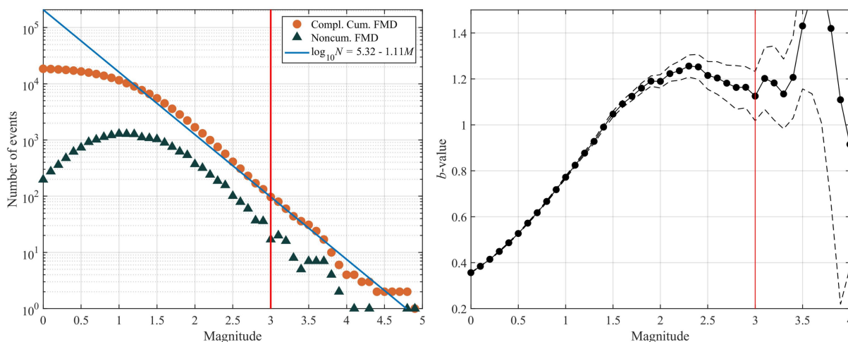
图 5. 过去半年中国地震科学实验场地震活动性的（左）互补累积和密度震级-频次分布以及大于目录截止震级 M_{co} = 3.0 （红线）地震的古登堡-里克特（GR）关系拟合结果；（右）GR 关系 b 值随 M_{co} 变化的曲线，其中细虚线表示 \pm 1\sigma 的标准差。
