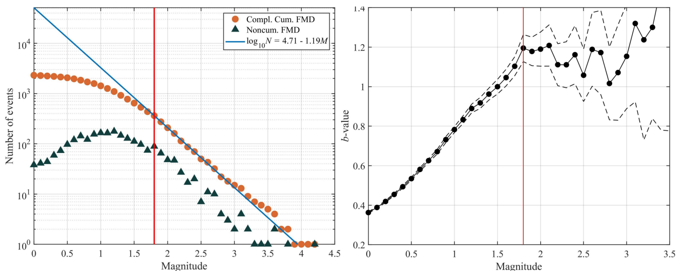
图 5. 过去一个月中国地震科学实验场地震活动性的（左）互补累积和非累积震级-频次分布及大于过去一个月的目录最小完整性震级 M_c （红竖线）地震的古登堡-里克特（GR）关系拟合结果；（右） b 值随目录截止震级 M_{co} 变化的曲线，其中细虚线表示 \pm 1\sigma 的标准差。
