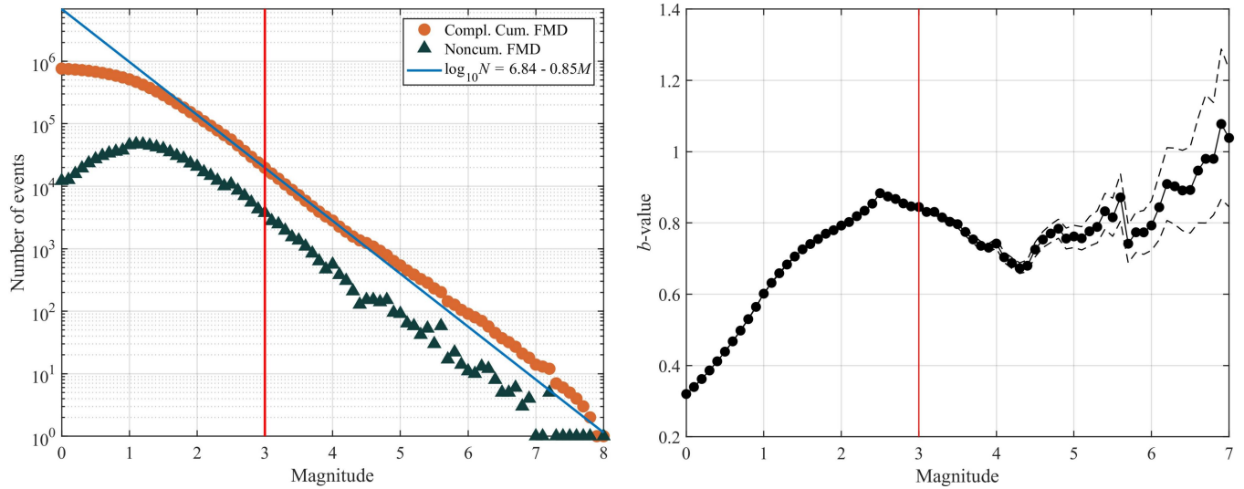
图 12. (左) 1970 年至今中国地震科学实验场内地震事件的互补累积和非累积震级-频次分布以及大于目录截止震级 M_{co} = 3.0 (红线) 地震的古登堡-里克特 (GR) 关系拟合结果; (右) 相同地震目录 b 值随 M_{co} 变化的曲线, 其中细虚线表示 \pm 1\sigma 的标准差。估计 b 值和拟合 GR 关系的方法详见 Li 等 (2025) 补充材料。
