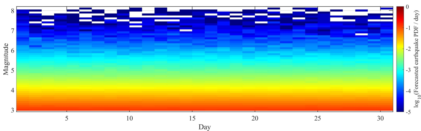
图 3. 未来一个月中国地震科学实验场内预测地震每日的概率密度分布 (PDF)。
