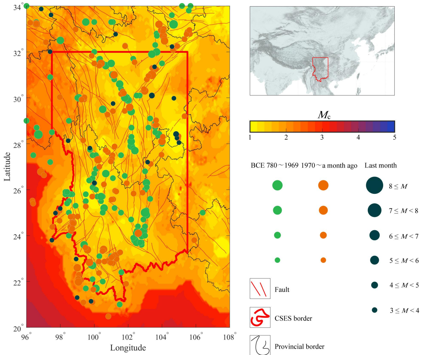
图 9. 中国地震科学实验场（川滇地区）内历史地震和活动断层空间分布。背景为最小完整性震级 ( M_c ) 的空间分布 (摘自 Li 等, 2023)。
