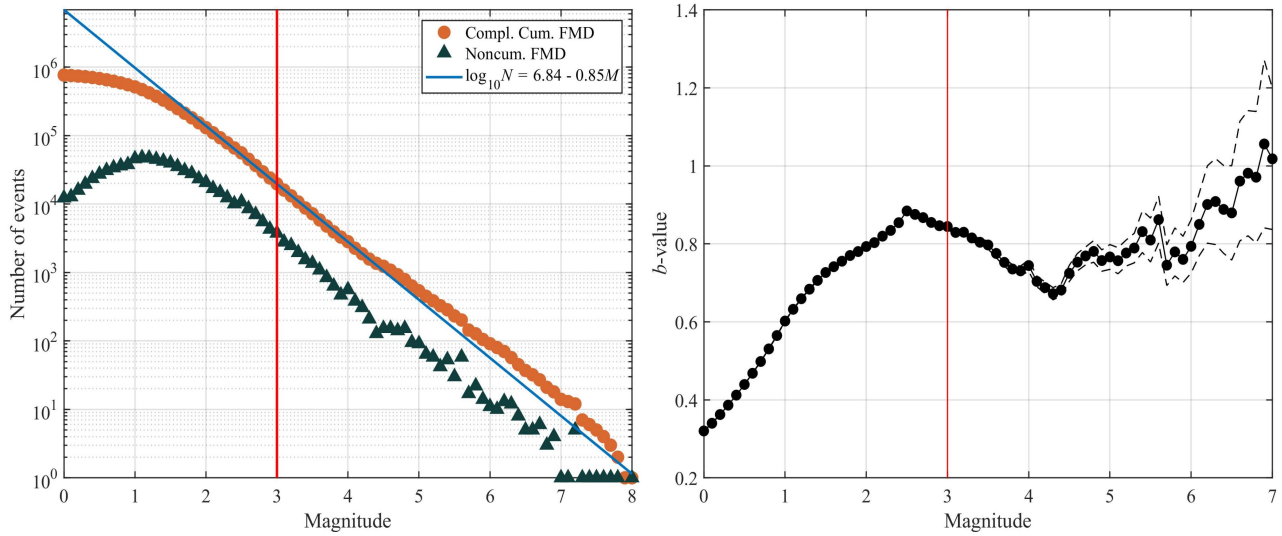
图 12. (左) 1970 年至今中国地震科学实验场内地震事件的互补累积和非累积震级-频次分布以及大于目录截止震级 M_{co} = 3.0 (红线) 地震的古登堡-里克特 (GR) 关系拟合结果; (右) 相同地震目录 b 值随 M_{co} 变化的曲线, 其中细虚线表示 \pm 1\sigma 的标准差。估计 b 值和拟合 GR 关系的方法详见 Li 等 (2025) 补充材料。
