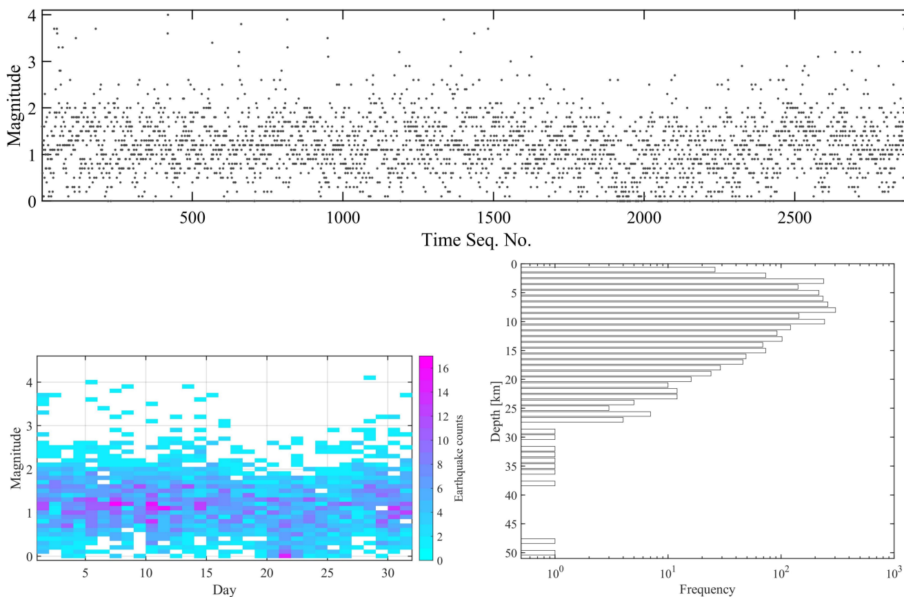
图 4. 过去一个月中国地震科学实验场地震活动性的（上）震级-时间序号图；（左下）每 0.1 个震级区间的每日地震数量；（右下）深度-频次分布。
