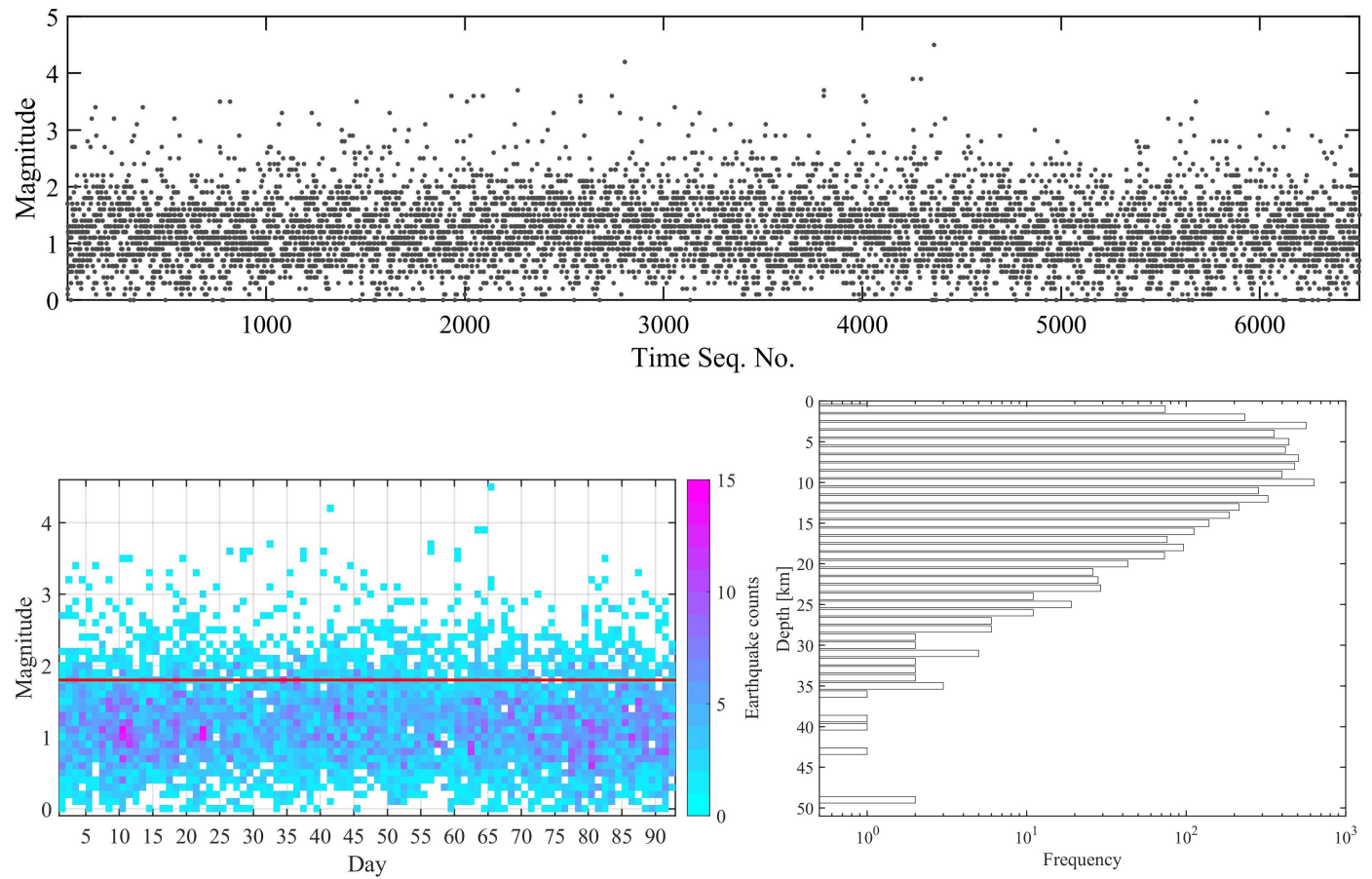
图 4. 过去一个季度中国地震科学实验场地震活动性的（上）震级-时间序号图；（左下）每 0.1 个震级区间的每日地震数量；（右下）深度-频次分布。左下图中的红色直线为过去一个季度的目录最小完整性震级 ( M_c )。
