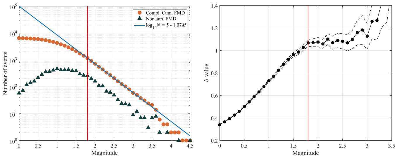
图 5. 过去一个季度中国地震科学实验场地震活动性的（左）互补累积和密度震级-频次分布以及大于过去一个季度的目录最小完整性震级 M_c （红竖线）地震的古登堡-里克特（GR）关系拟合结果；（右） b 值随目录截止震级 M_{co} 变化的曲线，其中细虚线表示 \pm 1\sigma 的标准差。
