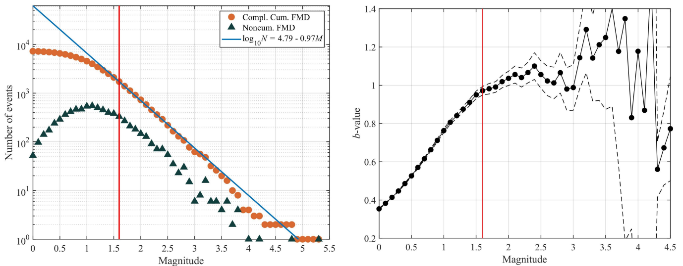
图 5. 过去一个季度中国地震科学实验场地震活动性的（左）互补累积和密度震级-频次分布以及大于过去一个季度的目录最小完整性震级 M_c （红竖线）地震的古登堡-里克特（GR）关系拟合结果；（右） b 值随目录截止震级 M_{\infty} 变化的曲线，其中细虚线表示 \pm 1\sigma 的标准差。
