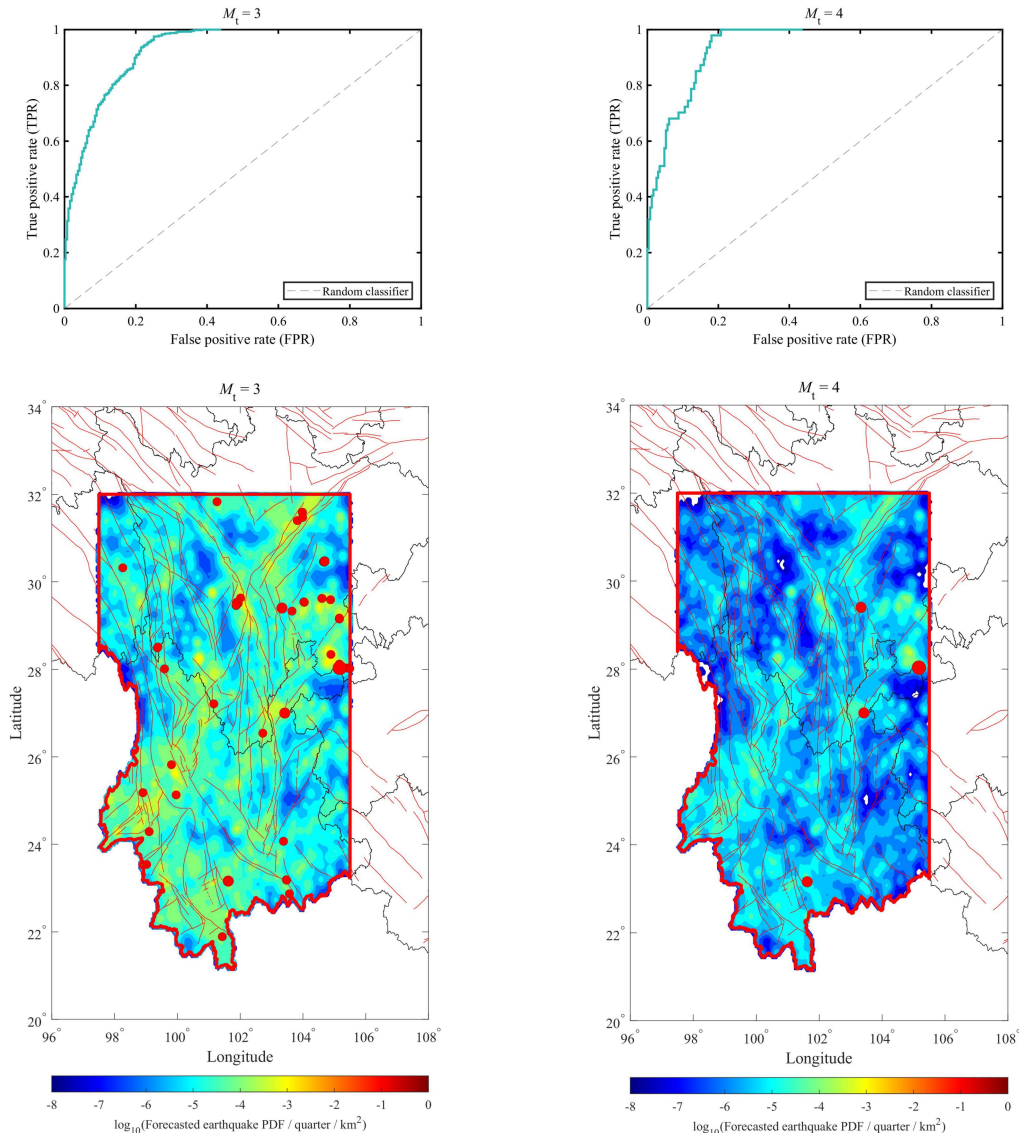
图 7. 过去一个季度中国地震科学实验场内观测地震活动 (红色实心圆) 的空间分布及其受试者操作特征 (ROC) 曲线 (正上方插图)。下图背景为上个季度预测报告发布的预测地震 ( M \geq M_t ) 每平方公里 ( \text{km}^2 ) 概率密度分布 (PDF)。
