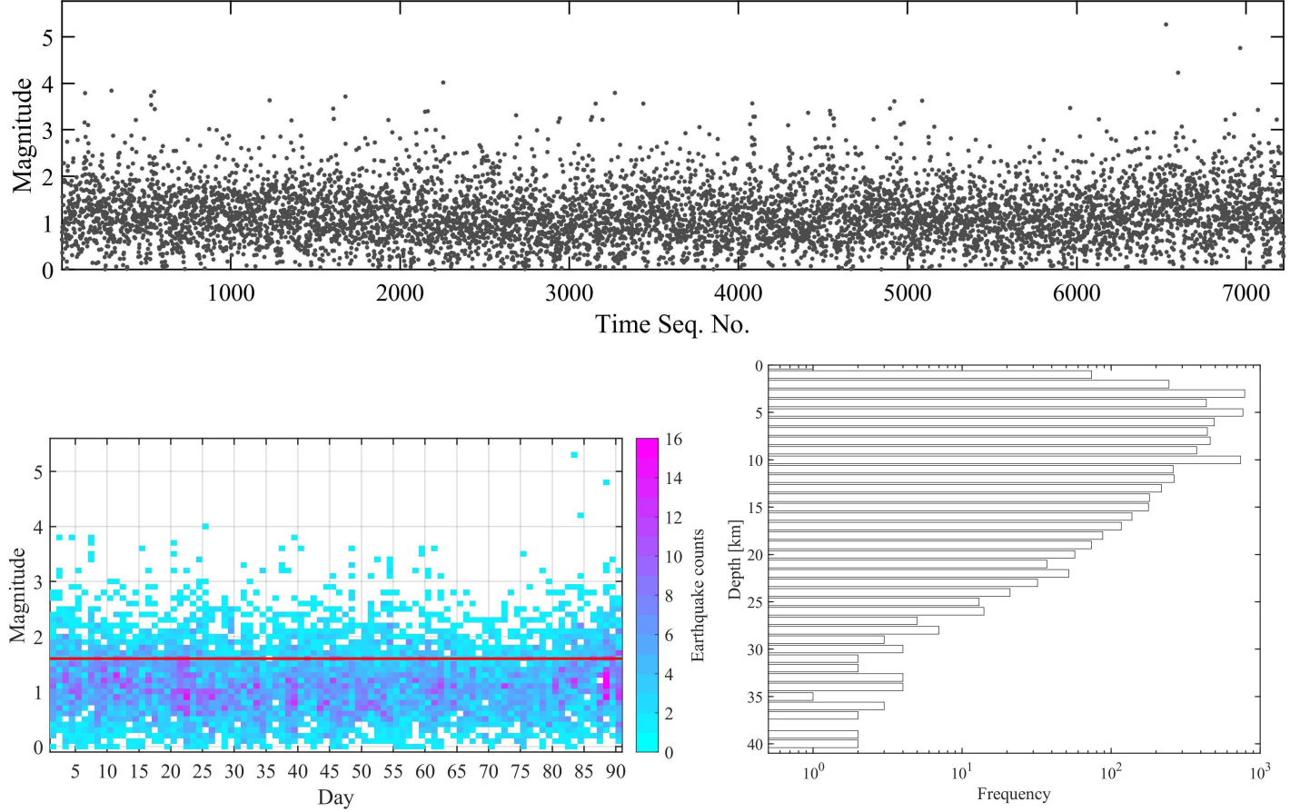
图 4. 过去一个季度中国地震科学实验场地震活动性的（上）震级-时间序号图；（左下）每 0.1 个震级区间的每日地震数量；（右下）深度-频次分布。震级-时间序号图中的震级被添加了 [-0.05, 0.05] 均匀分布的随机误差。左下图中的红色直线为过去一个季度的目录最小完整性震级 ( M_c )。
