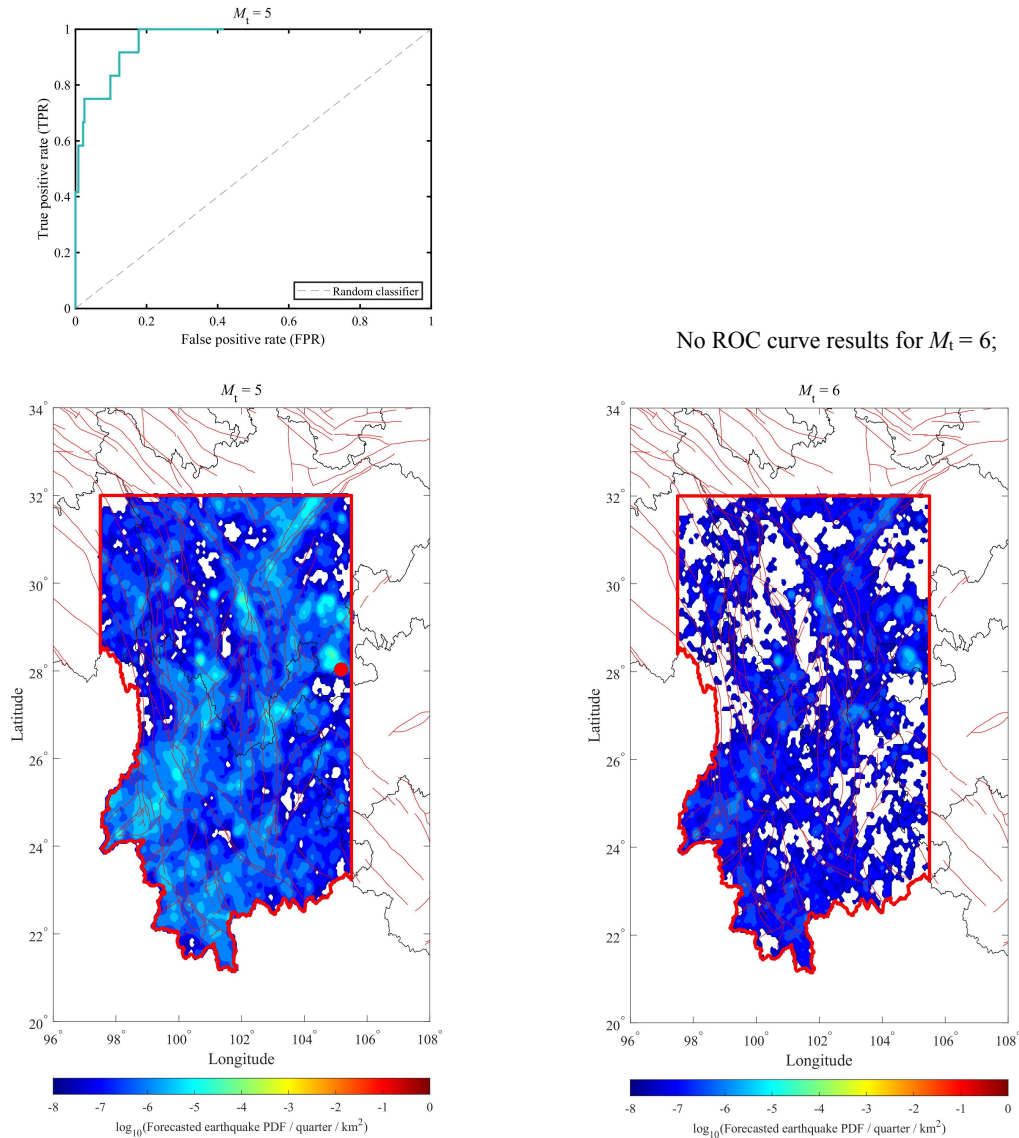
图 7.-同上。ROC 曲线是通过遍历所有预测的地震概率密度值并按降序计算出。对于每个概率密度阈值，计算真实发生地震所占网格的真阳性率 (TPR) 和假阳性率 (FPR)。在这种情况下，ROC 曲线是基于上个季度预测报告发布的预测地震 ( M \geq M_t ) 每平方公里概率密度分布所构建。这个过程涉及通过将预测的概率密度与该期间内实际发生的地震进行比较来评估预测模型的性能。
