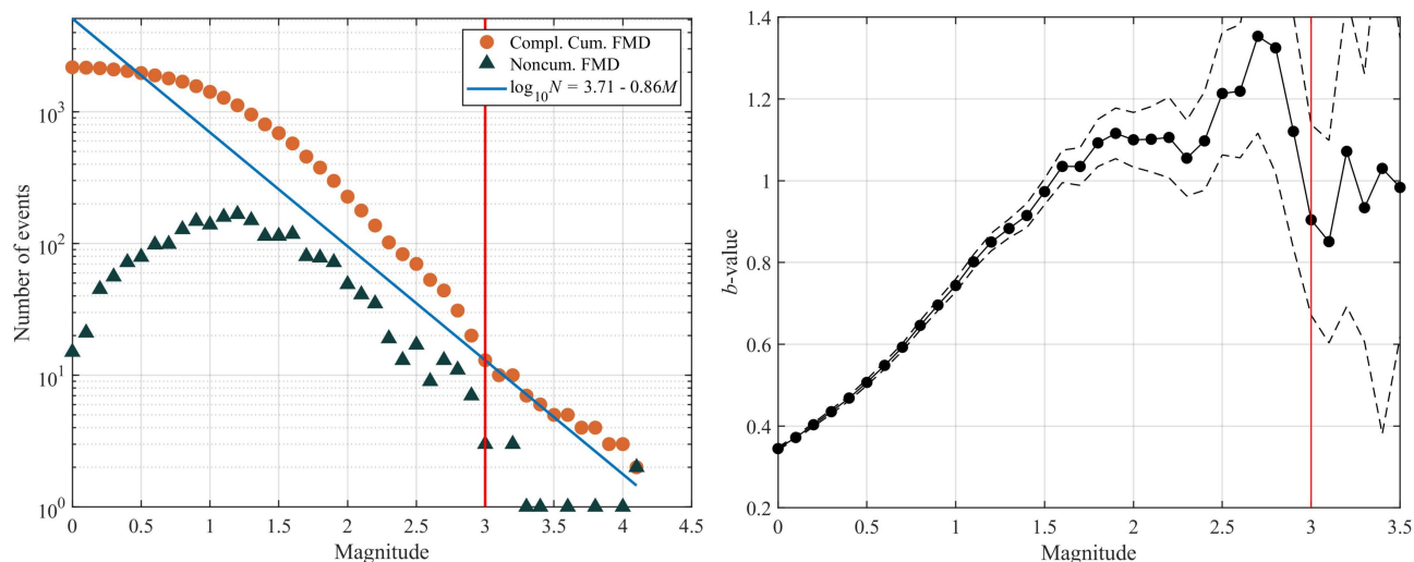
图 5. 过去一个月中国地震科学实验场地震活动性的（左）互补累积和密度震级-频次分布以及大于目录截止震级 M_{\infty} = 3.0 （红线）地震的古登堡-里克特（GR）关系拟合结果；（右） b 值随 M_{\infty} 变化的曲线，其中细虚线表示 \pm 1\sigma 的标准差。
