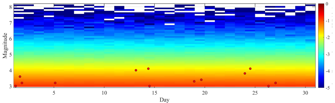
图 8. 过去一个月中国地震科学实验场内观测地震活动（红色实心圆）的震级时间分布，背景为上个月度预测报告发布的预测地震每日概率密度分布（PDF）。
