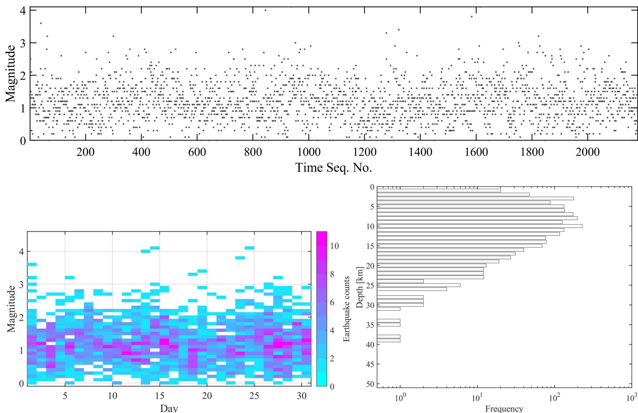
图 4. 过去一个月中国地震科学实验场地震活动性的（上）震级-时间序号图；（左下）每 0.1 个震级区间的每日地震数量；（右下）深度-频次分布。
