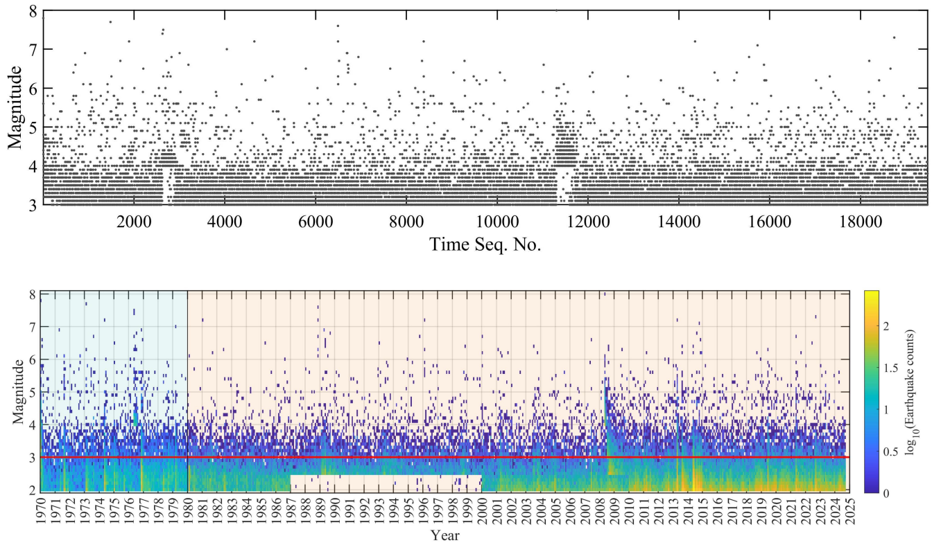
图 10. 中国地震科学实验场内自 1970 年以来地震活动性的 (上) 震级序号图及 (下) 每 0.1 个震级区间的每月地震数量。红线表示截止震级 M_{co} = 3.0 。浅红色和浅蓝色背景区域分别为主时段和辅助时段。截止震级 M_{co} 、主时段和辅助时段等参数均用于 ETAS 模型参数反演和预测模拟的构建。
