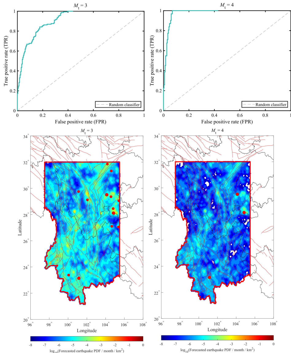
图 7. 过去一个月中国地震科学实验场内观测地震活动 (红色实心圆) 的空间分布及其受试者操作特征 (ROC) 曲线 (正上方插图)。下图背景为上个月度预测报告发布的预测地震 ( M \geq M_t ) 每平方公里 ( \text{km}^2 ) 概率密度分布 (PDF)。
