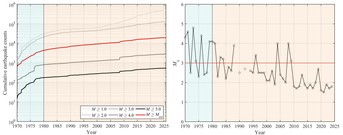
图 11. (左) 中国地震科学实验场内不同截止震级 ( M_{co} = 1, 2, 3, 4 和 5) 的累积地震计数时间序列; (右) 最小完整性震级 ( M_c ) 的时间变化曲线。估计 M_c 的方法详见 Li 等 (2024) 补充材料。
