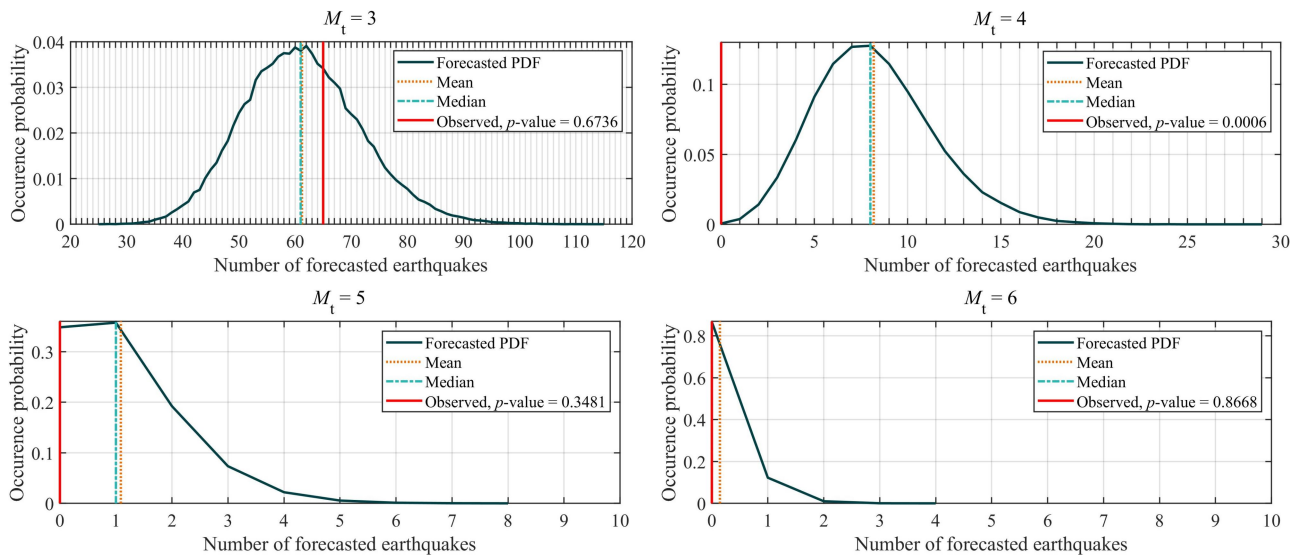
图 6. 过去一个季度中国地震科学实验场内观测到的不同震级范围 ( M \geq M_t ) 地震数量 (红竖线) 以及上个季度发布的地震数目预测概率。 p 值是观测地震数目的累积分布函数。
