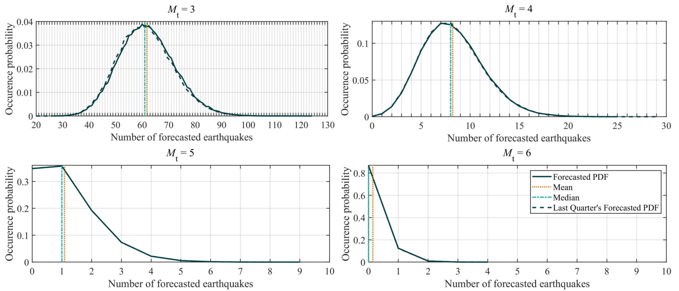
图 1. 未来一个季度中国地震科学实验场（川滇地区）内不同震级范围 ( M \geq M_t ) 的地震数目预测概率。
