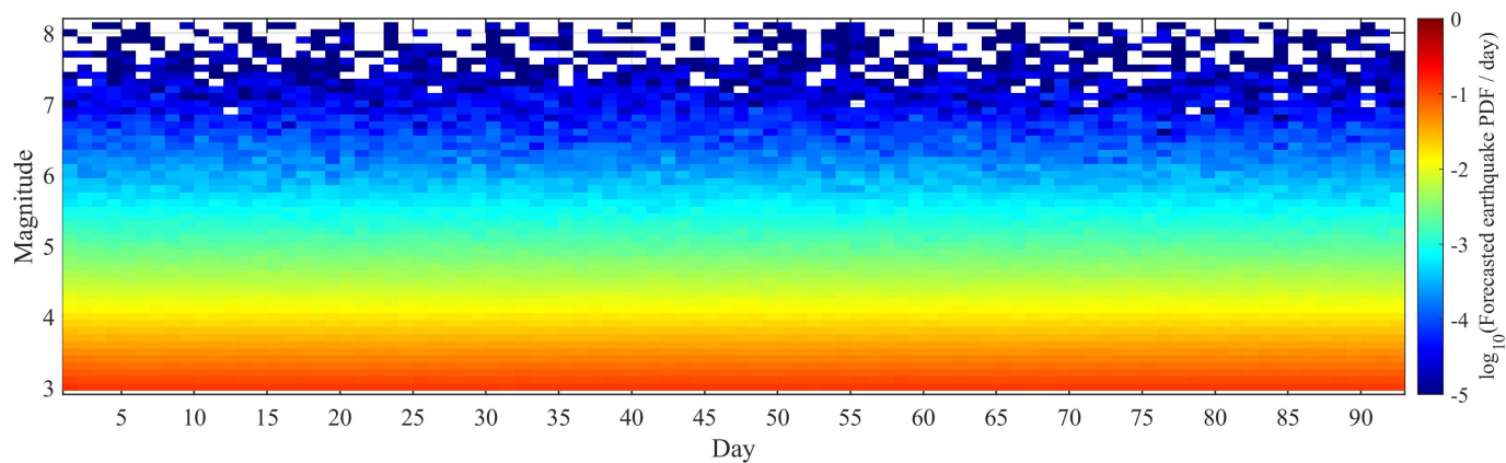
图 3. 未来一个季度中国地震科学实验场内预测地震每日的概率密度分布 (PDF)。
