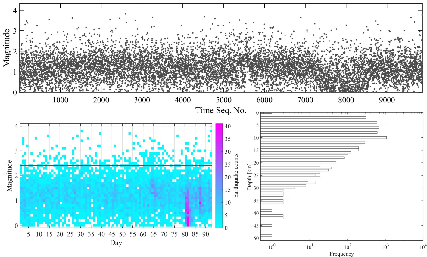
图 4. 过去一个季度中国地震科学实验场地震活动性的（上）震级-时间序号图；（左下）每 0.1 个震级区间的每日地震数量；（右下）深度-频次分布。震级-时间序号图中的震级被添加了 [-0.05, 0.05] 均匀分布的随机误差。左下图中的红色直线为过去一个季度的目录最小完整性震级 ( M_c )。
