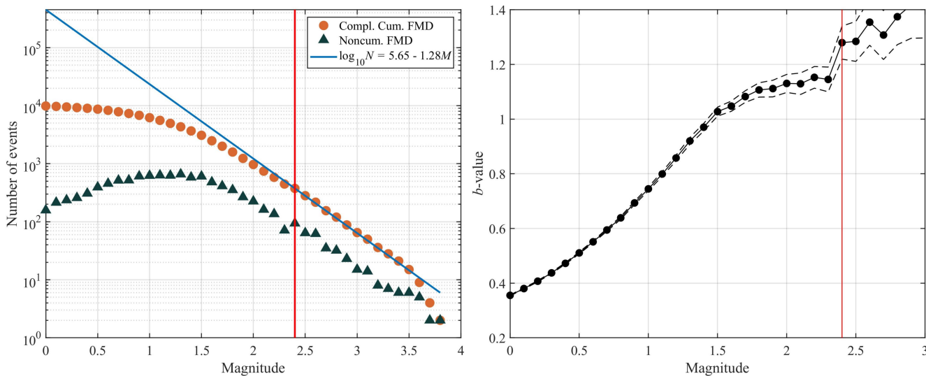
图 5. 过去一个季度中国地震科学实验场地震活动性的（左）互补累积和密度震级-频次分布以及大于过去一个季度的目录最小完整性震级 M_c （红竖线）地震的古登堡-里克特（GR）关系拟合结果；（右） b 值随目录截止震级 M_{\infty} 变化的曲线，其中细虚线表示 \pm 1\sigma 的标准差。
