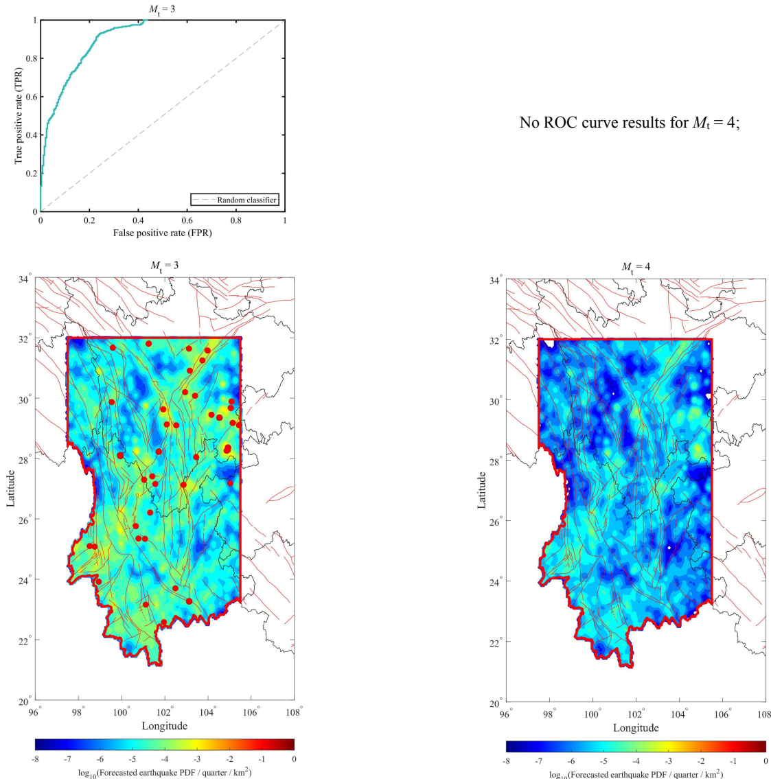
图 7. 过去一个季度中国地震科学实验场内观测地震活动 (红色实心圆) 的空间分布及其受试者操作特征 (ROC) 曲线 (正上方插图)。下图背景为上个季度预测报告发布的预测地震 ( M \geq M_t ) 每平方公里 (km 2 ) 概率密度分布 (PDF)。
