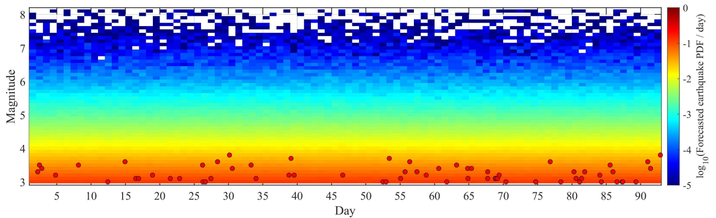
图 8. 过去一个季度中国地震科学实验场内观测地震活动 (红色实心圆) 的震级时间分布, 背景为上个季度预测报告发布的预测地震每日概率密度分布 (PDF)。
