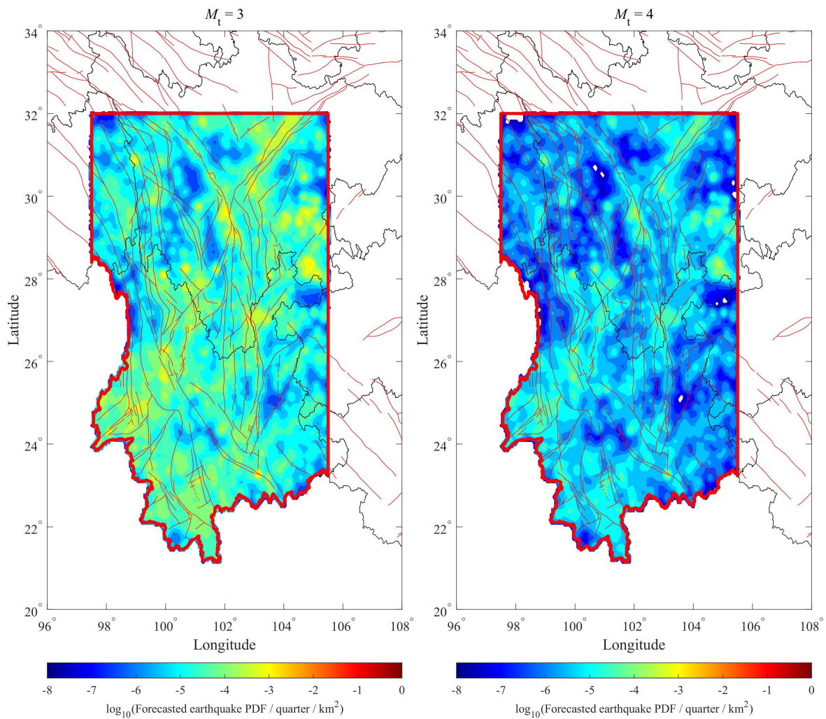
图 2. 未来一个季度中国地震科学实验场内预测地震 ( M \geq M_t ) 每平方公里 ( \text{km}^2 ) 的概率密度分布 (PDF)。
