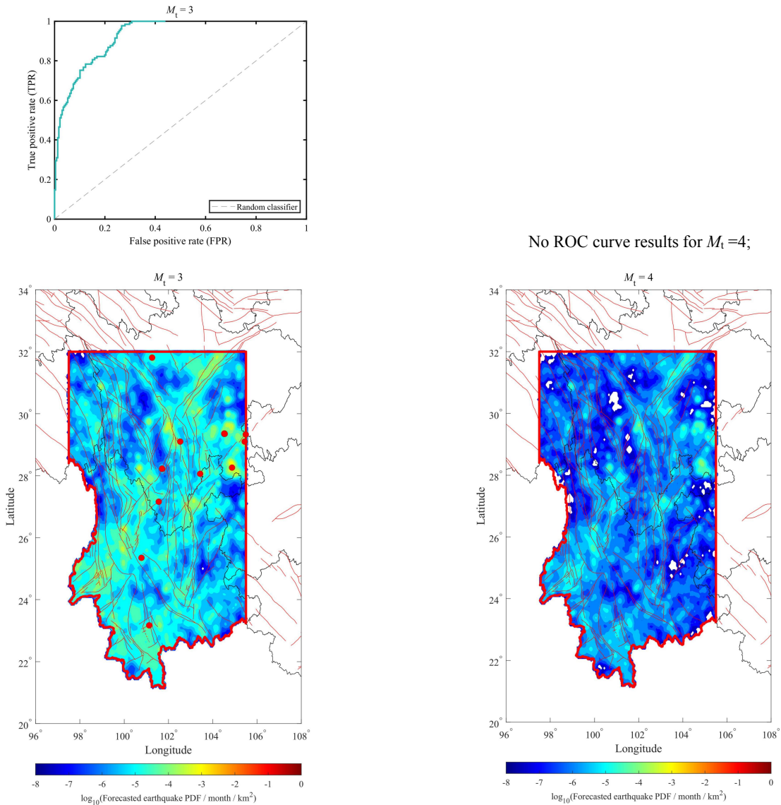
图 7. 过去一个月中国地震科学实验场内观测地震活动 (红色实心圆) 的空间分布及其受试者操作特征 (ROC) 曲线 (正上方插图)。下图背景为上个月度预测报告发布的预测地震 ( M \geq M_t ) 每平方公里 ( \text{km}^2 ) 概率密度分布 (PDF)。
