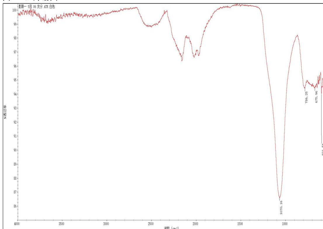
图 1 红外谱图
