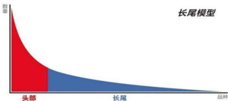
图 4-1 长尾模型
