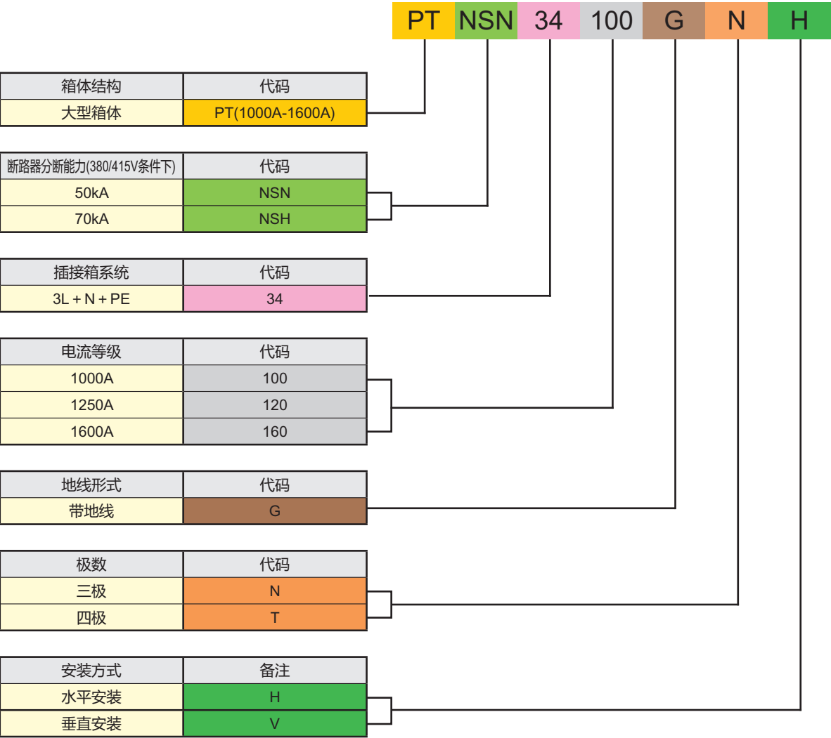
施耐德电气Compact NS断路器插接箱 (1000A-1600A)
