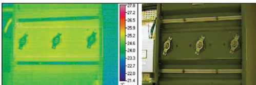
不同电流等级母线满载运行时的温度
