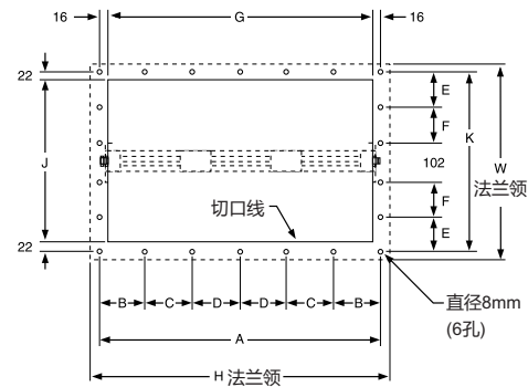
法兰领切口线和钻孔样板
