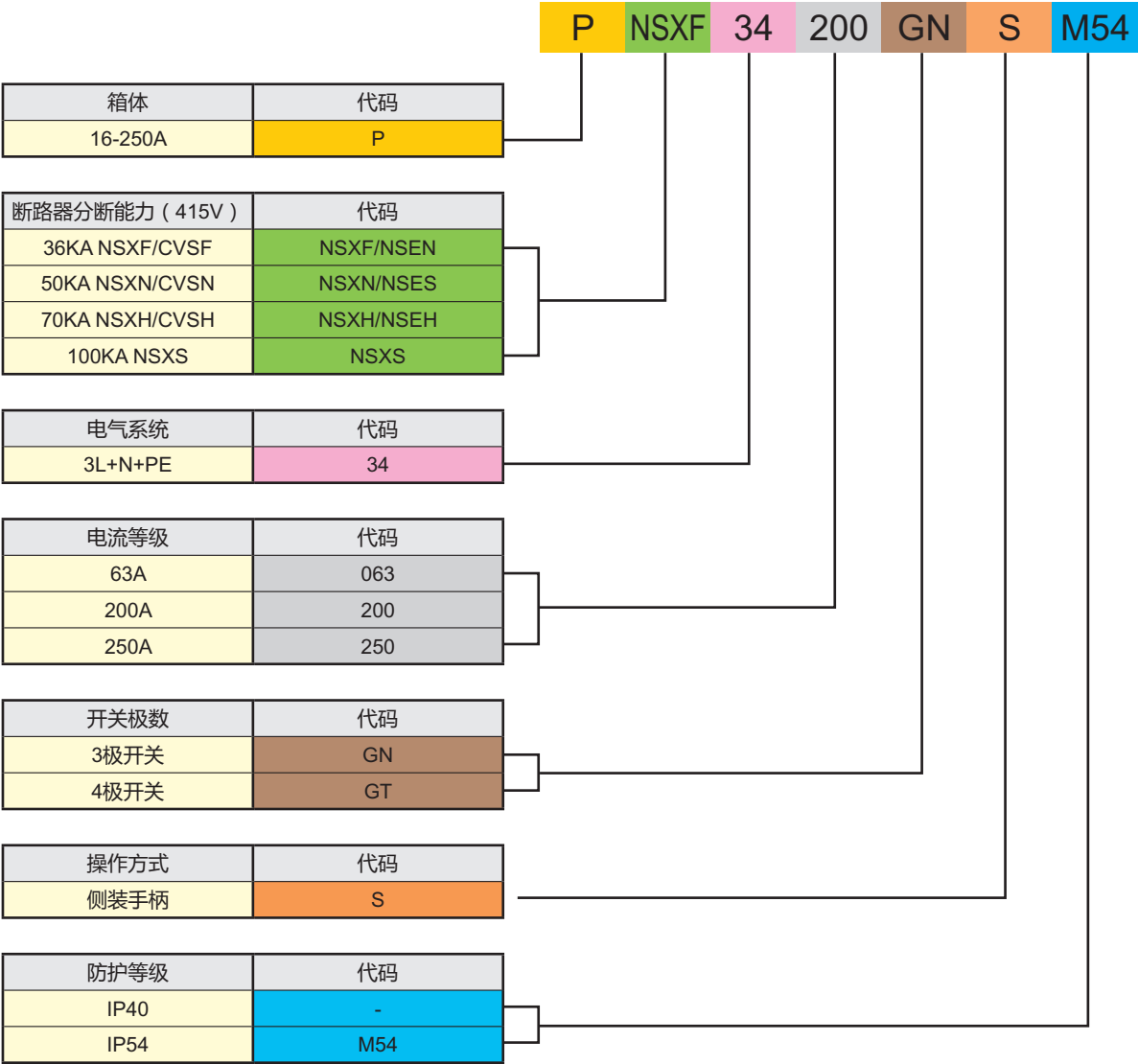
施耐德电气插接箱侧操箱（16A-250A）
