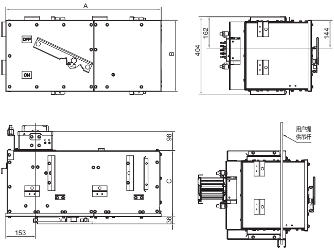
图6 1000-1600A插接箱
