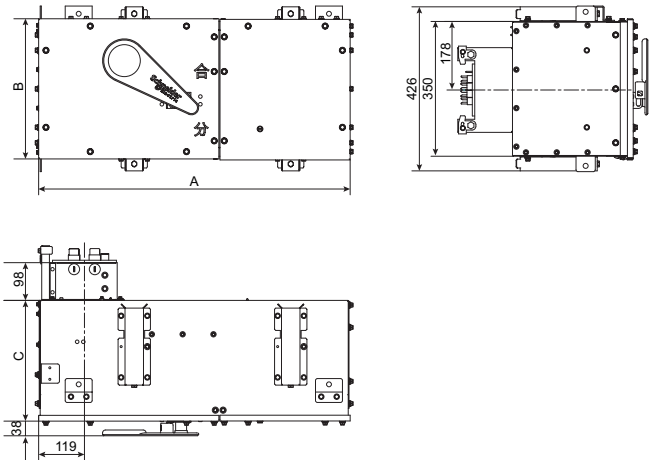
图5 800A插接箱
