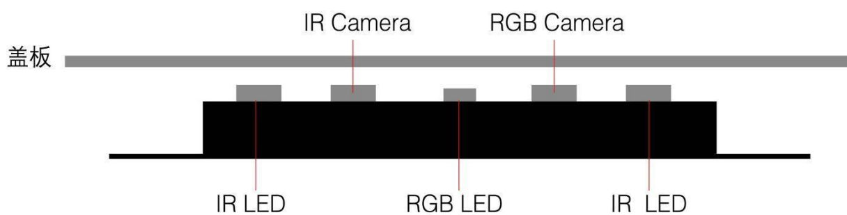
盖板与摄像头 AI 视觉算法模组安装示意图
