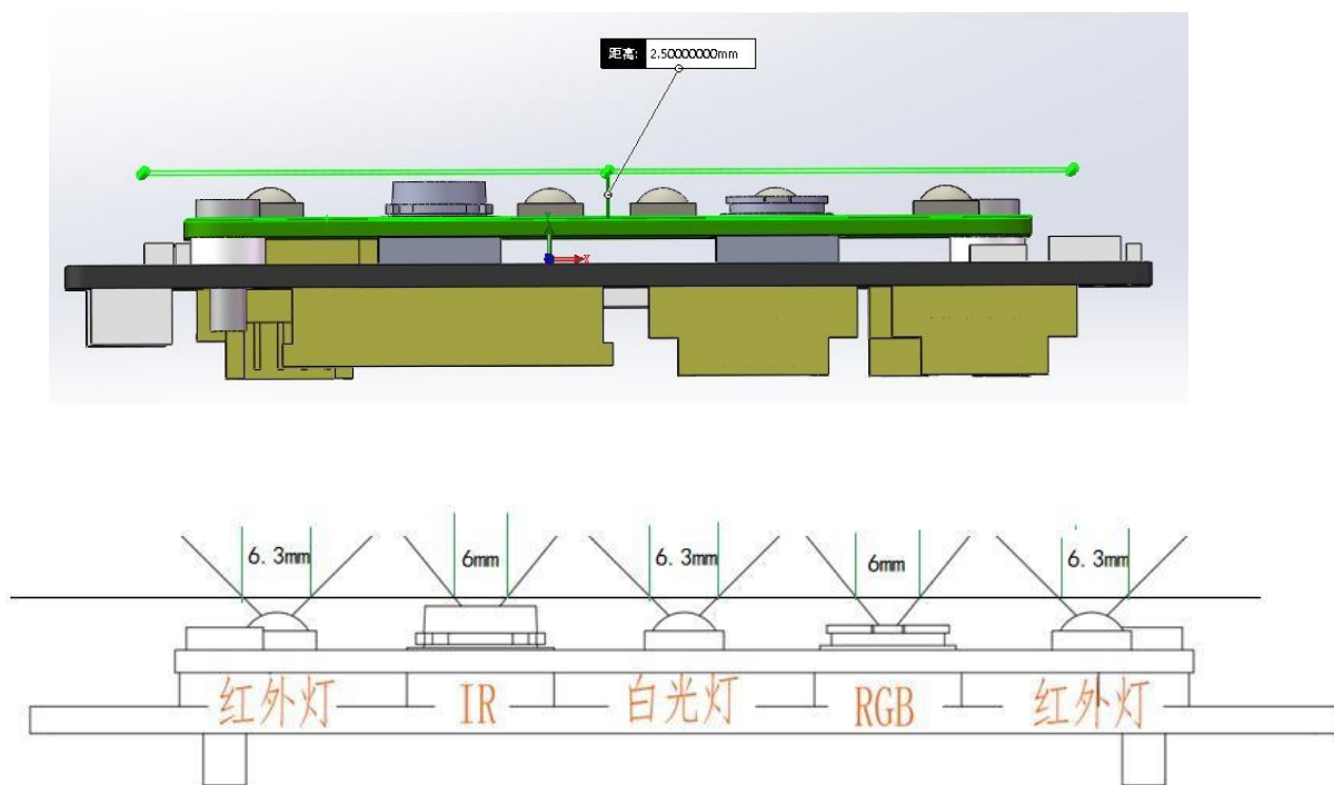
盖板开孔示意图
