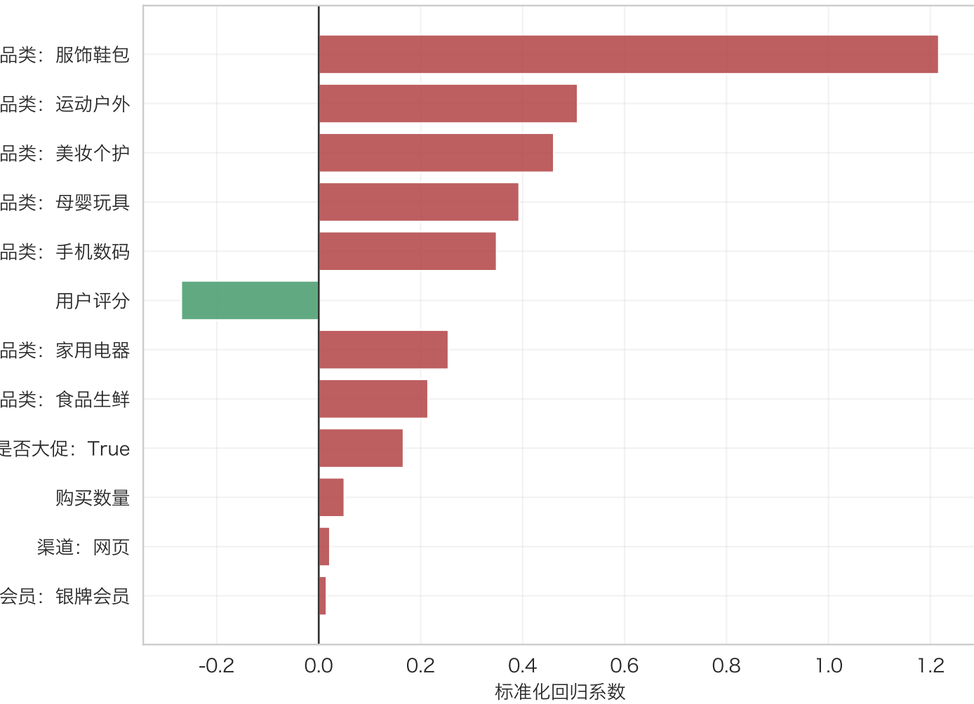
退货预测模型：特征影响方向 (红色提高退货概率，绿色降低)
