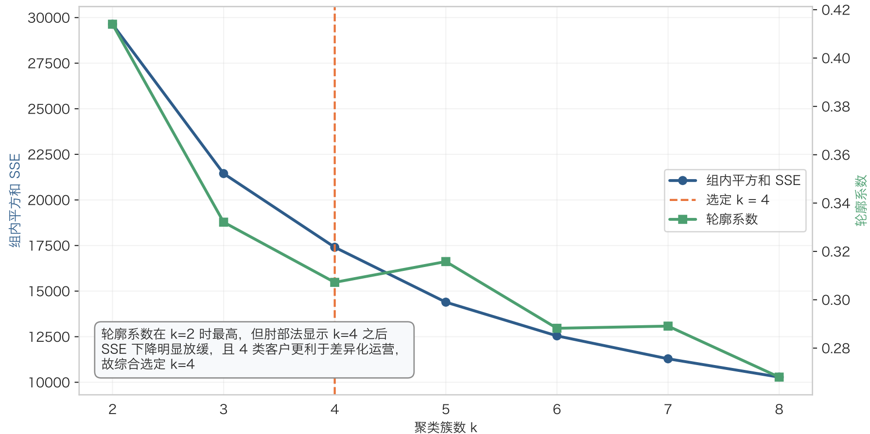
客户分群簇数选择：肘部法与轮廓系数
