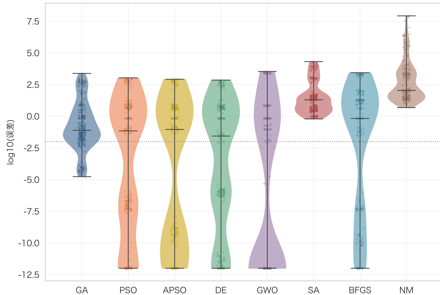
10 维：全部函数合并后的误差分布
