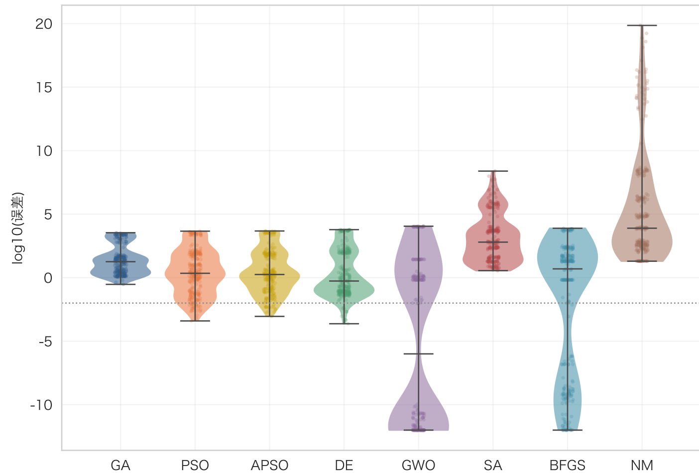
30 维：全部函数合并后的误差分布
