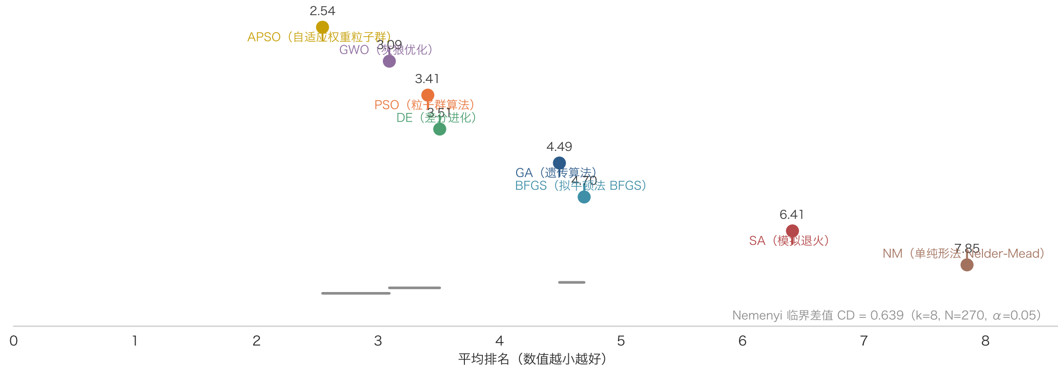
10 维下的算法排序与 Nemenyi 临界差异图
