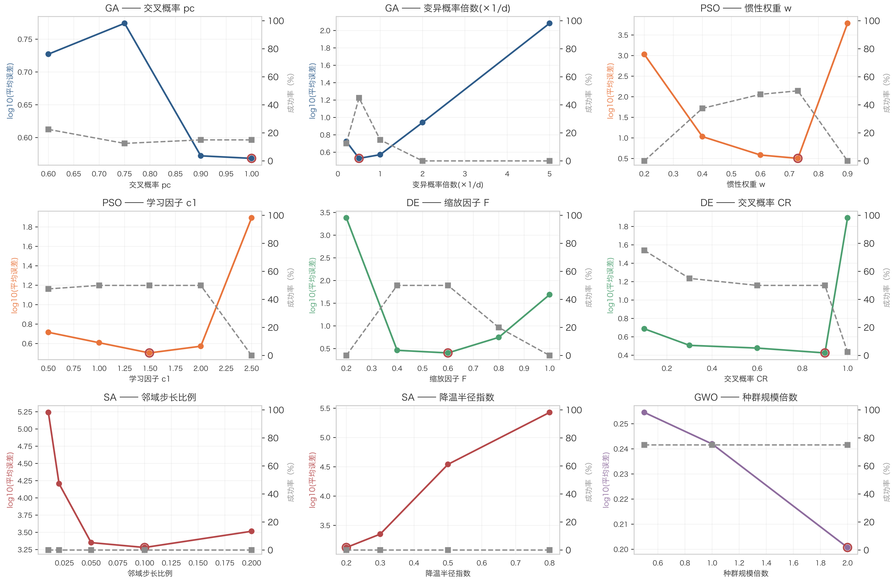
参数敏感性分析 (10 维, 4 个代表性函数 x 10 次重复; 红圈标记该参数的最优取值)
