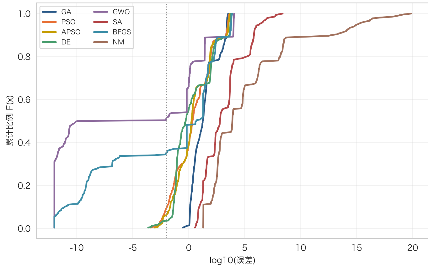
30 维: 全部 (函数 x 运行) 样本的误差 ECDF
