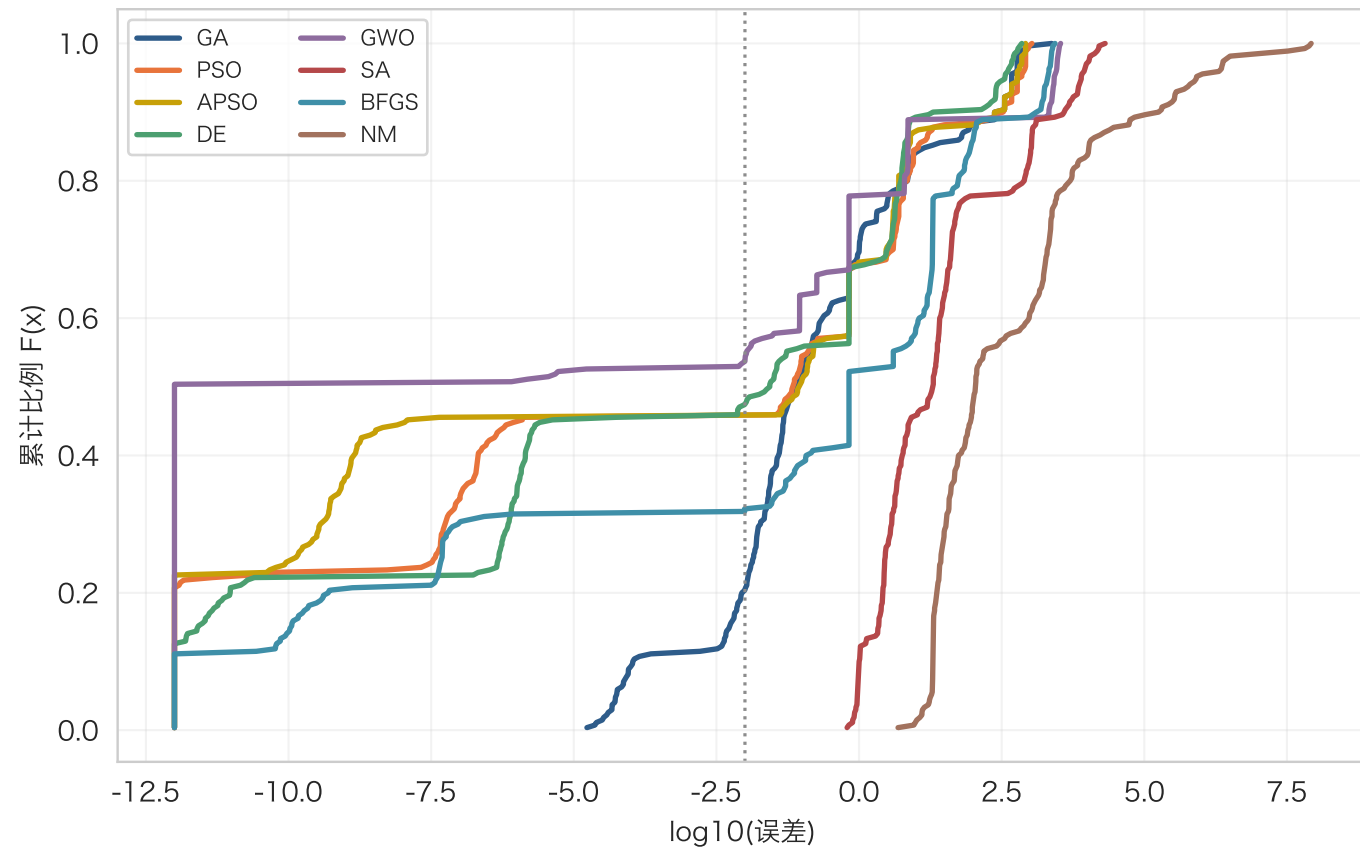
10 维: 全部 (函数 x 运行) 样本的误差 ECDF
