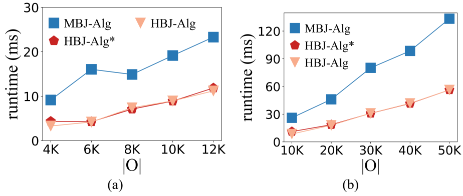
图 6-7 不同 |O| 下的构建时间影响 (a):Geolife 数据集下的实验; (b):Porto 数据集下的实验
