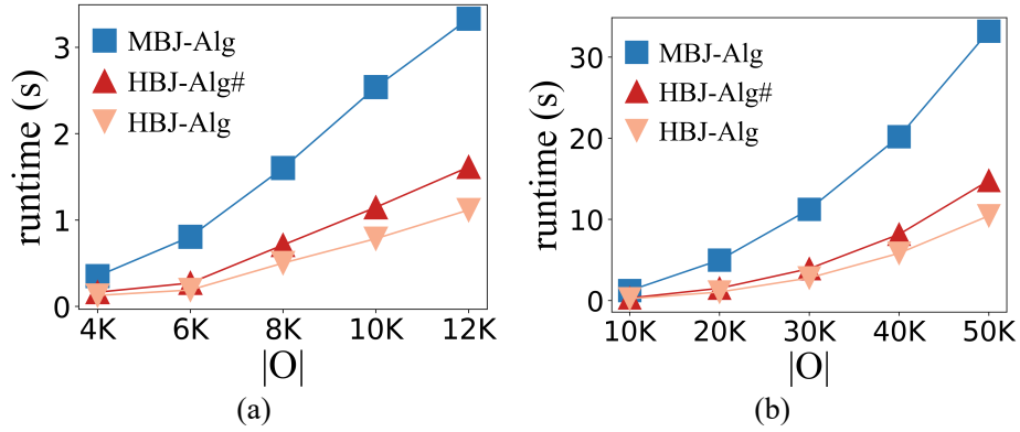
图 6-8 不同 |O| 下的查询时间影响 (a):Geolife 数据集下的实验; (b):Porto 数据集下的实验
