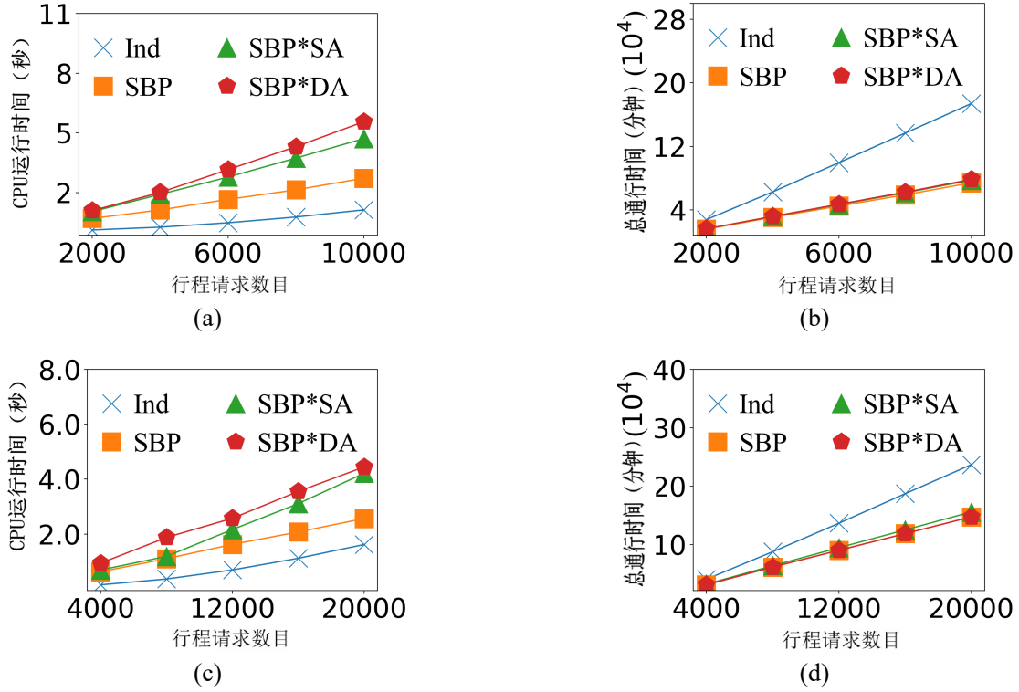
图 3-2 行程请求数目对算法运行时间和全局通行时间的影响。?? NY 路网下的算法运行时间；?? NY 路网下的总通行时间；?? TG 路网下的算法运行时间；?? TG 路网下的总通行时间
