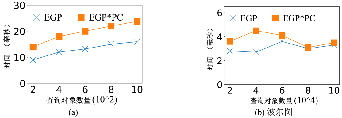
图 5-7 预检查策略的评估。?? 北京数据集；?? 波尔图数据集
