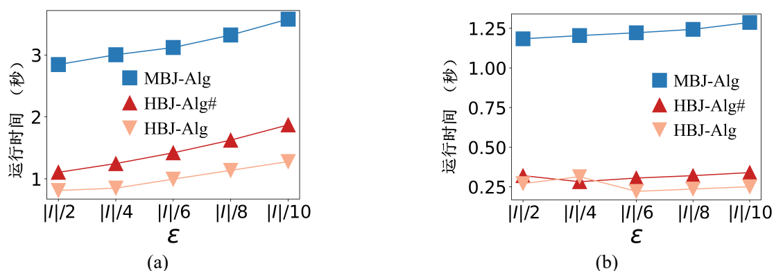
图 6-11 放宽参数对运行时间的影响。??:Geolife; ??: 波尔图
