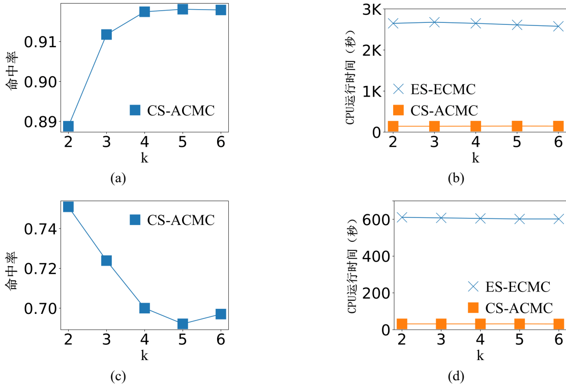
图 4-4 联合移动时长阈值的影响。?? 北京数据集上的命中率 ?? 北京数据集上的运行时间 ?? 波尔图数据集上的命中率 ?? 波尔图数据集上的运行时间
