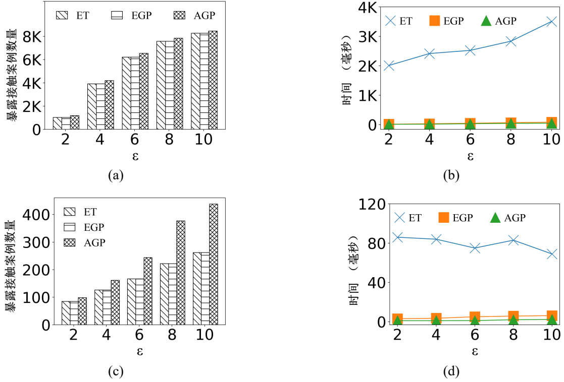
图 5-4 距离阈值的影响。?? 北京数据集上暴露接触案例数量；?? 北京数据集上算法运行时间；?? 波尔图数据集上暴露接触案例数量；?? 波尔图数据集上算法运行时间
