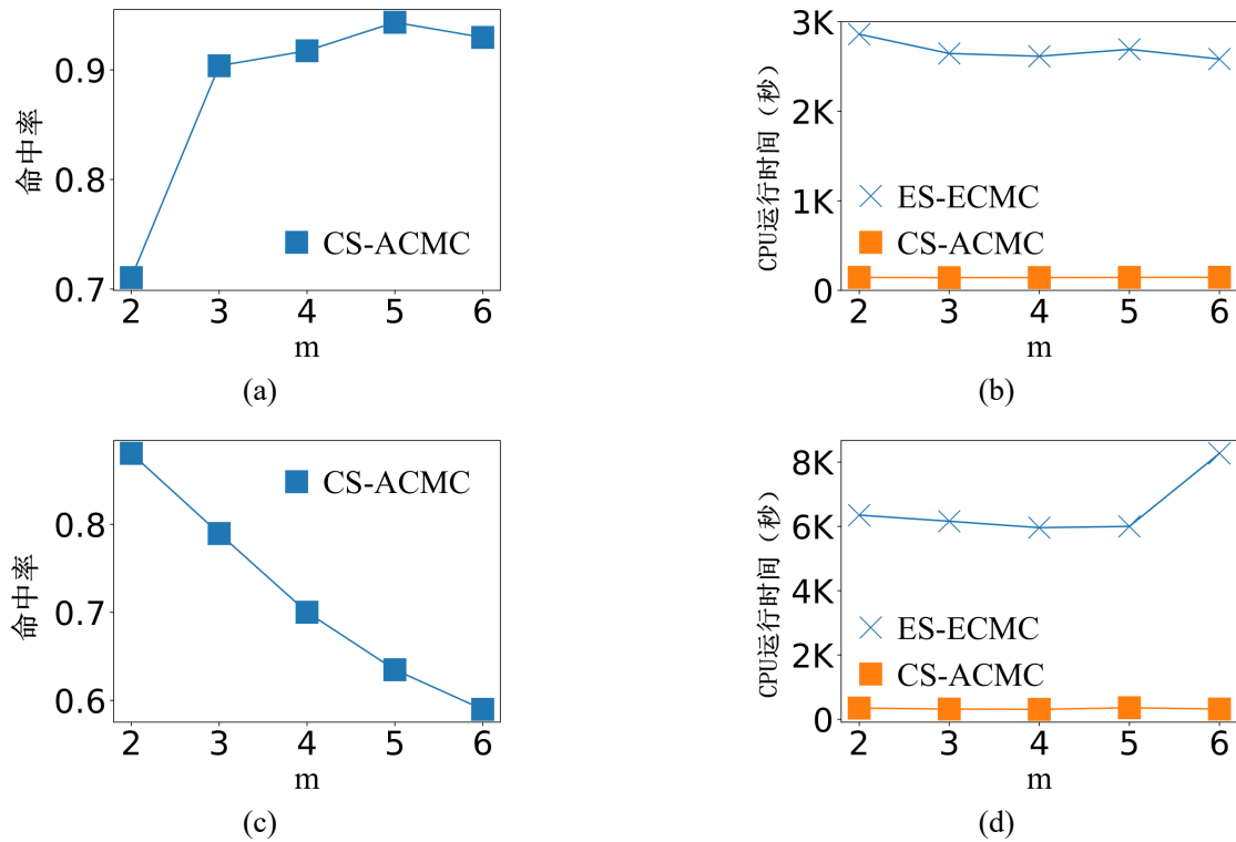
图 4-5 伴随群体规模阈值的影响。?? 北京数据集上的命中率 ?? 北京数据集上的运行时间 ?? 波尔图数据集上的命中率 ?? 波尔图数据集上的运行时间
