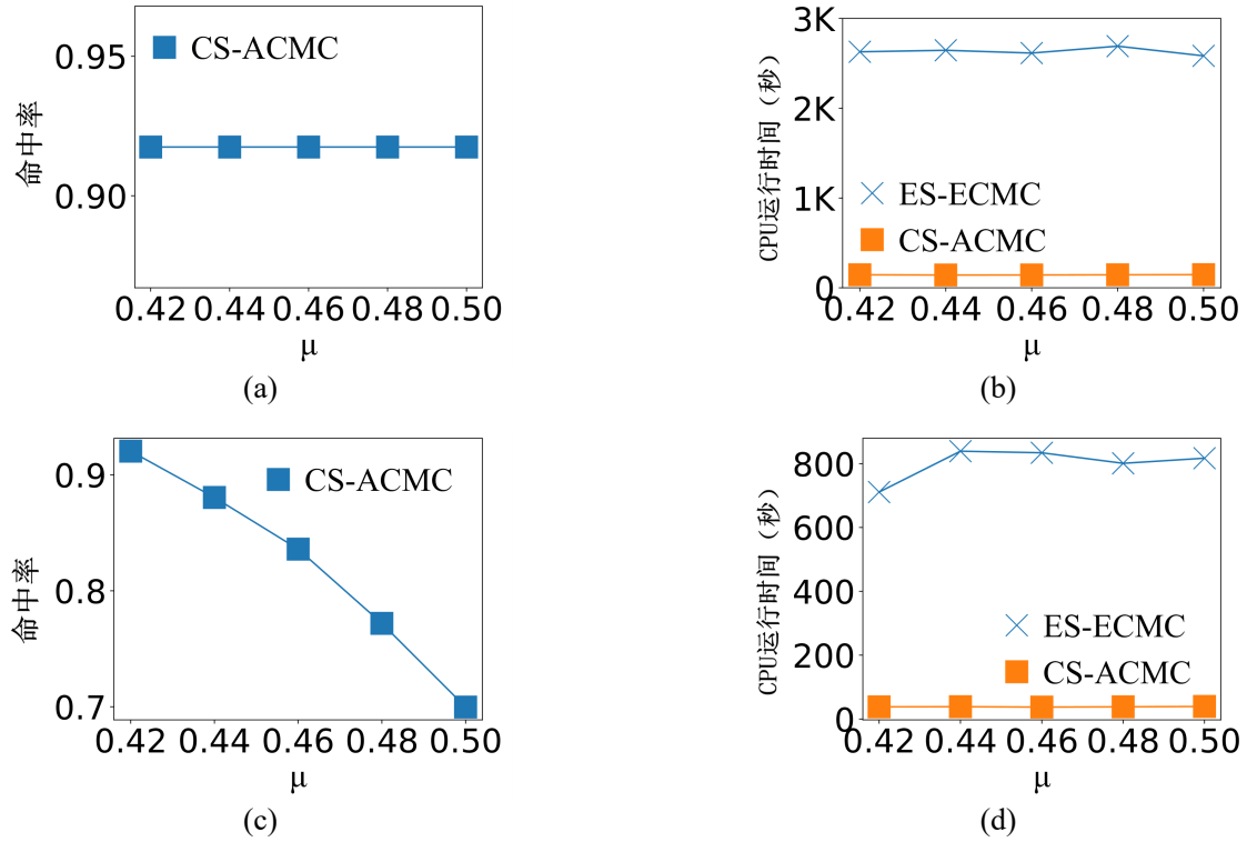
图 4-6 SCAN 聚类结构相似度参数的影响。?? 北京数据集上的命中率 ??
