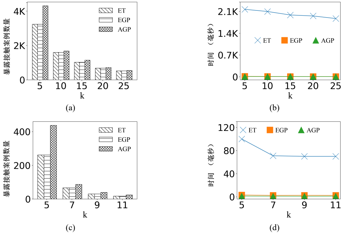
图 5-5 接触持续时长阈值的影响。?? 北京数据集上暴露接触案例数量；?? 北京数据集上算法运行时间；?? 波尔图数据集上暴露接触案例数量；?? 波尔图数据集上算法运行时间
