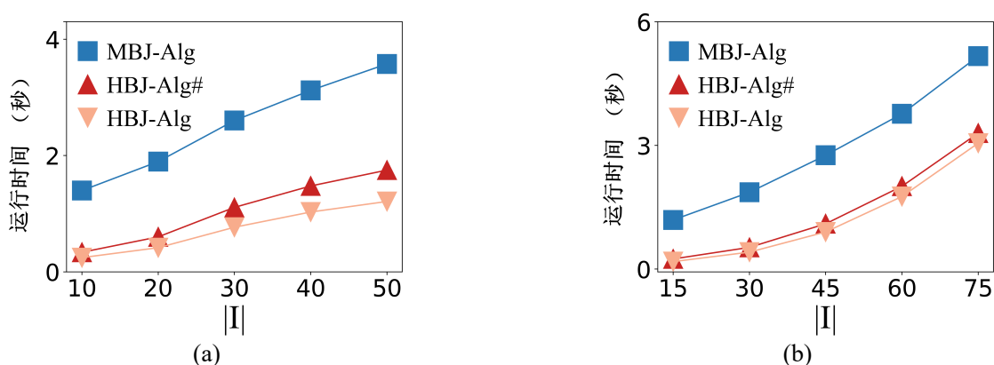
图 6-10 时间段对运行时间的影响。??:Geolife; ??: 波尔图
