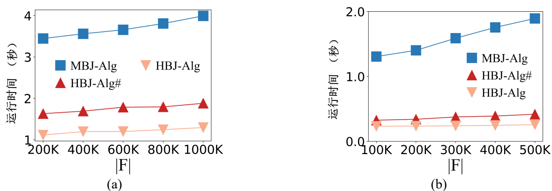
图 6-9 兴趣点数量对运行时间的影响。??:Geolife; ??: 波尔图
