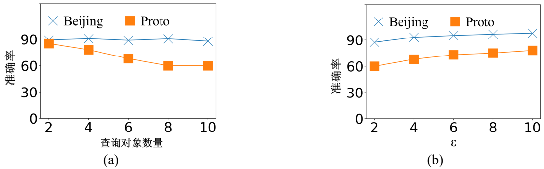
图 5-6 近似算法的评估。?? 变化查询对象数目；?? 变化接触阈值
