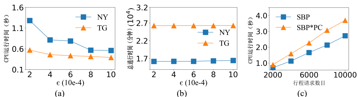
图 3-6 提升参数和预检查策略的影响。?? 运行时间；?? 通行时间；?? 预检查策略的影响评估
