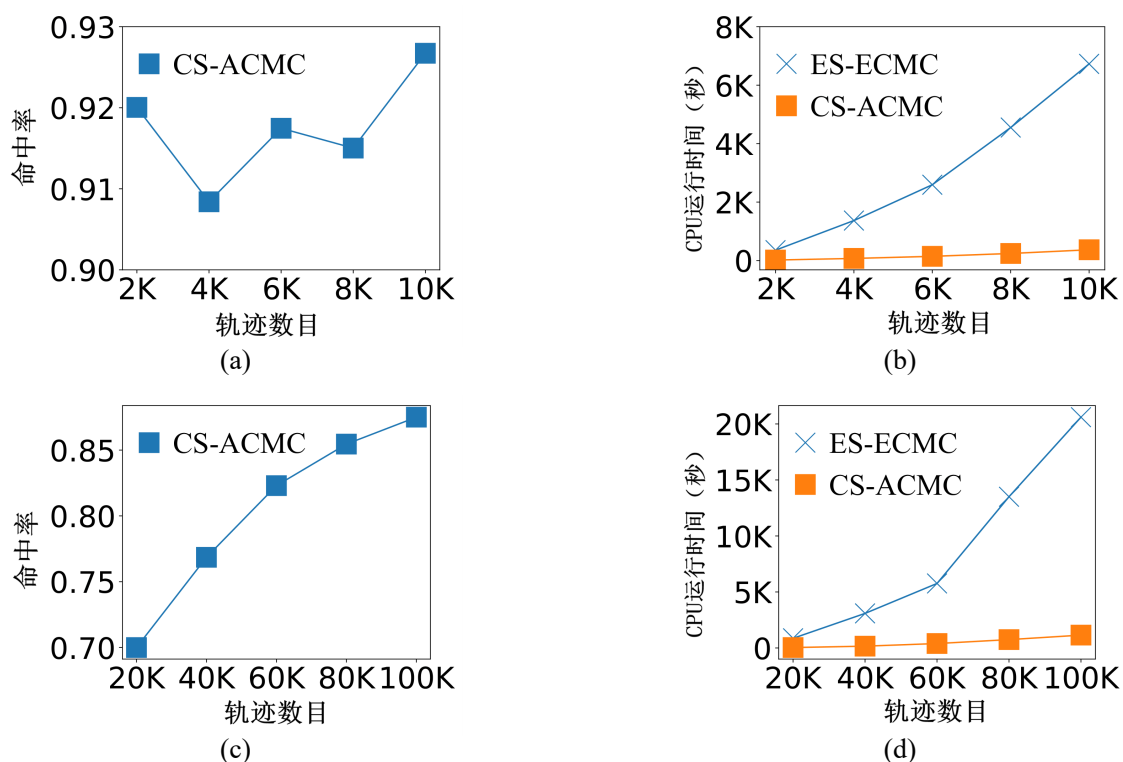
图 4-3 轨迹数目的影响。?? 北京数据集上的命中率 ?? 北京数据集上的运行时间 ?? 波尔图数据集上的命中率 ?? 波尔图数据集上的运行时间
