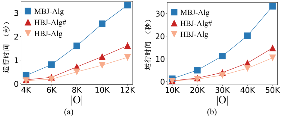
图 6-8 不同移动对象数目下的查询时间。?? : Geolife; ?? : 波尔图
