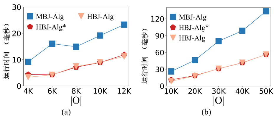
图 6-7 不同移动对象数目下的构建时间。??: Geolife; ??: 波尔图
