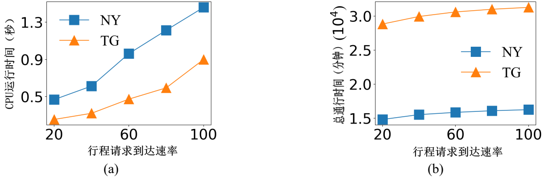
图 3-3 行程请求到达速率的影响。?? 对算法运行时间的影响；?? 对总通行时间的影响
