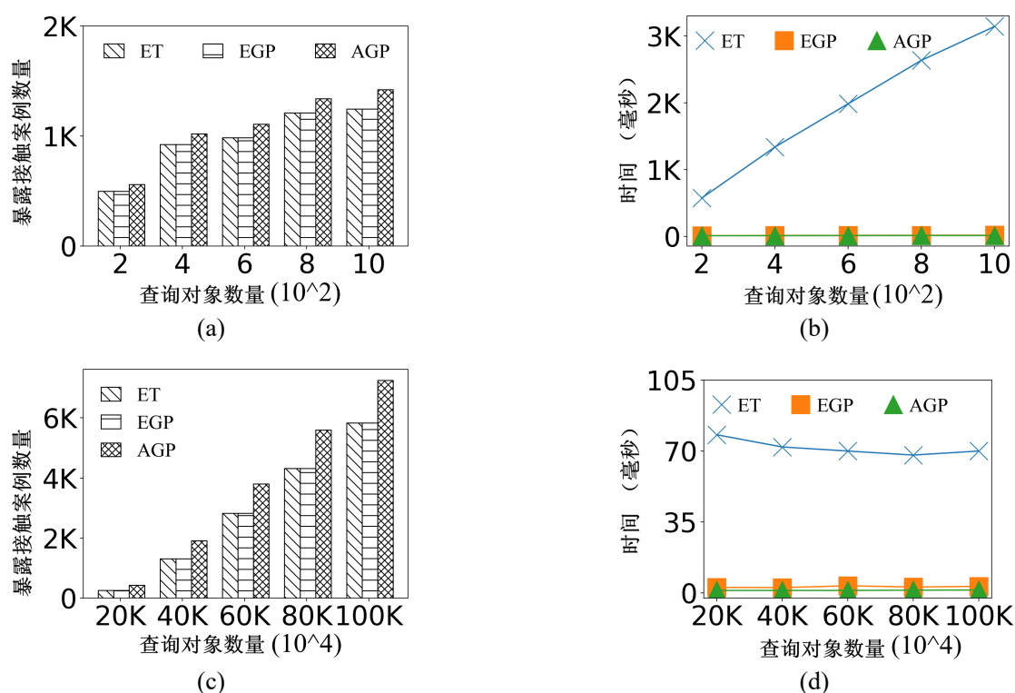
图 5-3 查询对象数量的影响。?? 北京数据集上暴露接触案例数量；?? 北京数据集上算法运行时间；?? 波尔图数据集上暴露接触案例数量；?? 波尔图数据集上算法运行时间
