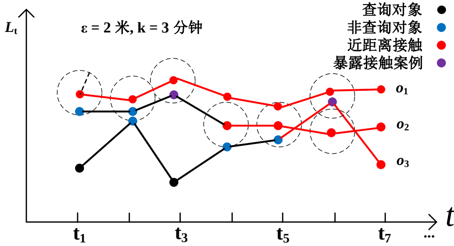
图 5-1 持续暴露接触搜索问题
