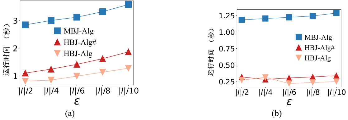
图 6-11 参数 \epsilon 的影响 (a):Geolife 数据集下的实验; (b): 波尔图数据集下的实验
