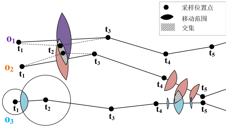
图 6-1 交集相似度连接问题示例
