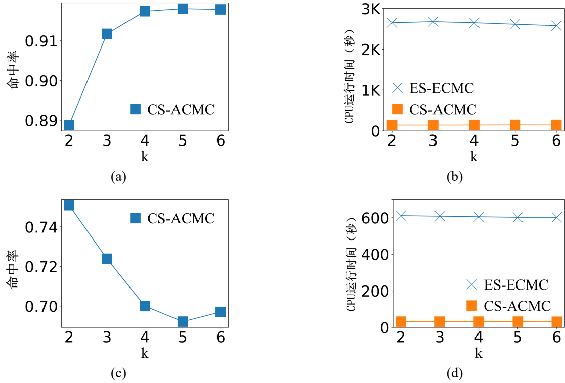
图 4-4 协同行为持续时间阈值的影响。(a) 北京数据集上的命中率 (b) 北京数据集上的运行时间 (c) 波尔图数据集上的命中率 (d) 波尔图数据集上的运行时间
