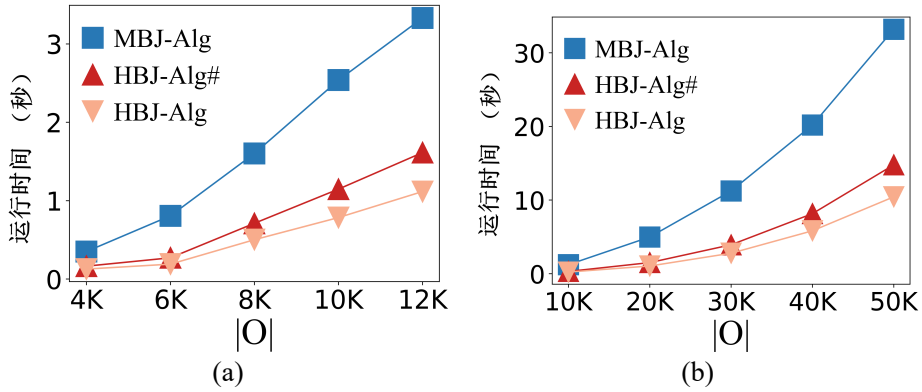
图 6-8 不同 |O| 下的查询时间影响 (a):Geolife 数据集下的实验; (b): 波尔图数据集下的实验
