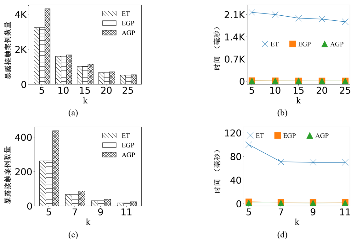
图 5-5 接触持续时长阈值 k 的影响。(a) 北京数据集上暴露接触案例数量； (b) 北京数据集上算法运行时间；(c) 波尔图数据集上暴露接触案例数量； (d) 波尔图数据集上算法运行时间
