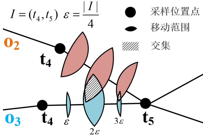
图 6-3 时间区间交集相似度的示意图
