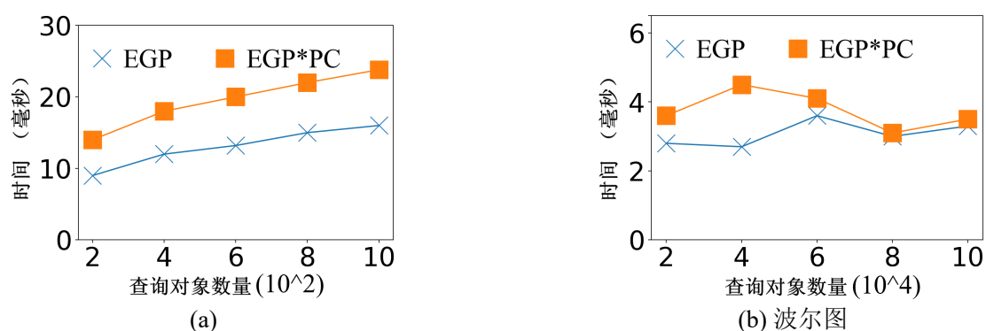
图 5-7 预检查策略的评估。(a) 北京数据集；(b) 波尔图数据集
