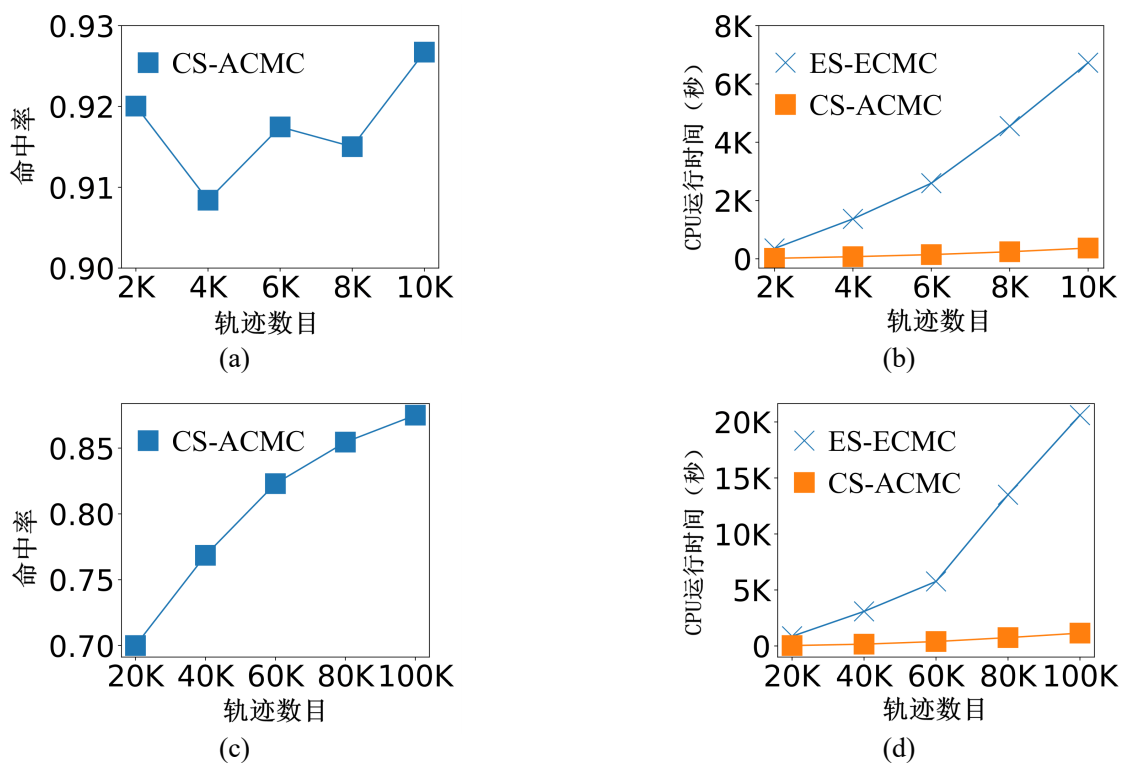
图 4-3 轨迹数量的影响。(a) 北京数据集上的命中率 (b) 北京数据集上的运行时间 (c) 波尔图数据集上的命中率 (d) 波尔图数据集上的运行时间
