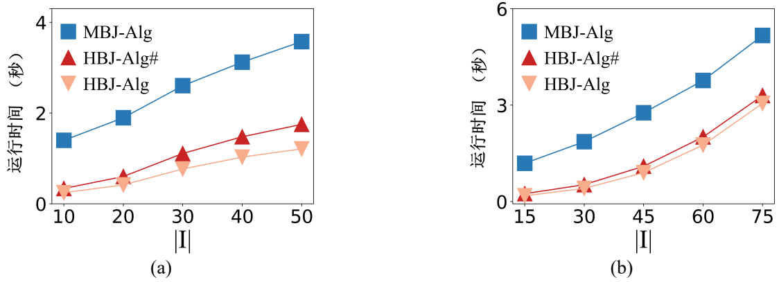
图 6-10 |I| 对运行时间的影响 (a):Geolife 数据集下的实验; (b): 波尔图数据集下的实验
