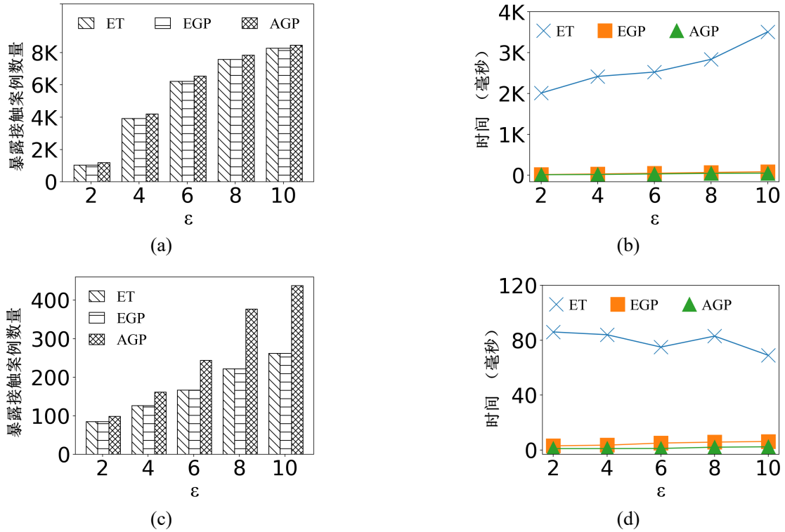
图 5-4 距离阈值 \epsilon 的影响。(a) 北京数据集上暴露接触案例数量；(b) 北京数据集上算法运行时间；(c) 波尔图数据集上暴露接触案例数量；(d) 波尔图数据集上算法运行时间
