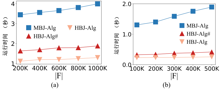
图 6-9 POI 数量对运行时间的影响 (a):Geolife 数据集下的实验; (b): 波尔图数据集下的实验
