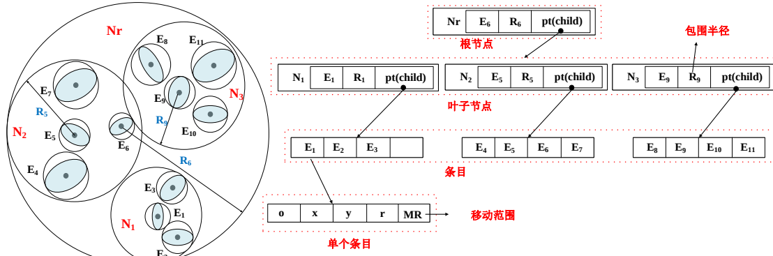
图 6-4 M* 树的结构
