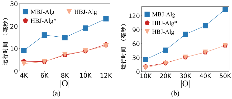
图 6-7 不同 |O| 下的构建时间影响 (a):Geolife 数据集下的实验; (b): 波尔图数据集下的实验
