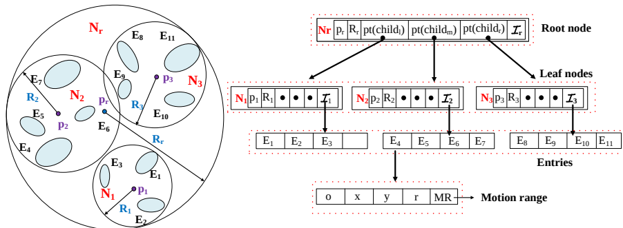
图 7-5 混合 Ball-tree 的示意图
