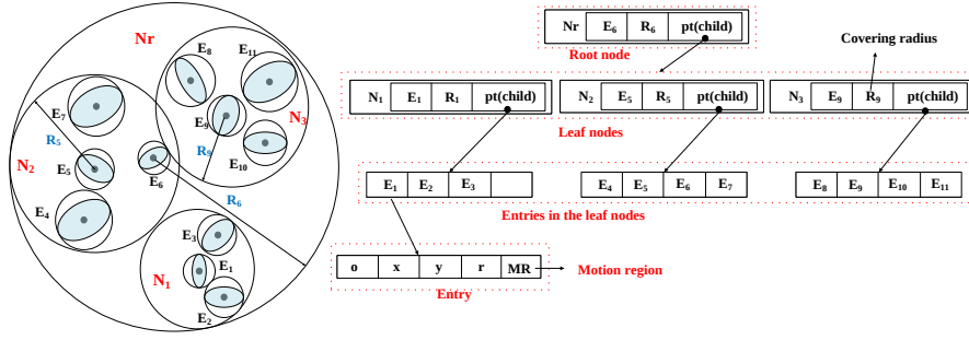
图 7-11 M*-树的结构
