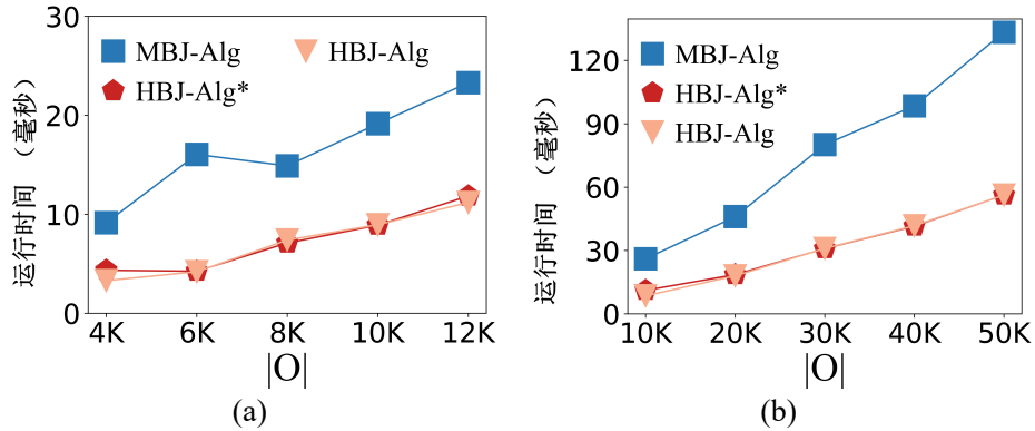
图 6-7 不同移动对象数目下的构建时间。(a): Geolife; (b): 波尔图
