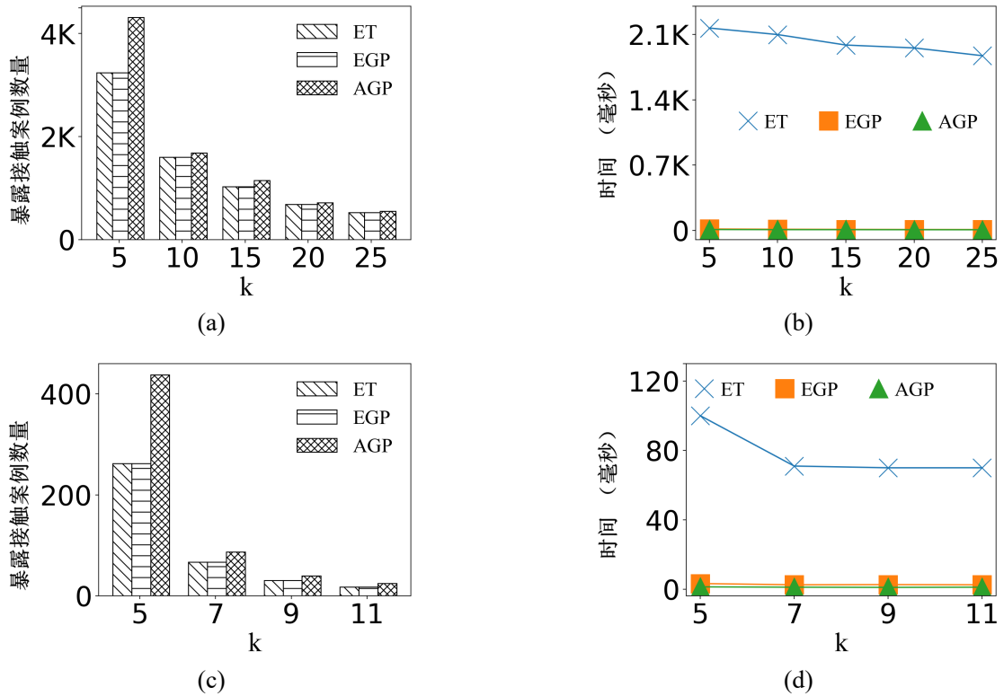
图 5-5 接触持续时长阈值的影响。(a) 北京数据集上暴露接触案例数量； (b) 北京数据集上算法运行时间；(c) 波尔图数据集上暴露接触案例数量； (d) 波尔图数据集上算法运行时间
