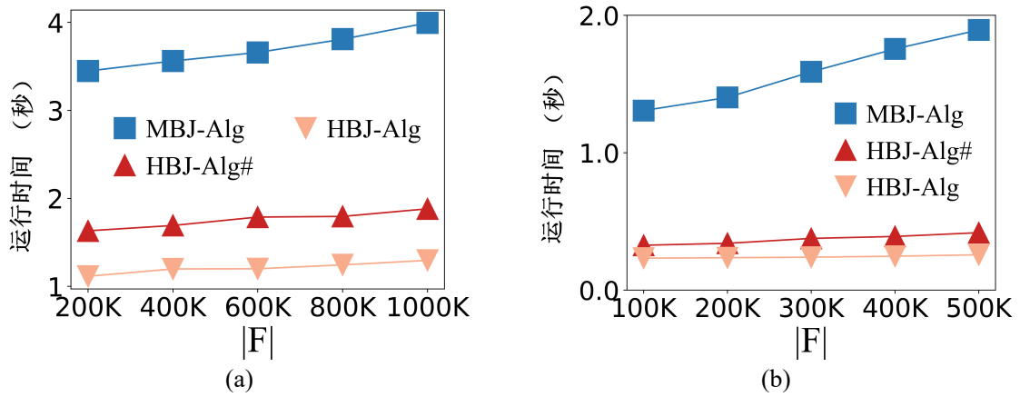
图 6-9 兴趣点数量对运行时间的影响。(a):Geolife; (b): 波尔图
