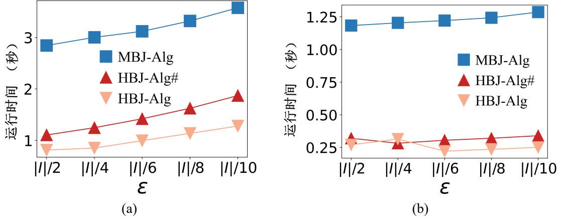
图 6-11 放宽参数对运行时间的影响。(a):Geolife; (b): 波尔图
