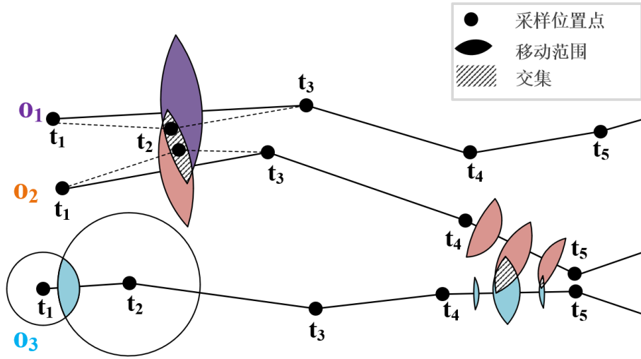
图 6-1 交集相似度连接示例
