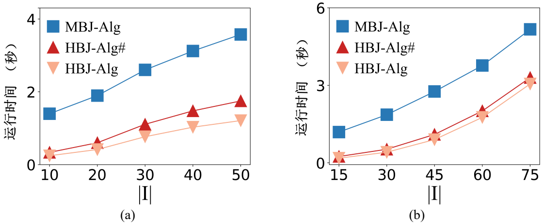
图 6-10 时间段对运行时间的影响。(a):Geolife; (b): 波尔图
