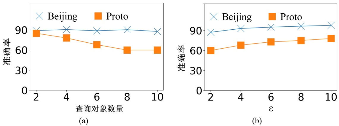
图 5-6 近似算法的评估。(a) 变化查询对象数目；(b) 变化接触阈值
