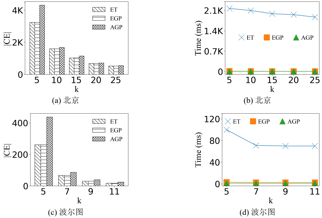
图 5-5 接触持续时长阈值 k 的影响
