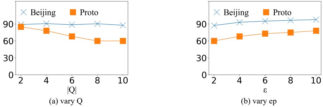
图 5-6 近似算法的评估
