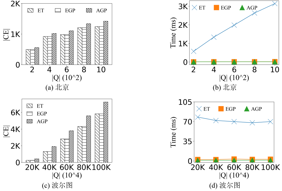
图 5-3 查询对象数量的影响
