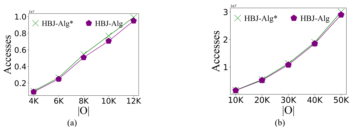
图 6-13 移动对象数量对节点访问次数的影响 (a):Geolife 数据集下的实验; (b):Porto 数据集下的实验
