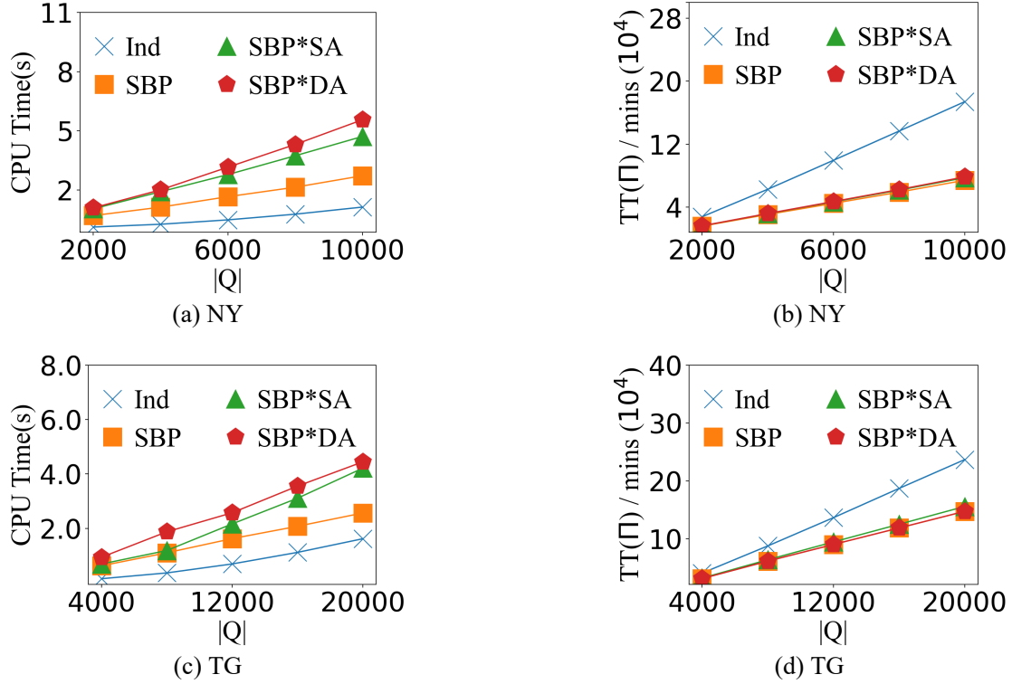
图 3-2 行程请求数目 |Q| 对算法运行时间和全局通行时间的影响
