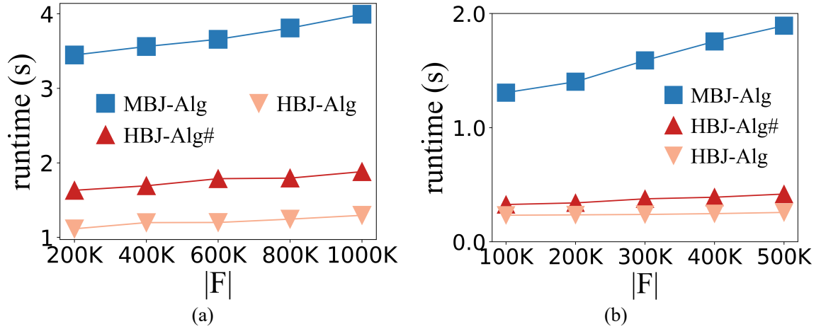
图 6-9 POI 数量对运行时间的影响 (a):Geolife 数据集下的实验; (b):Porto 数据集下的实验
