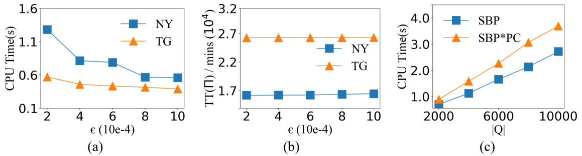
图 3-6 参数 \epsilon 和预检查策略的影响 (a) CPU 运行时间；(b) 通行时间；(c) 预检查策略的影响评估
