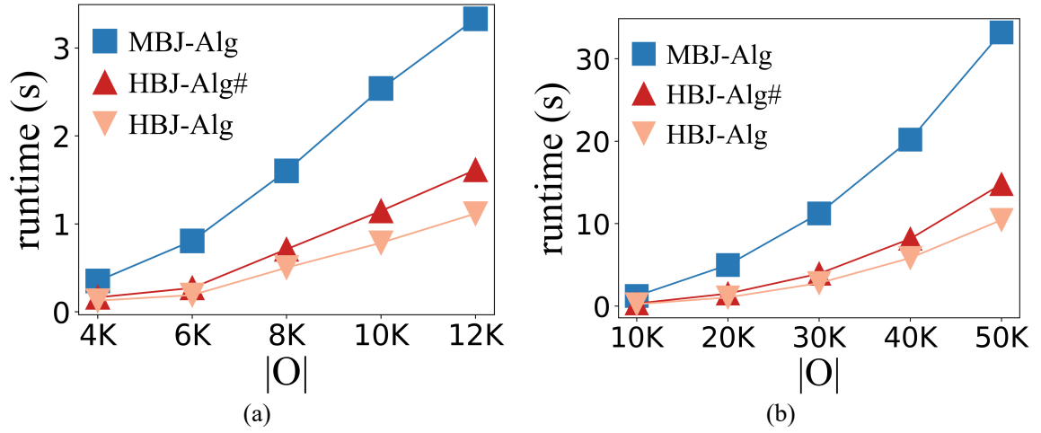
图 6-8 不同 |O| 下的查询时间影响 (a):Geolife 数据集下的实验; (b):Porto 数据集下的实验
