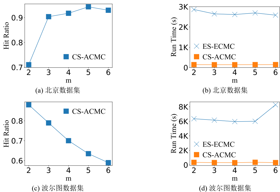
图 4-5 Effect of parameter m
