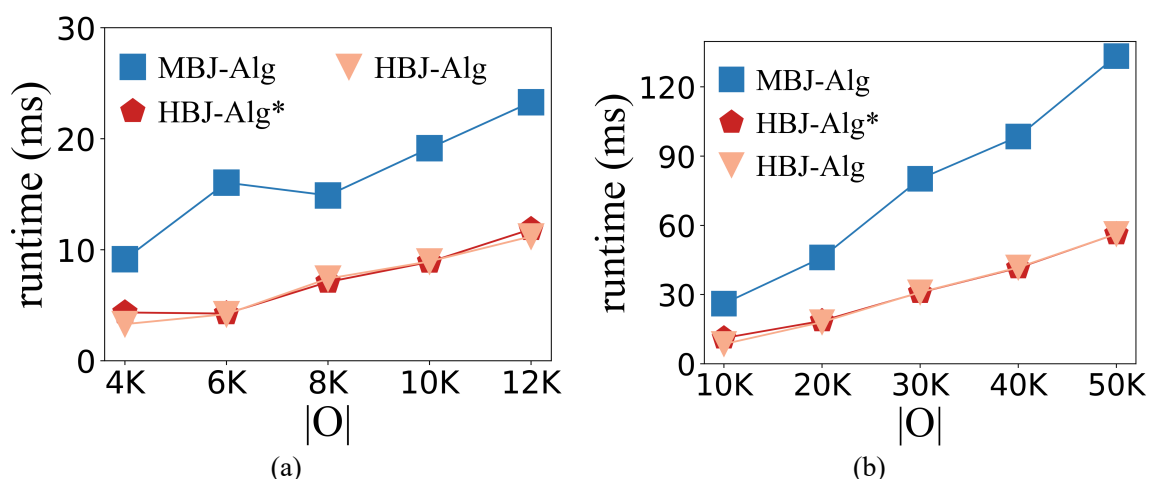
图 6-7 不同 |O| 下的构建时间影响 (a):Geolife 数据集下的实验; (b):Porto 数据集下的实验
