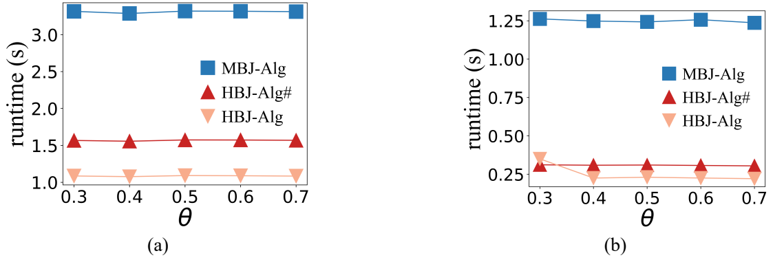
图 6-12 相似度阈值的影响 (a):Geolife 数据集下的实验; (b):Porto 数据集下的实验
