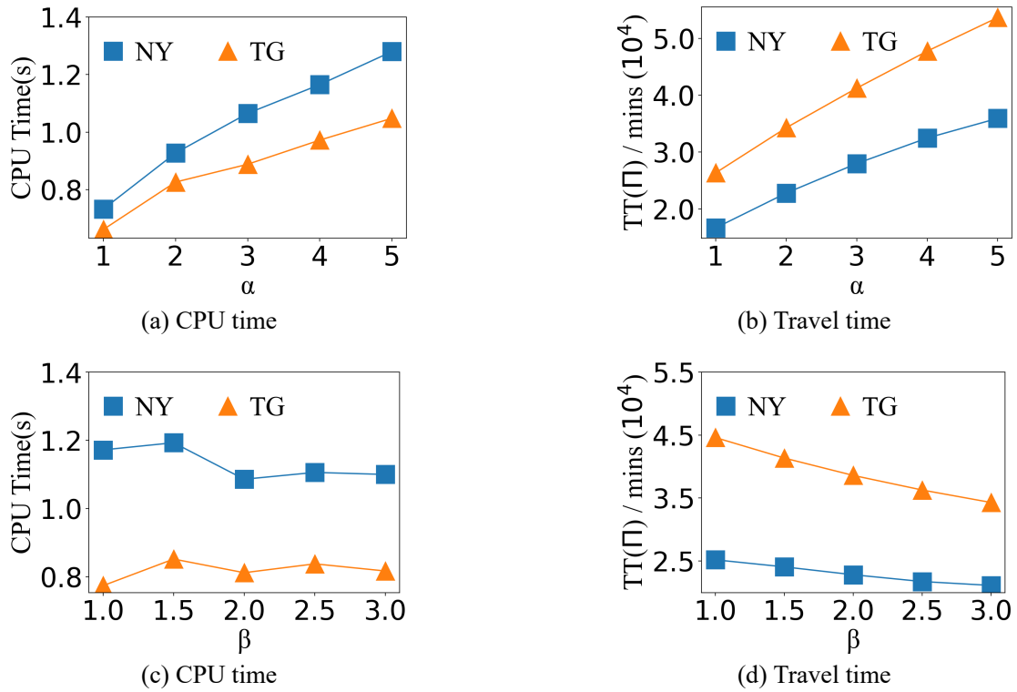
图 3-4 参数 \alpha & \beta 的影响
