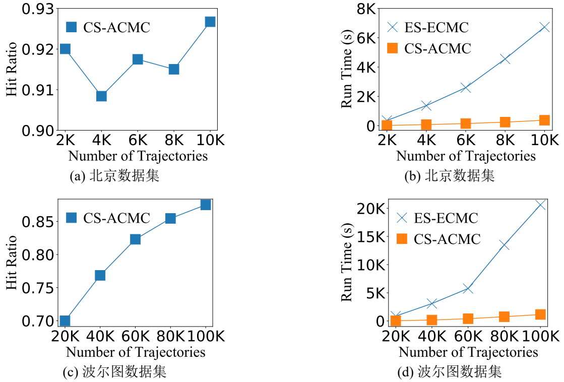
图 4-3 轨迹数量的影响
