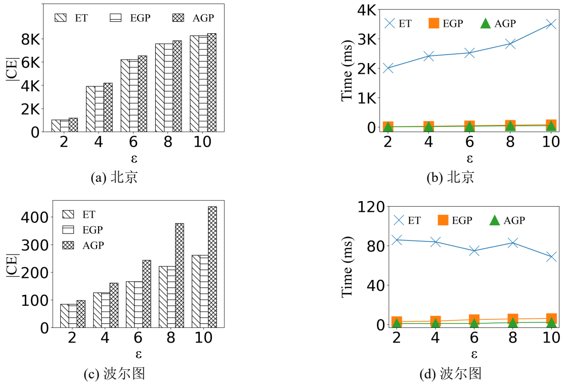
图 5-4 距离阈值 \epsilon 的影响
