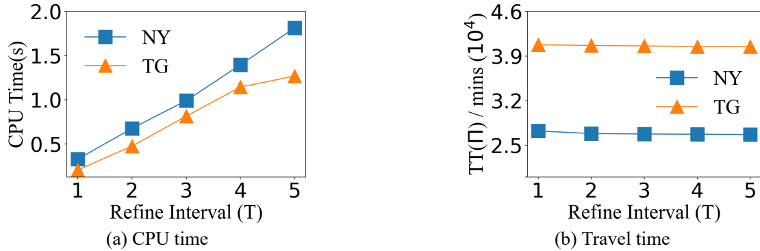
图 3-5 批优化时间间隔 T 的影响
