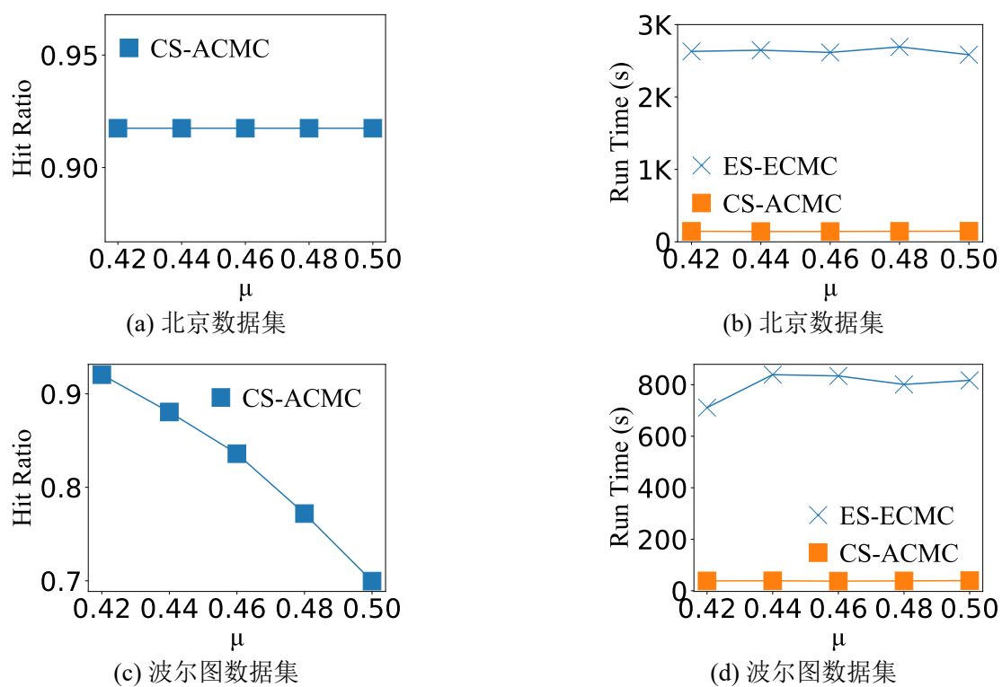
图 4-6 SCAN 聚类结构相似度参数的影响
