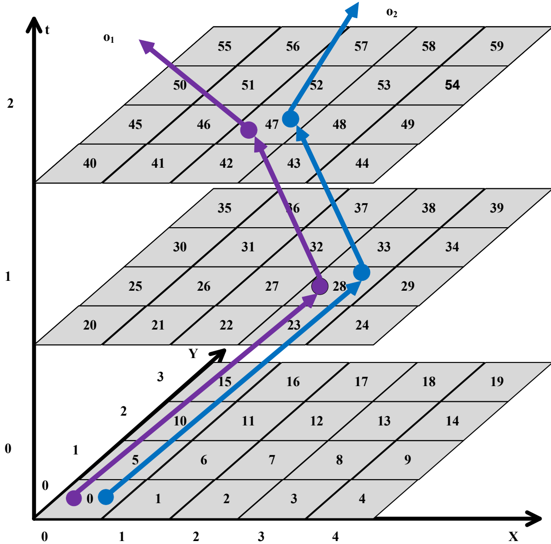
图 4-2 轨迹网格编号及网格编号序列示例
