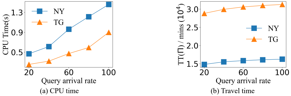
图 3-3 行程请求到达速率的影响
