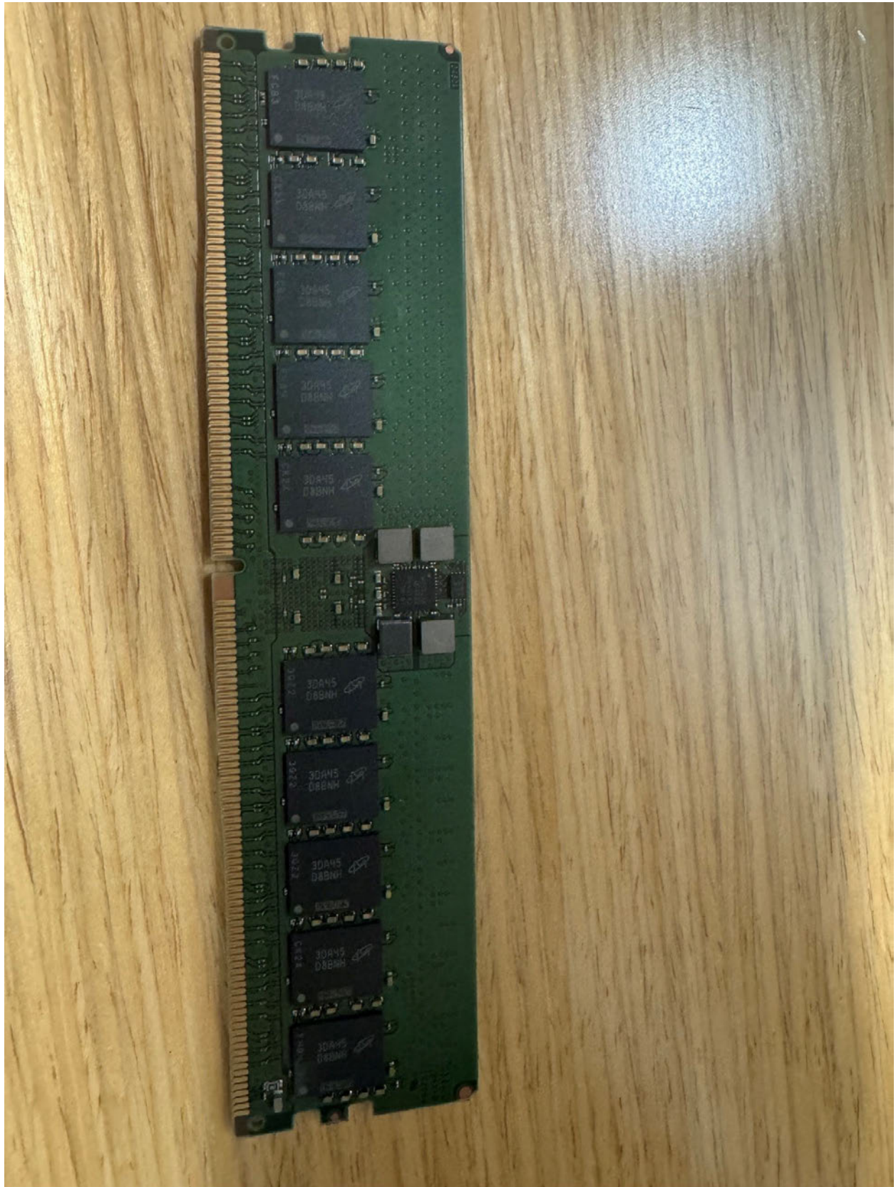
Lenovo_RDIMM_Jul26_4
