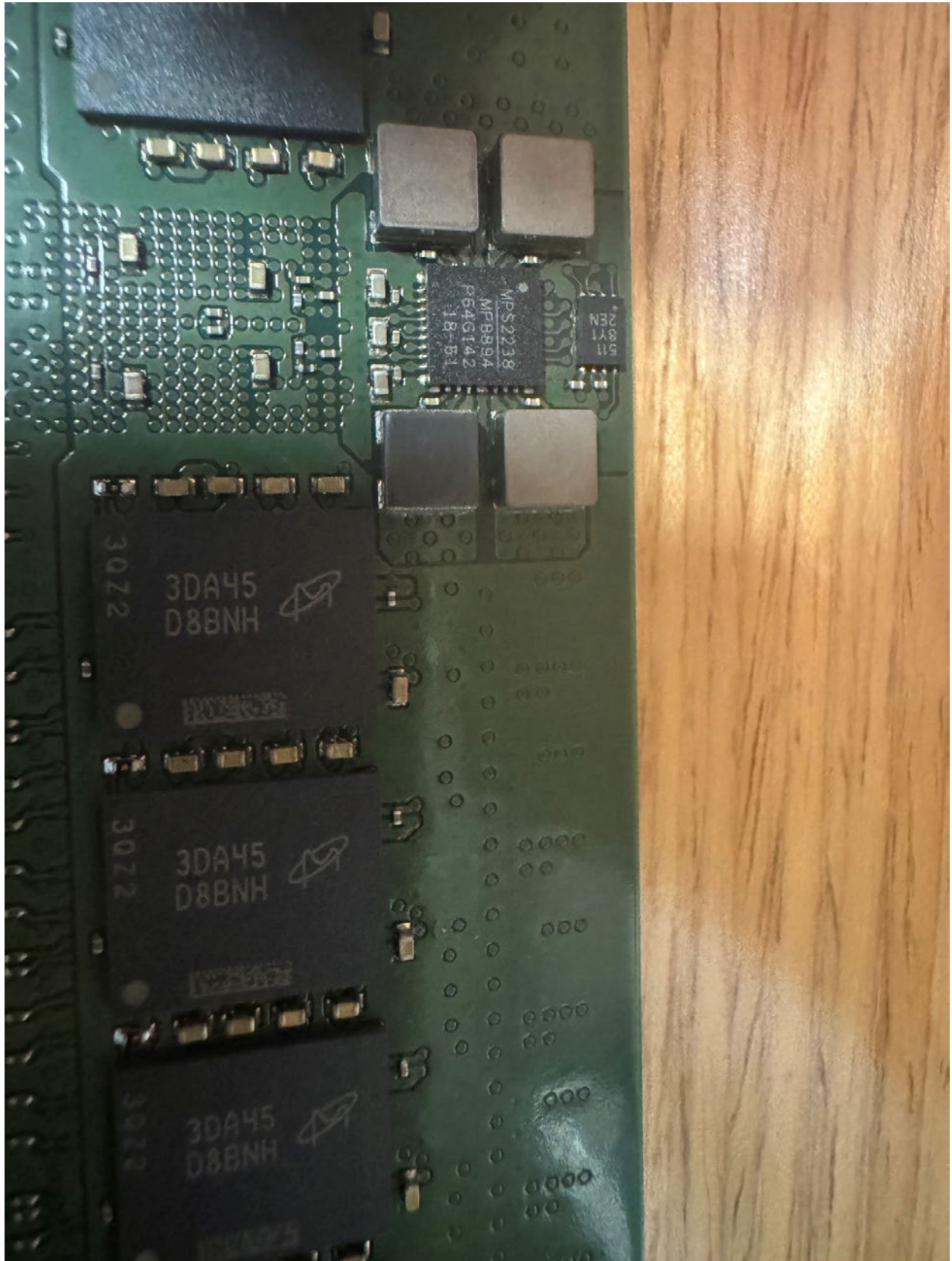
Lenovo_RDIMM_Jul26_PMIC
