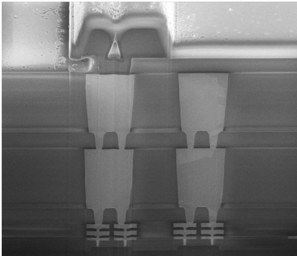
Qorvo QM81026 Guard Ring
