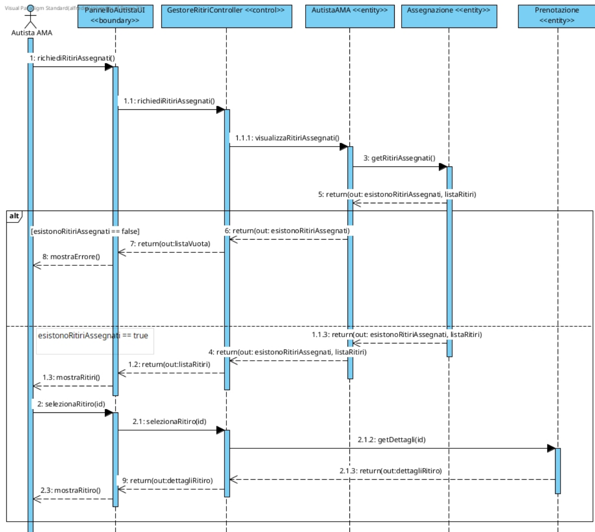
Figura 35: Sequence Diagram — Visualizzare ritiri assegnati
