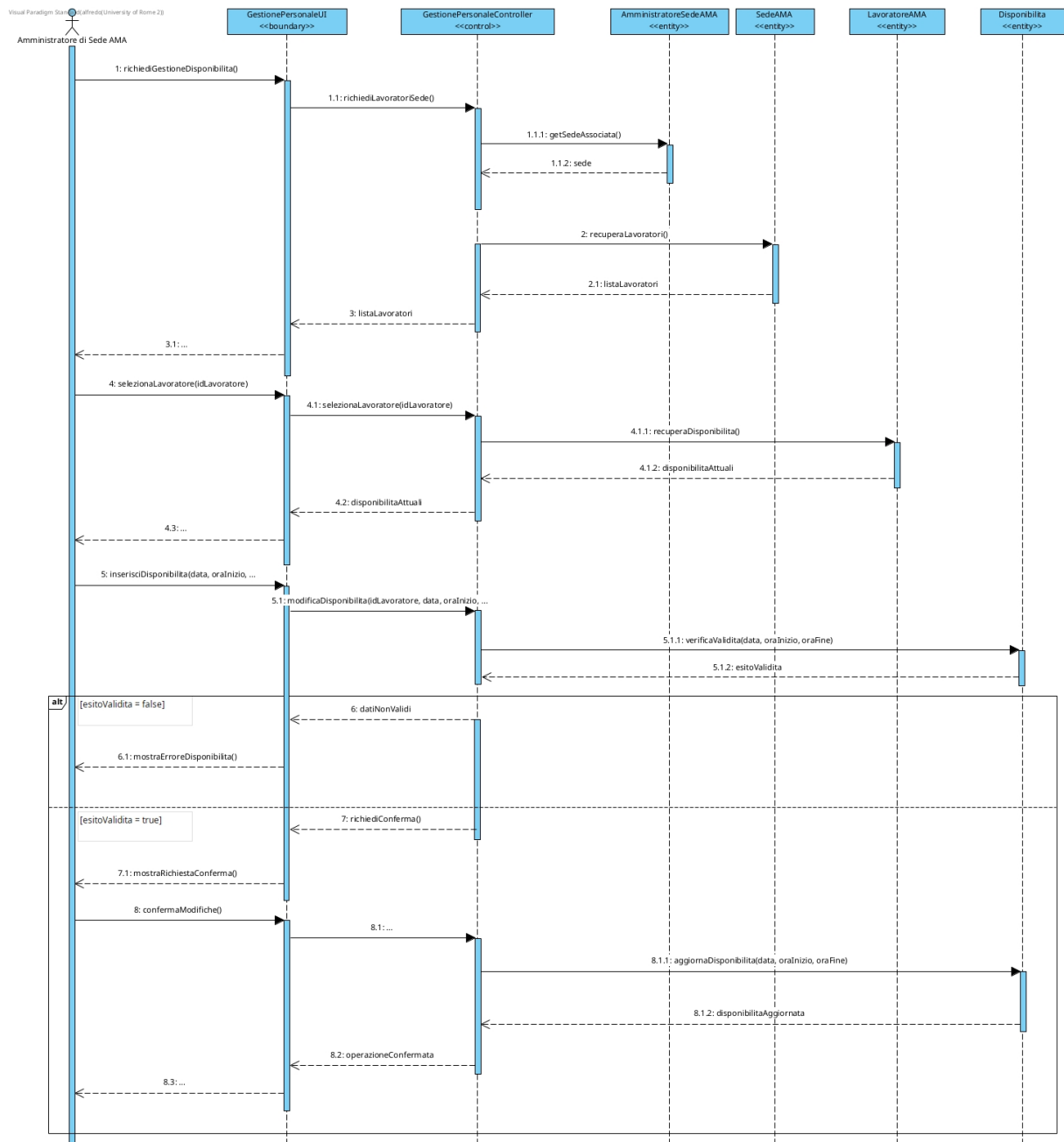
Figura 42: Sequence Diagram — Gestire disponibilità dei lavoratori
