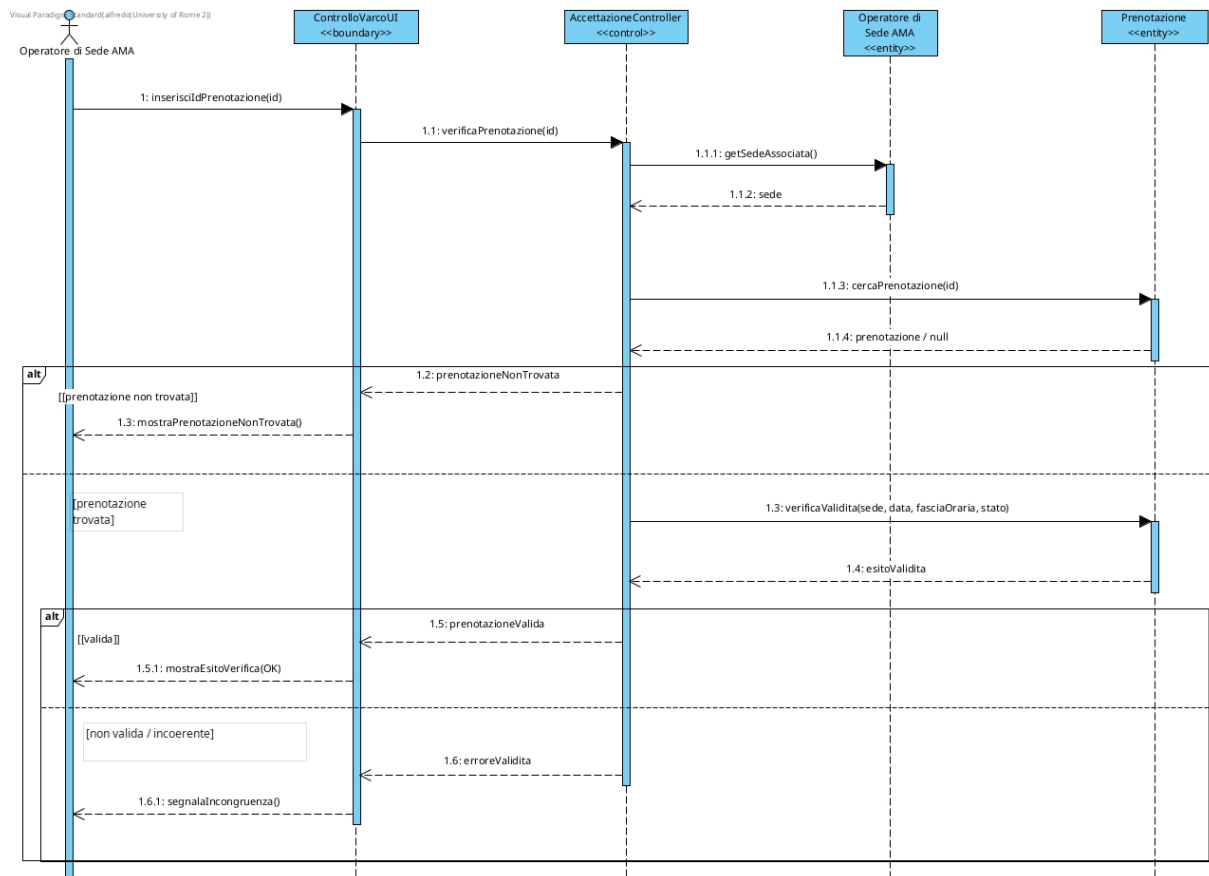
Figura 39: Sequence Diagram — Verificare prenotazione del cittadino
