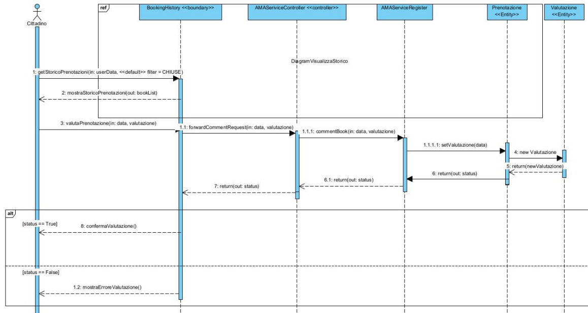
Figura 34: Sequence Diagram — Valutare il servizio
