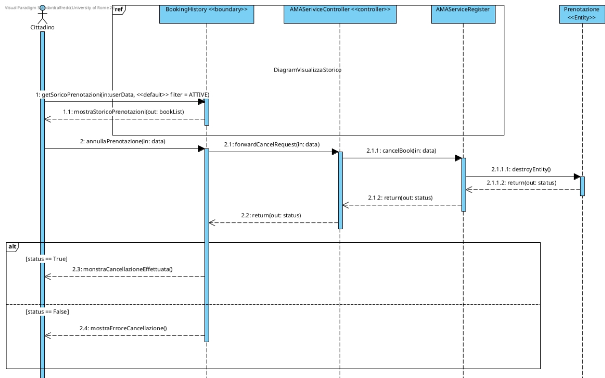
Figura 32: Sequence Diagram — Annullare prenotazione
