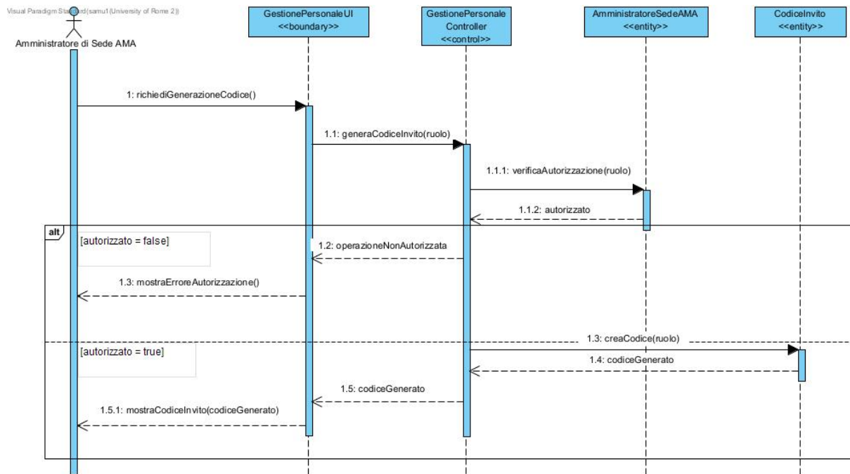
Figura 41: Sequence Diagram — Generare codice invito
