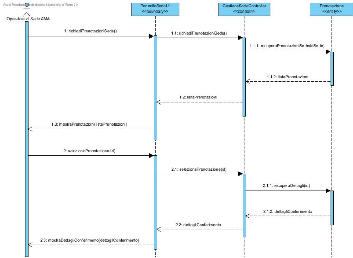
Figura 38: Sequence Diagram — Visualizzare prenotazioni della sede
