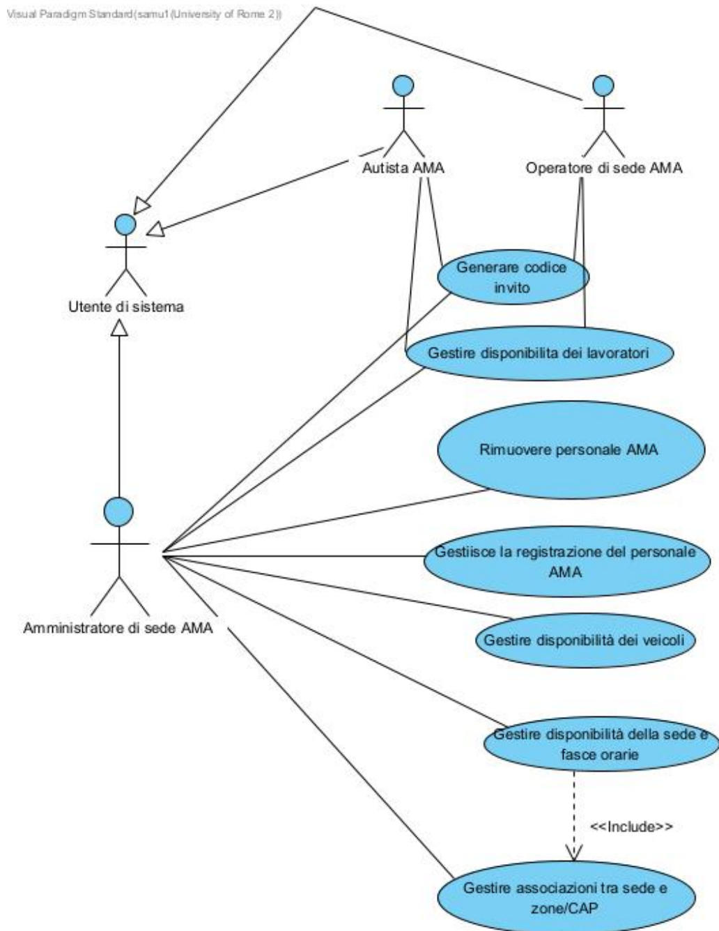
Figura 5: Use Case Diagram — Amministratore di sede AMA
