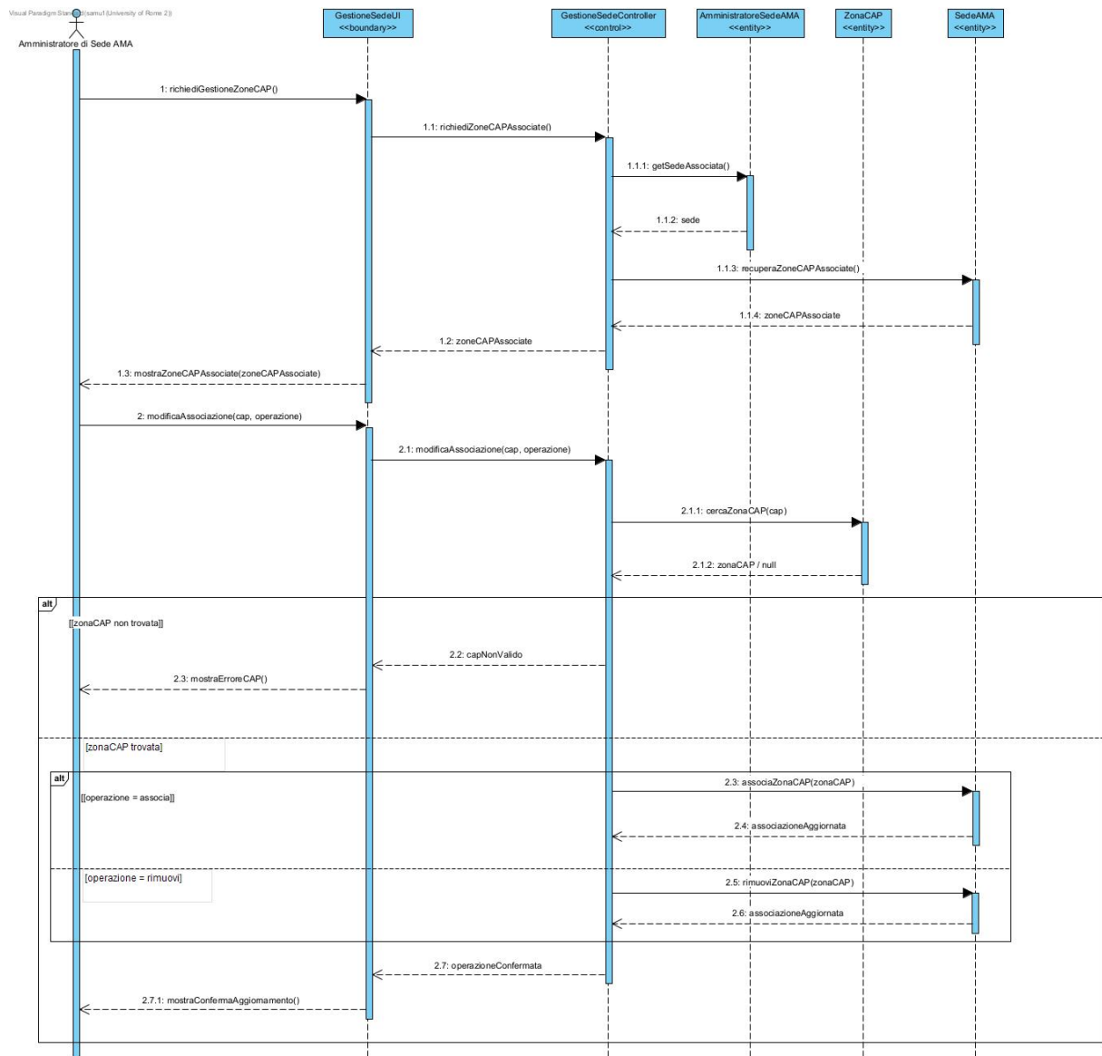
Figura 45: Sequence Diagram — Gestire associazioni tra sede e zone/CAP
