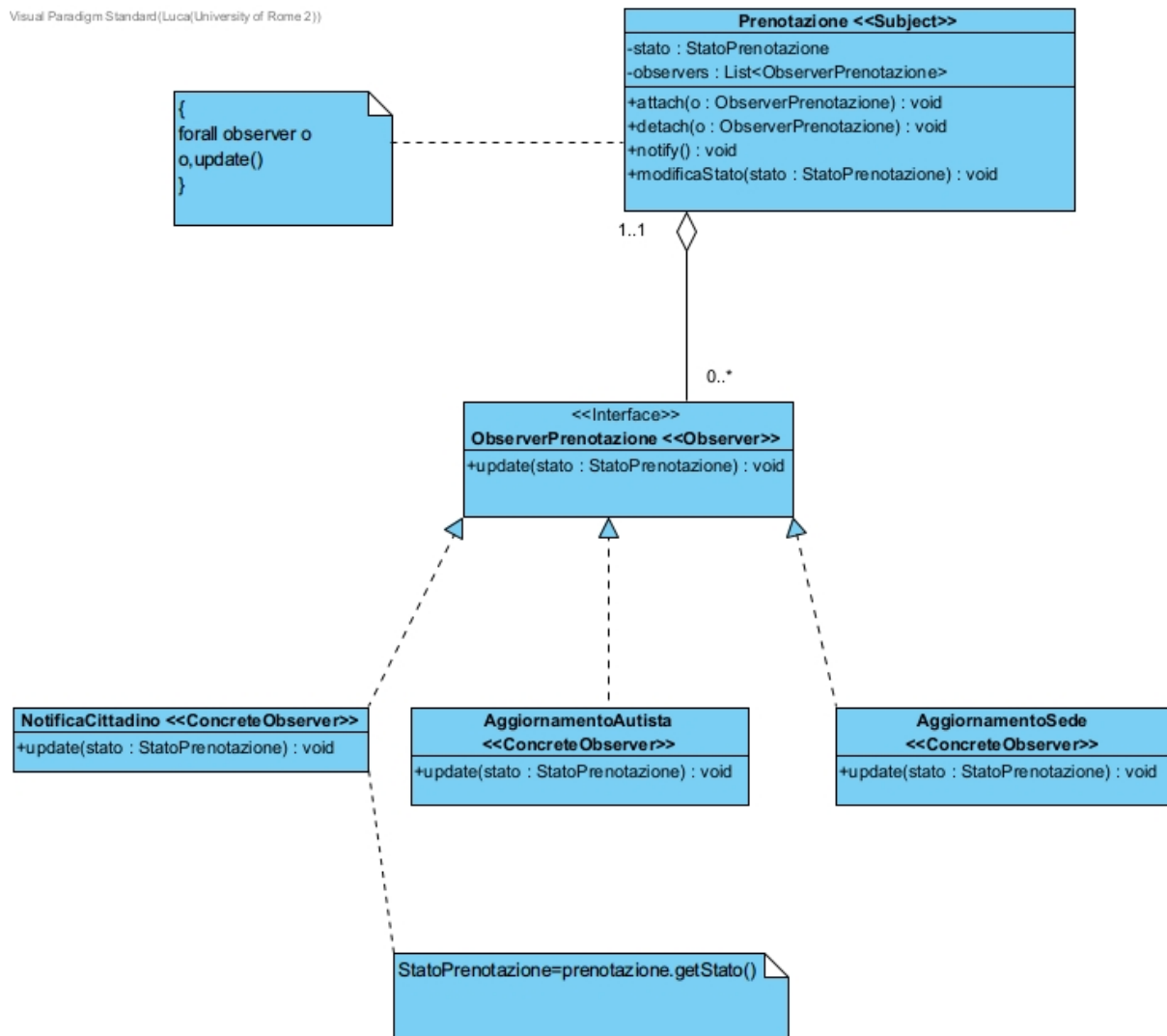
Figura 51: Struttura UML del Design Pattern Observer applicato a MyAma
