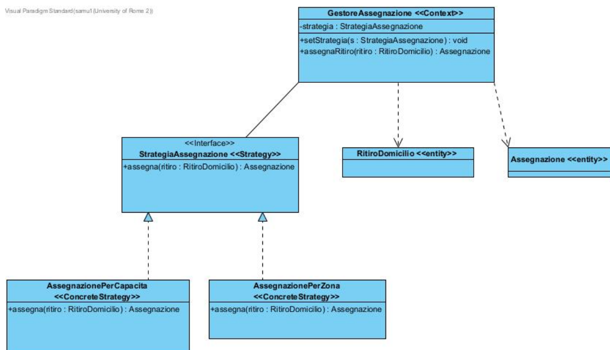
Figura 52: Struttura UML del Design Pattern Strategy per l'allocazione delle risorse
