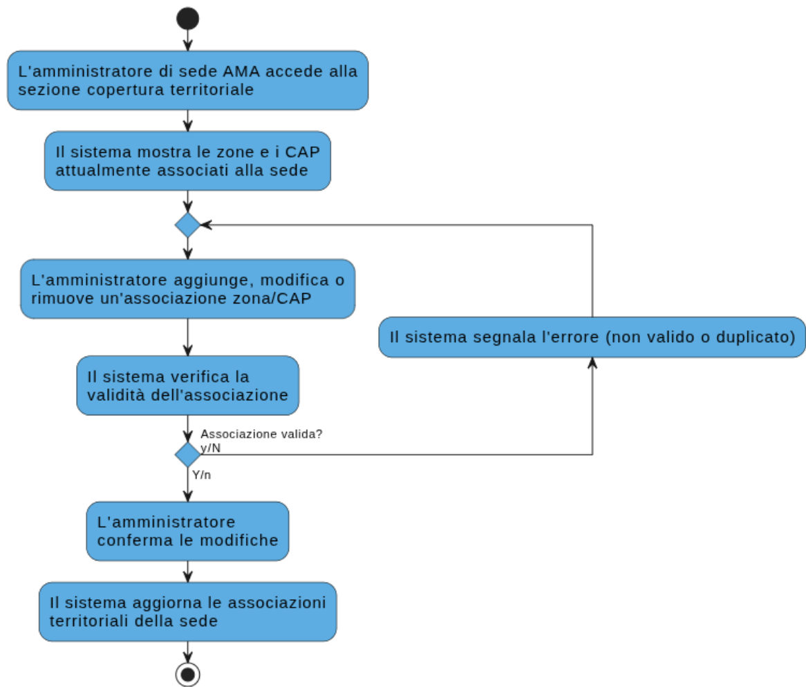
Figura 24: Activity Diagram — Gestire associazioni tra sede e zone/CAP
