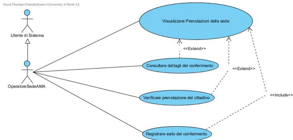
Figura 4: Use Case Diagram — Operatore di sede AMA
