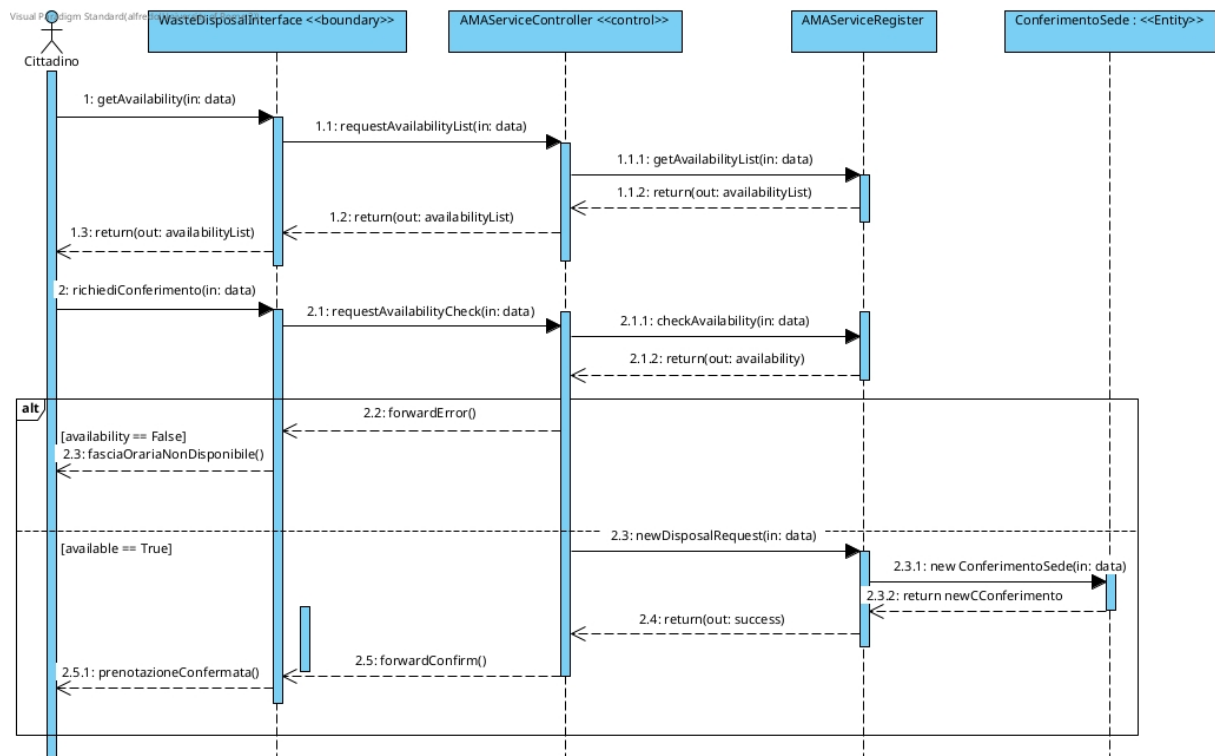
Figura 30: Sequence Diagram — Prenotare conferimento presso sede AMA
