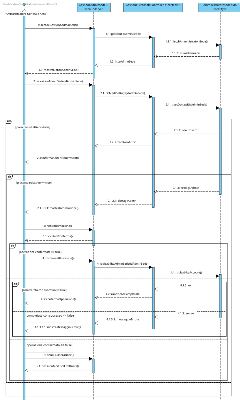
Figura 48: Sequence Diagram — Rimuovere amministratore di sede AMA
