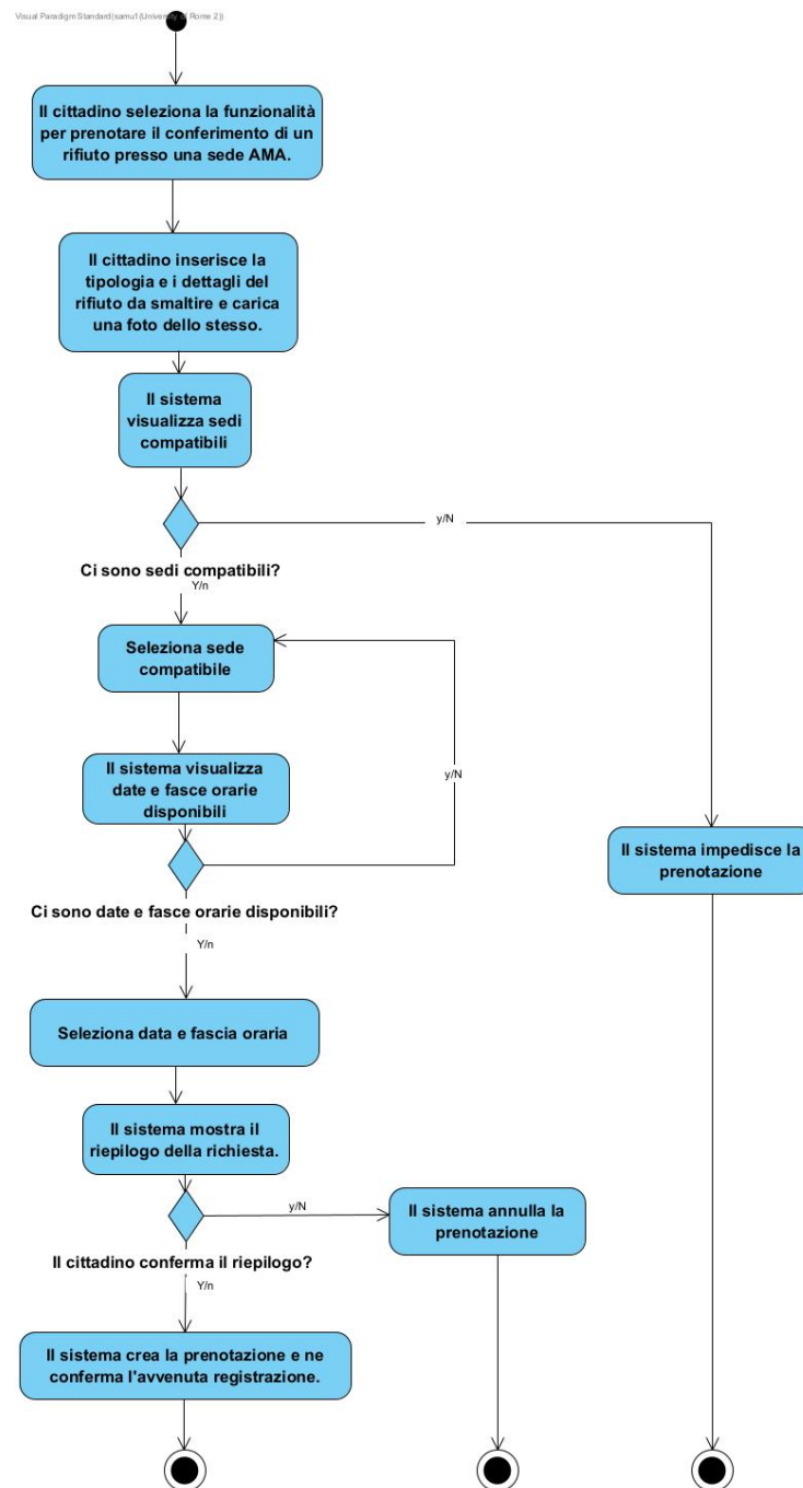
Figura 11: Activity Diagram — Prenotare conferimento in sede
