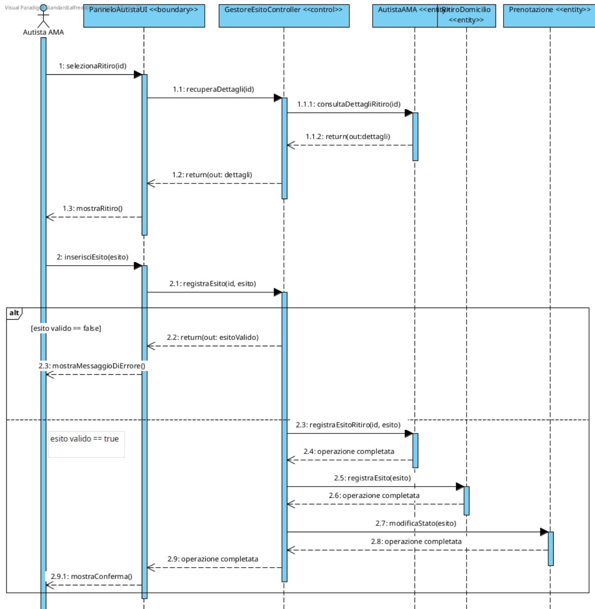
Figura 36: Sequence Diagram — Registrare esito del ritiro
