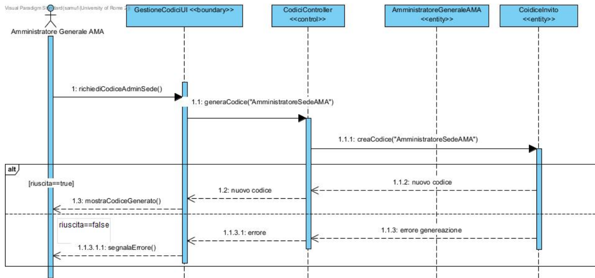
Figura 47: Sequence Diagram — Generare codice amministratore di sede
