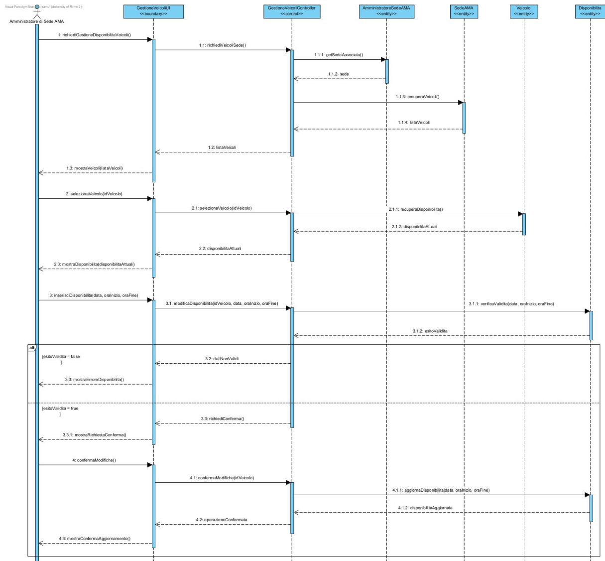
Figura 43: Sequence Diagram — Gestire disponibilit  dei veicoli
