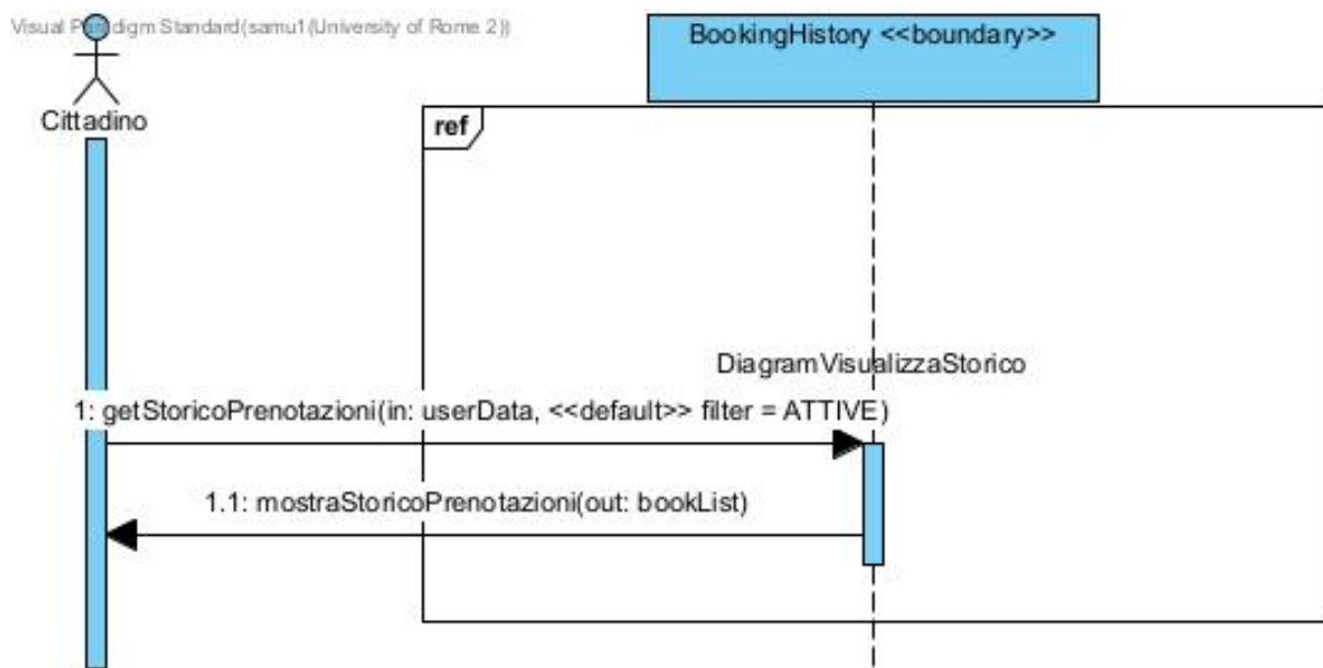
Figura 31: Sequence Diagram — Visualizzare prenotazioni attive
