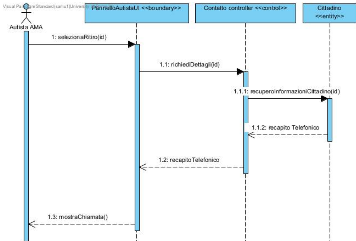
Figura 37: Sequence Diagram — Chiamare cittadino
