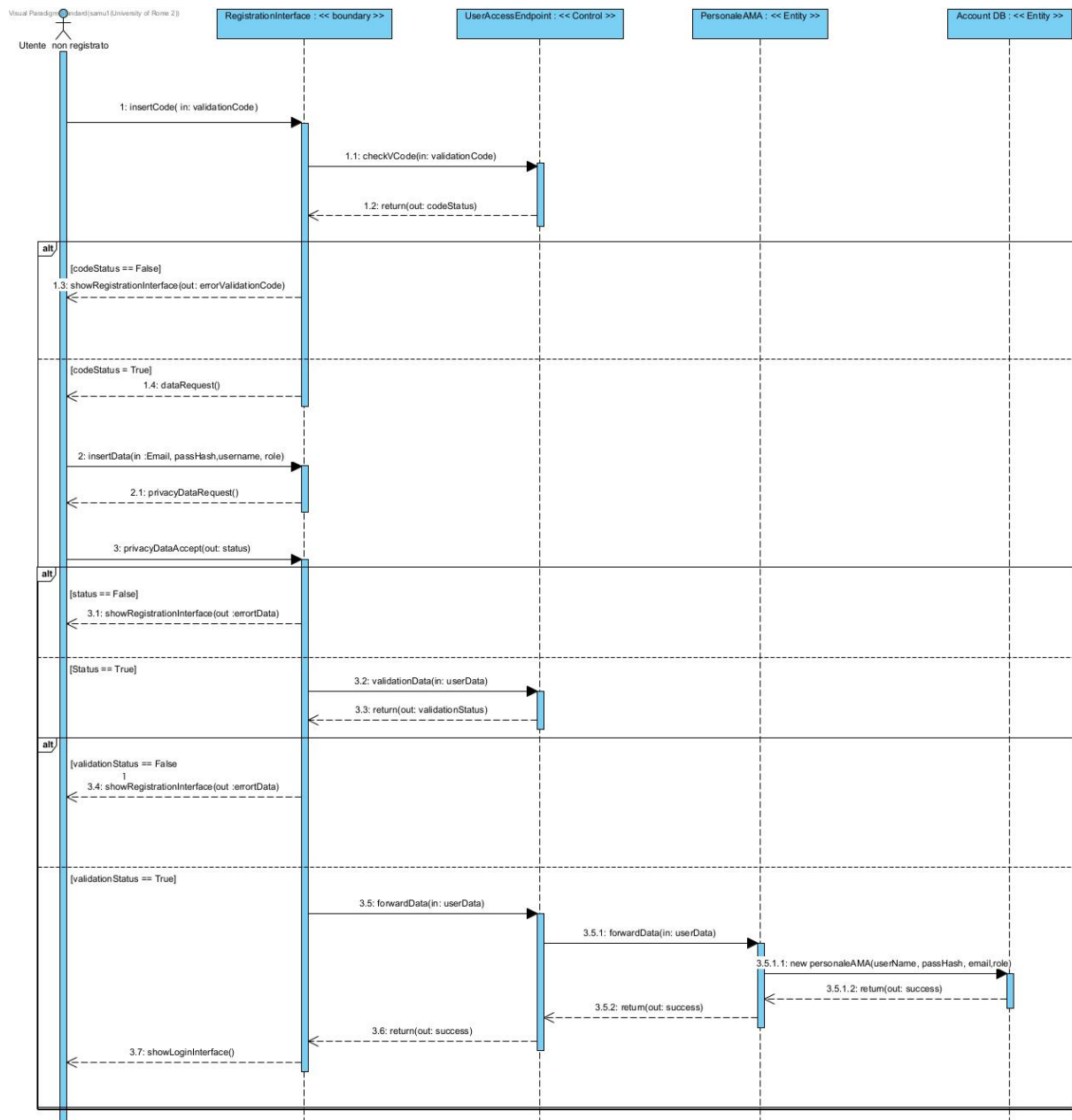
Figura 27: Sequence Diagram — Registrarsi tramite codice di invito
