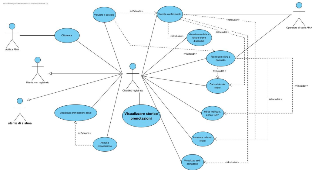
Figura 2: Use Case Diagram — Cittadino registrato
