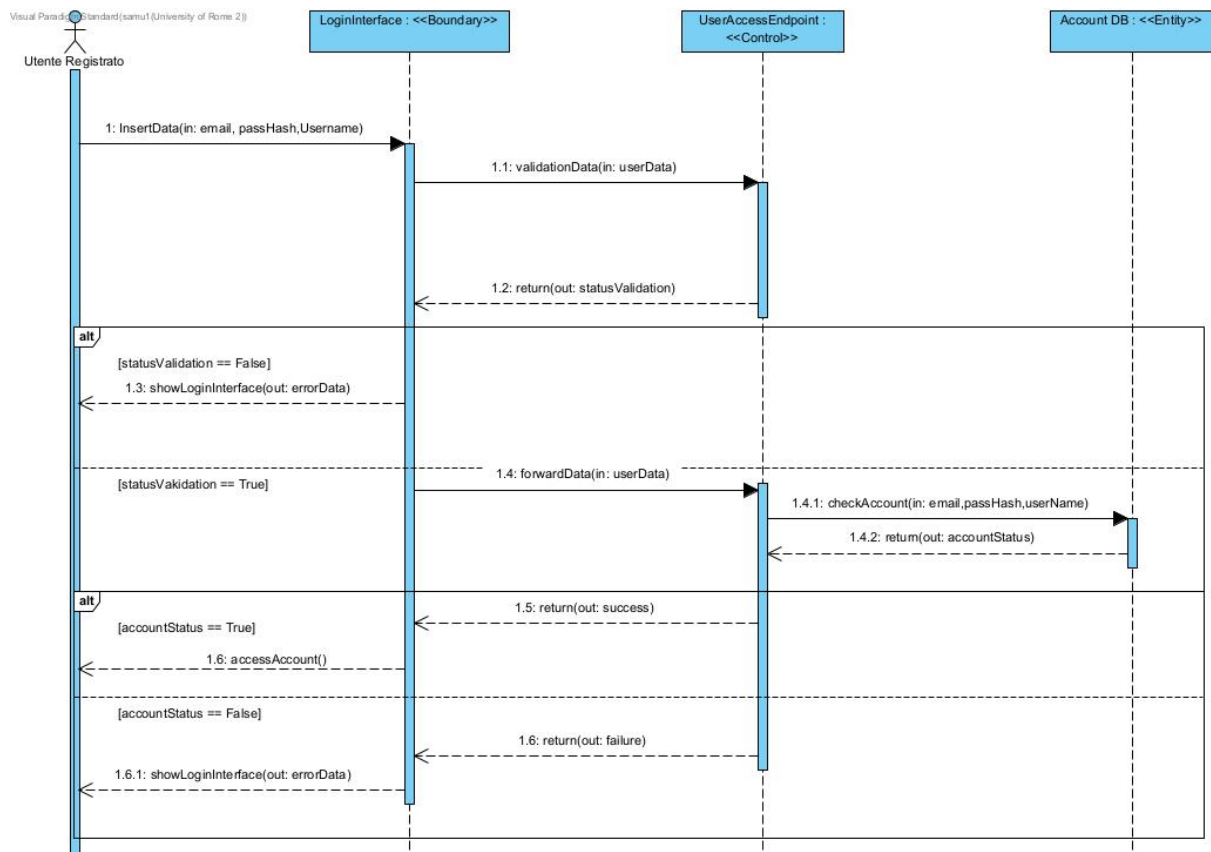
Figura 28: Sequence Diagram — Effettuare accesso
