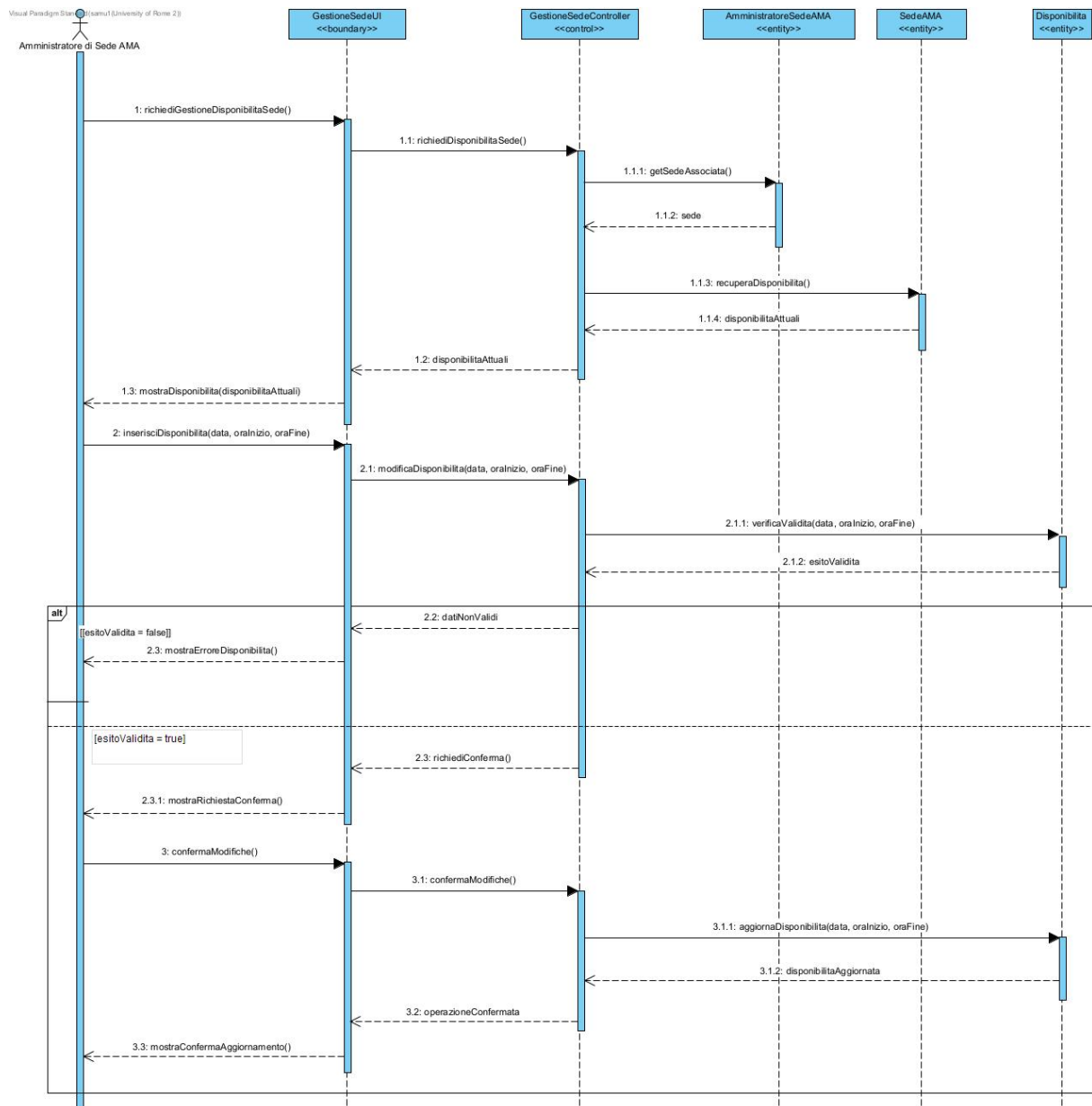
Figura 44: Sequence Diagram — Gestire disponibilità della sede e fasce orarie
