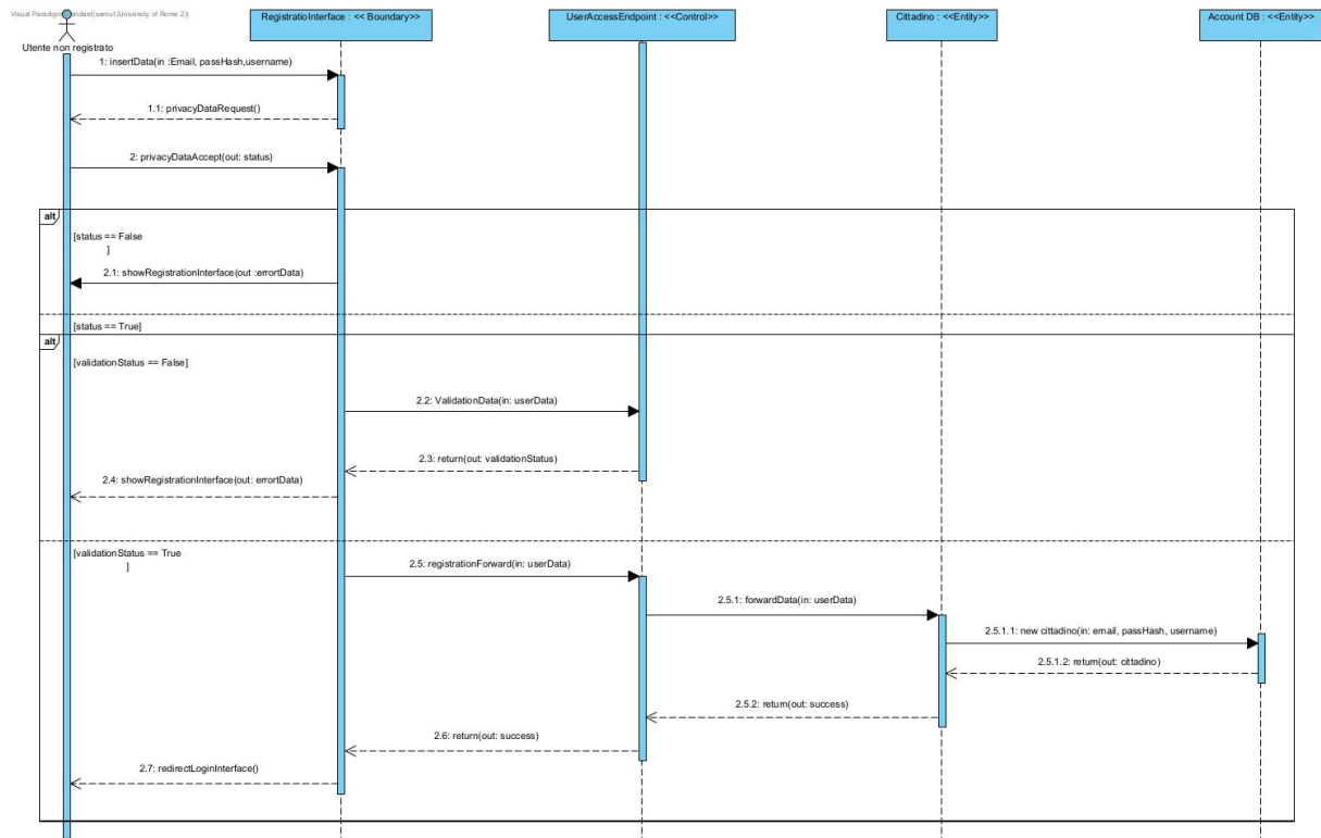
Figura 26: Sequence Diagram — Registrarsi come cittadino
