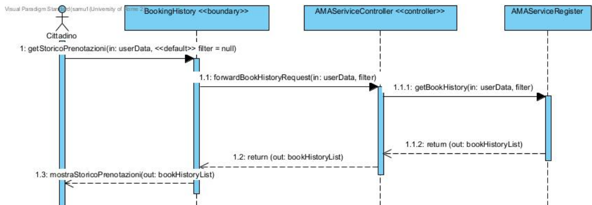
Figura 33: Sequence Diagram — Visualizzare storico prenotazioni
