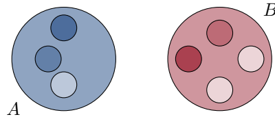
Figure 3.2: Disjunkte Mengen.
