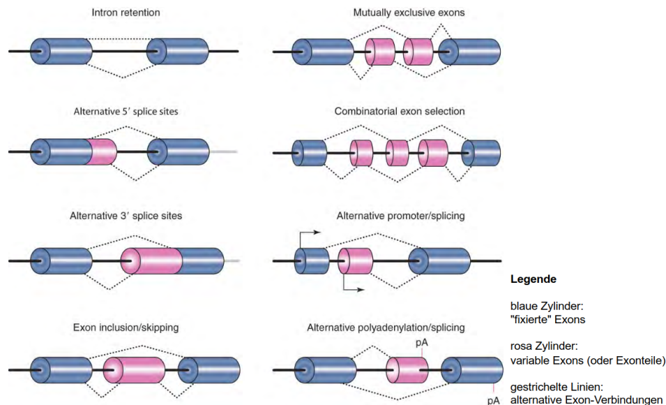
Abbildung 5.6: Arten von alternativem Spleißen
