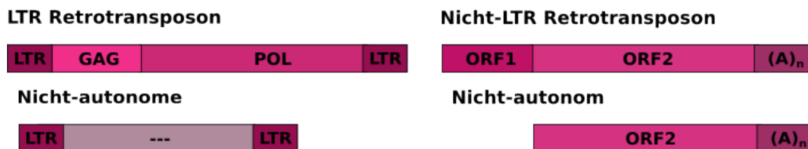
Abbildung 6.2: Kategorisierung auf Aufbau von Transposons
