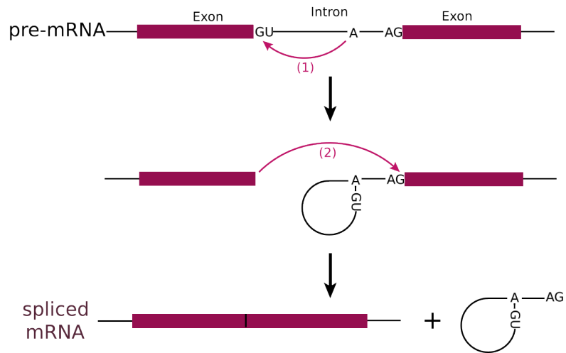
Abbildung 5.3: Adaptiert von BCSteve
