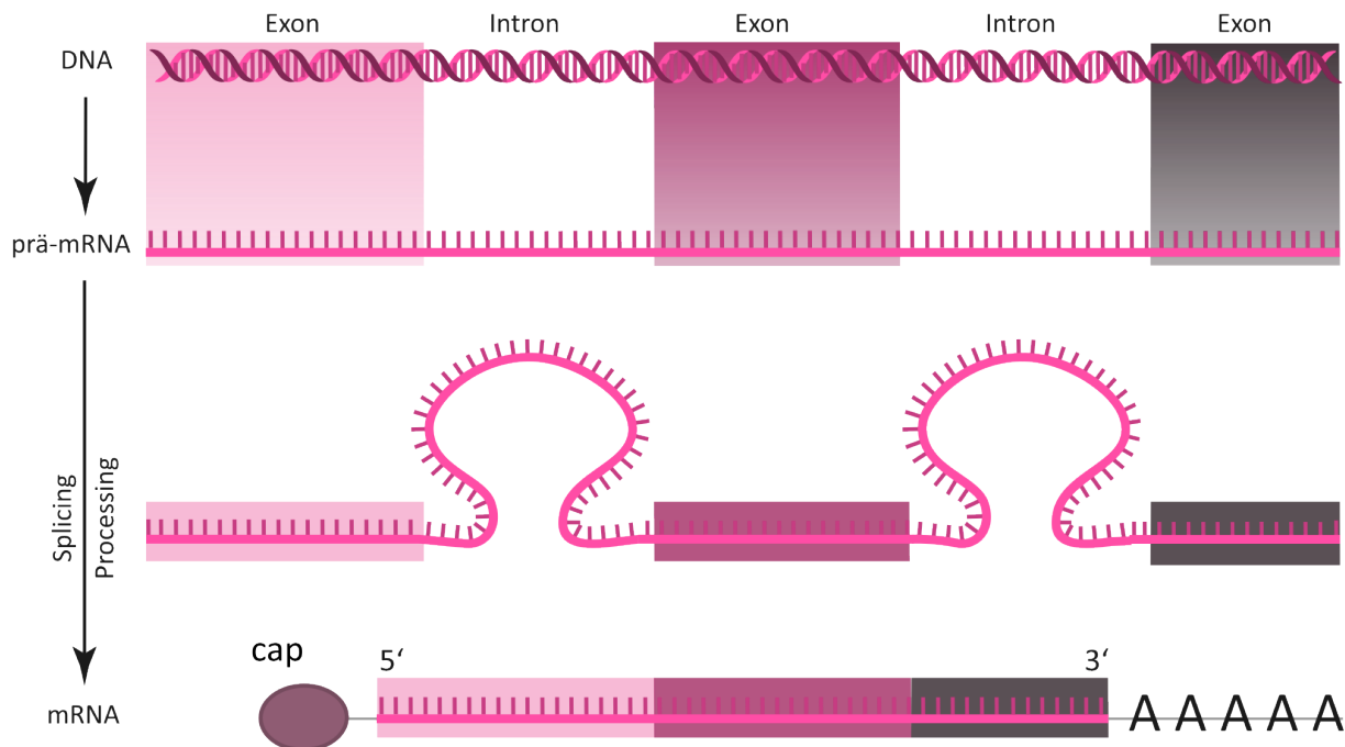
Abbildung 5.1: Spleißen (Adaptiert von abipass.de )
