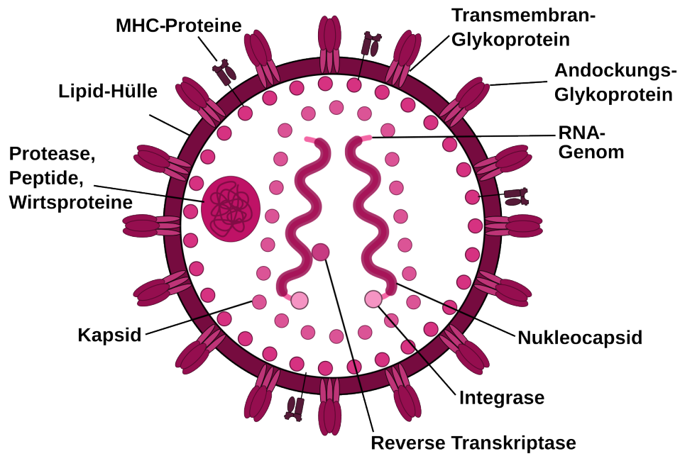
Abbildung 6.4: Schematischer Aufbau eines Retrovirus nach dem HI-Virus.
