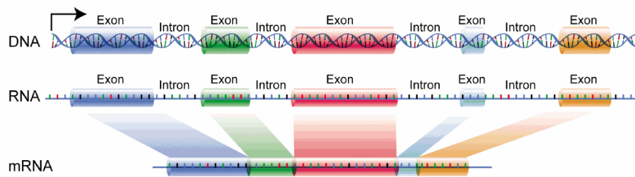
Abbildung 5.1: Spleißen
