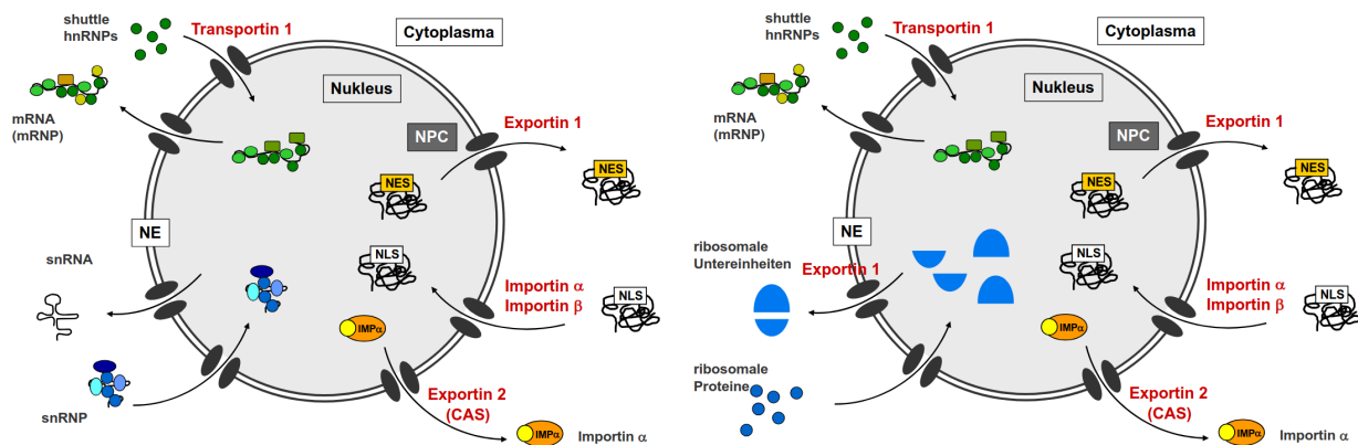
(a) snRNA/snRNP-Transport: snRNAs werden zunächst exportiert, dort zu einem kleinen nukleären Ribonukleoprotein-Komplex (snRNP) umgewandelt und diese in die Zelle re-importiert. (b) Ribosomenbiogenese: Im Nukleolus werden rRNA hergestellt und ribosomale Proteine eingebaut. Es entstehen die kleine und große ribosomale Untereinheiten. Diese werden durch Exportin 1 aus dem Kern exportiert.
