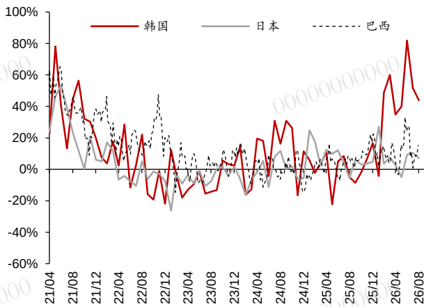
图表30：8月日本出口同比增速均较前月同期回落
