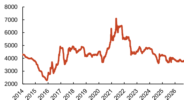
图 40：冷轧板价格 (元/吨)
