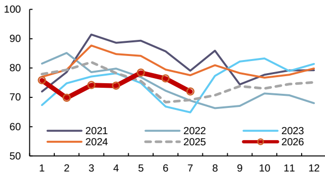
图 33：钛白粉月开工率（%）
