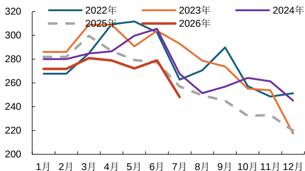
图 21：全国粗钢日均产量（万吨）
