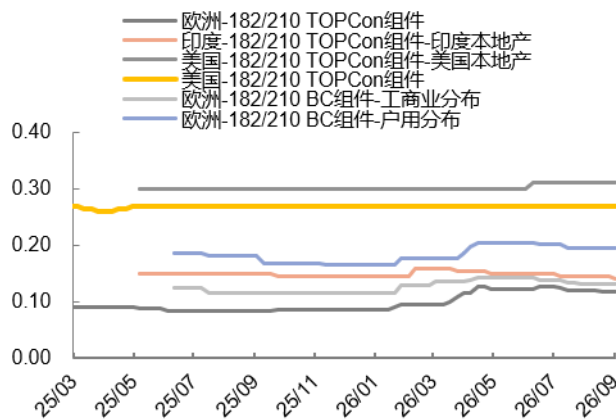
图表8：各区域组件价格（USD/W）
