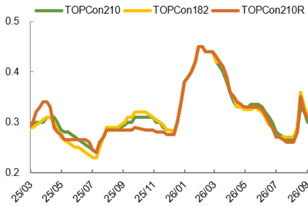
图表6：电池片价格（元/W）
