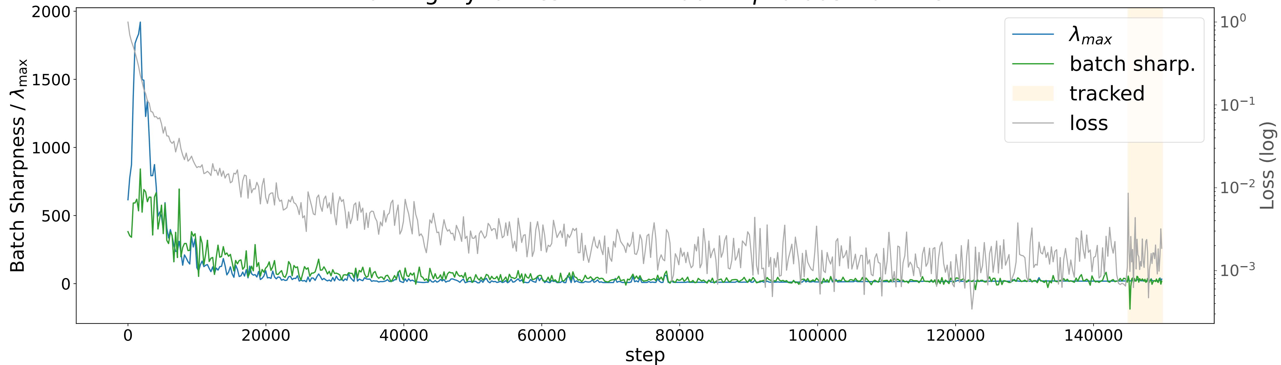
Training Dynamics — ViT · Muon · \eta=0.003 · b=128
