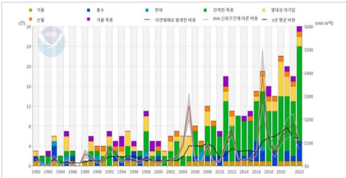
〈미국 유형별 피해 규모 10억 달러 이상의 자연재해 건수 및 전체 피해금액〉
