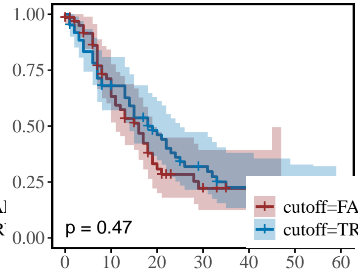
GEO_PAAD
