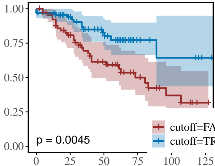
GEO_LUAD
