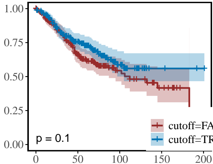
GEO_COAD
