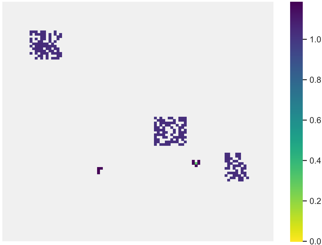
Sp. 0 (pop. size: 2324, range size: 226)
