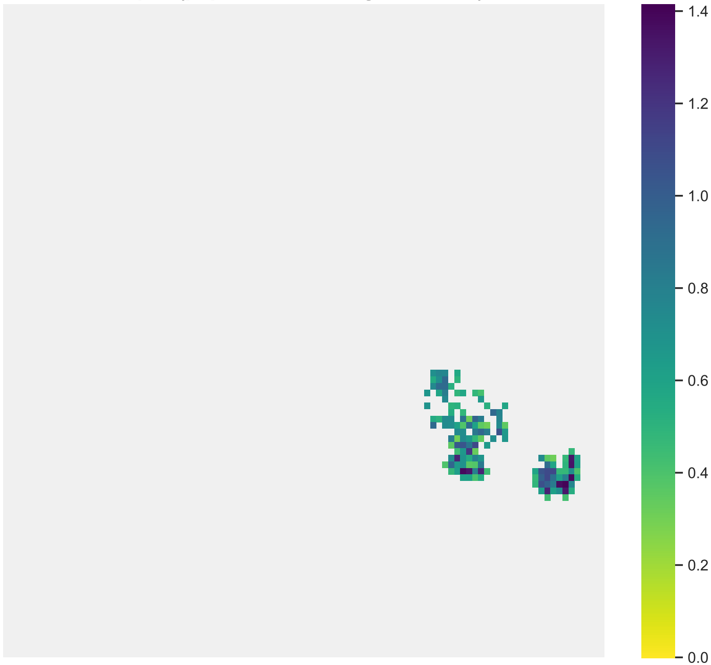
Sp. 7 (pop. size: 839, range size: 142)
