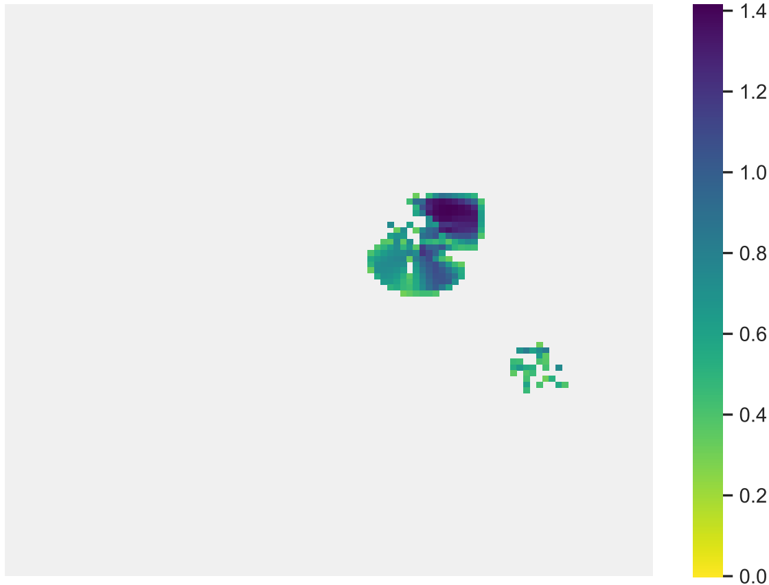
Sp. 5 (pop. size: 1795, range size: 243)
