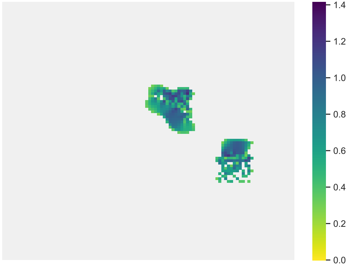
Sp. 1 (pop. size: 1822, range size: 360)
