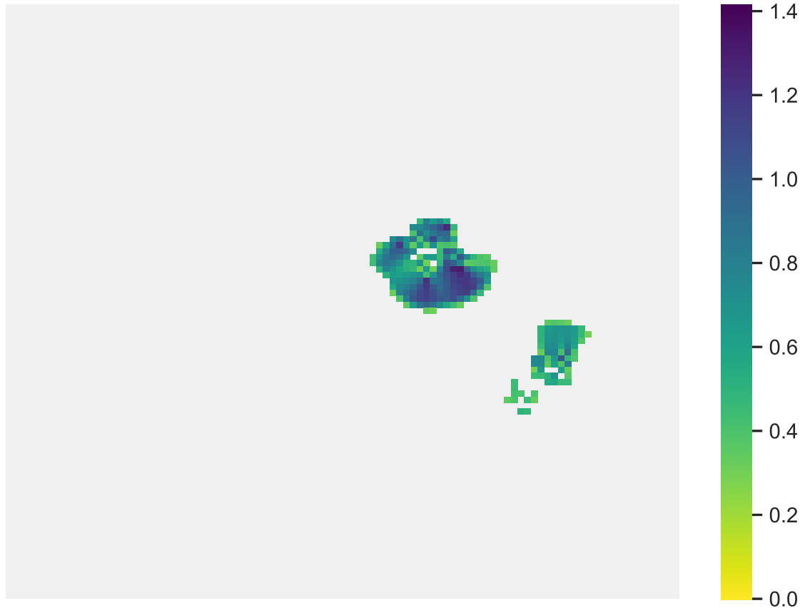
Sp. 4 (pop. size: 1402, range size: 262)
