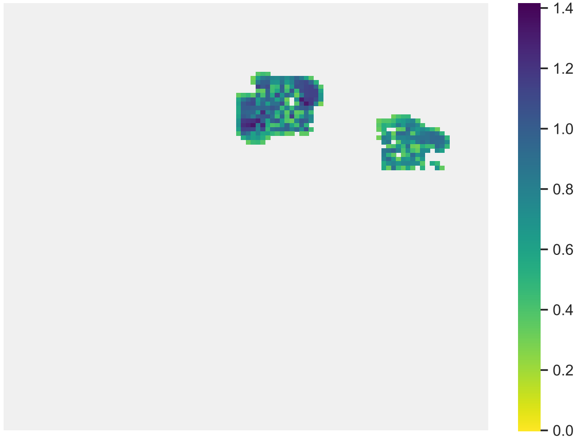
Sp. 2 (pop. size: 2056, range size: 367)
