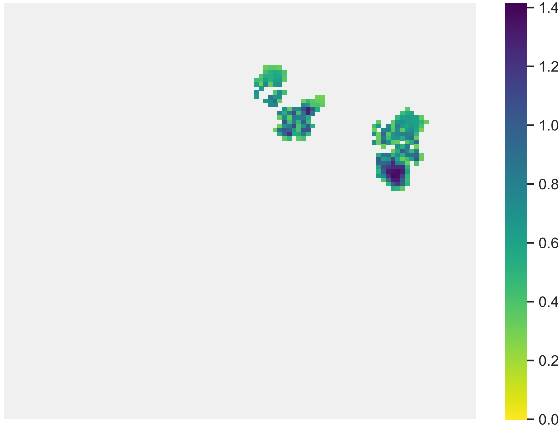
Sp. 6 (pop. size: 1294, range size: 252)
