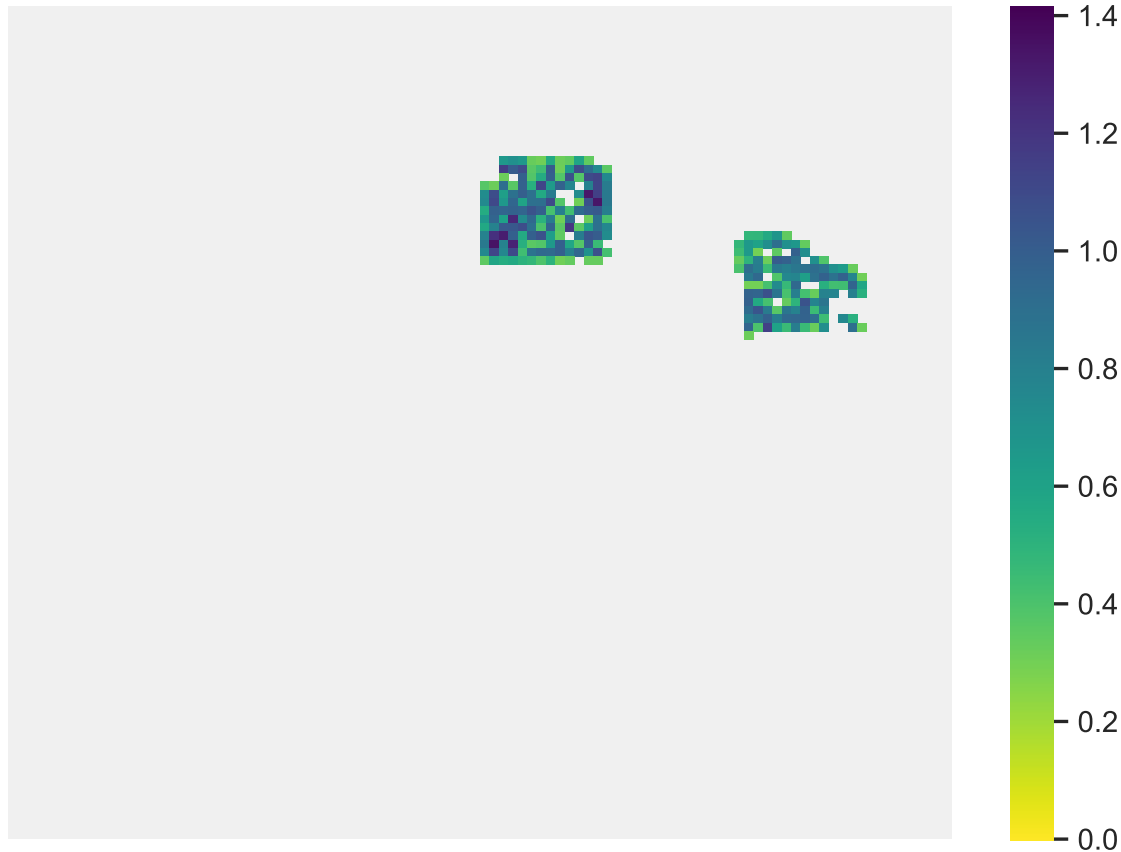
Sp. 2 (pop. size: 1565, range size: 280)
