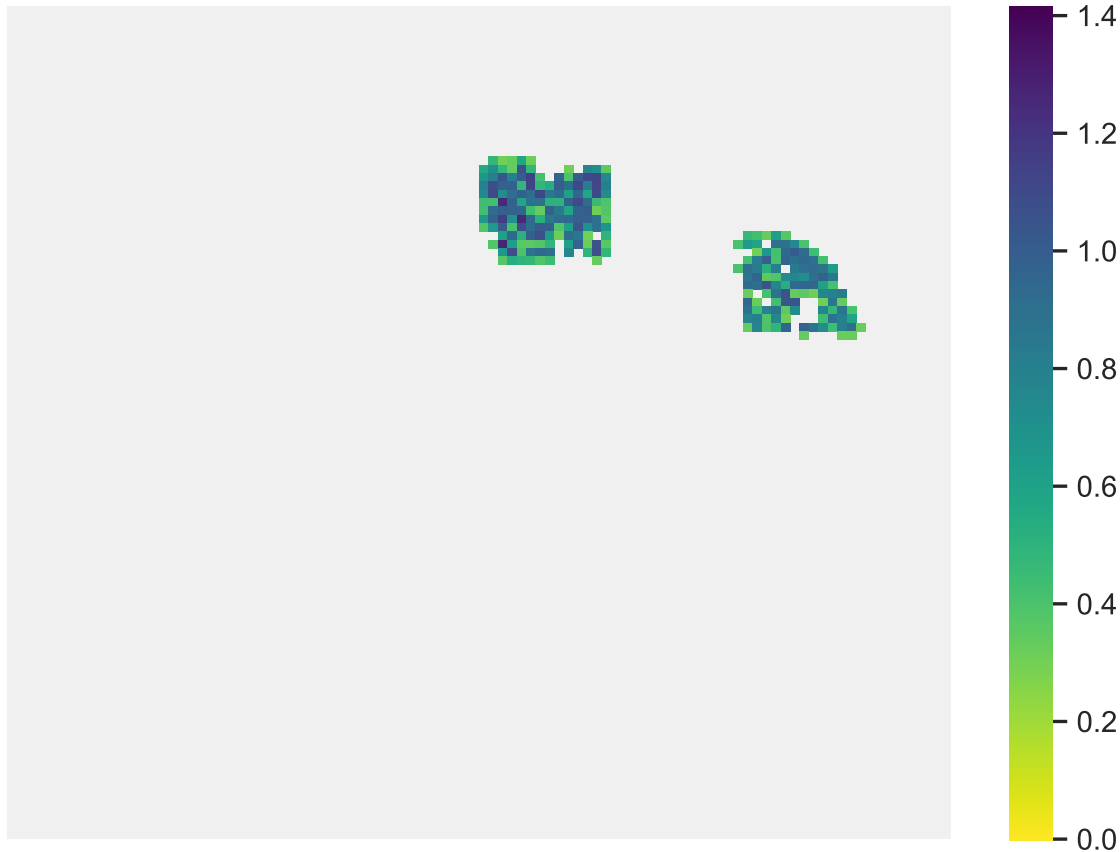
Sp. 1 (pop. size: 1396, range size: 262)
