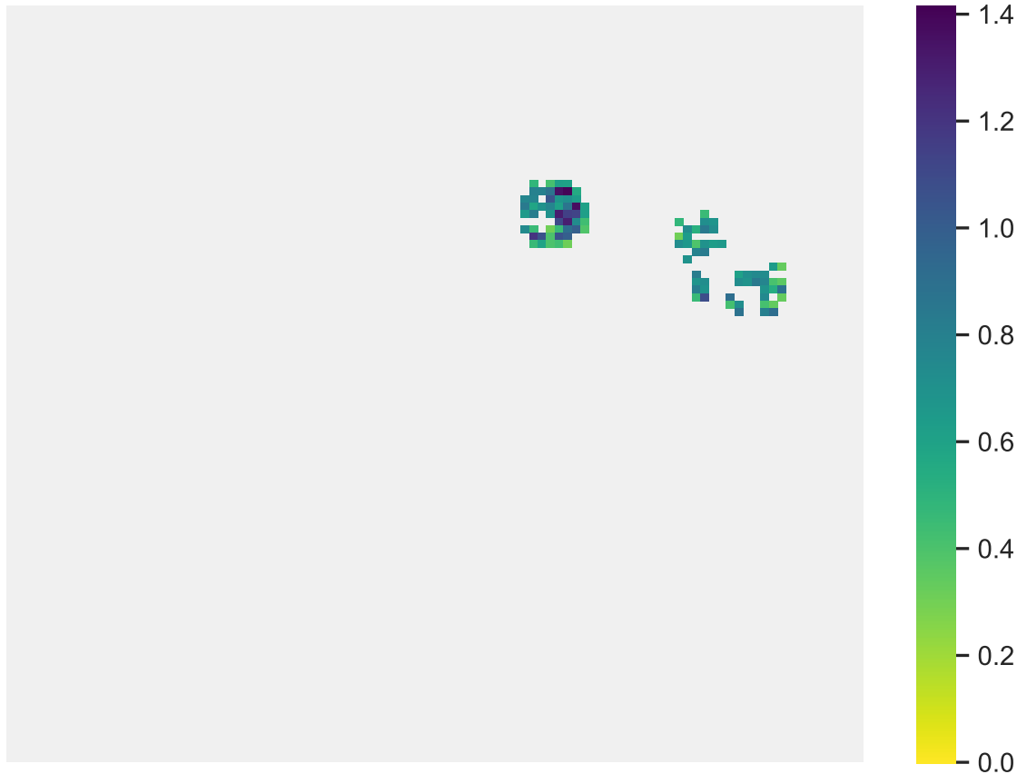
Sp. 4 (pop. size: 597, range size: 103)
