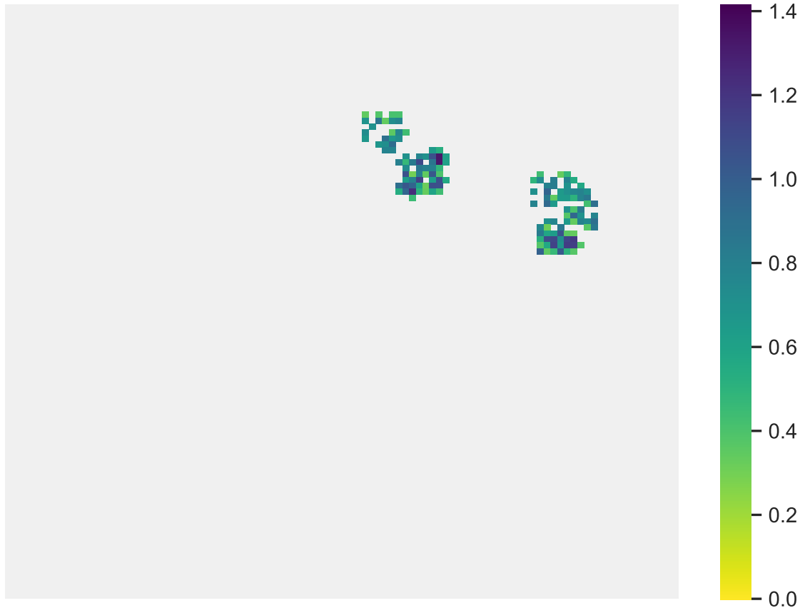
Sp. 6 (pop. size: 810, range size: 145)
