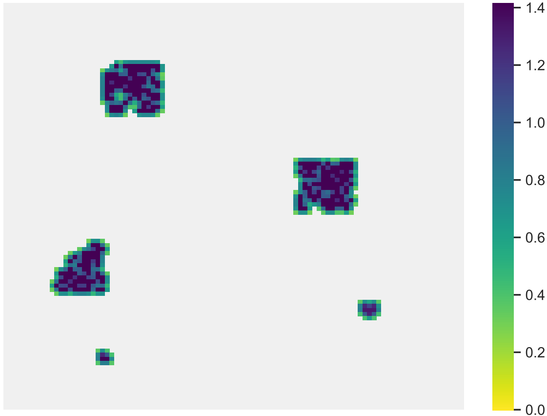
Sp. 0 (pop. size: 7724, range size: 545)
