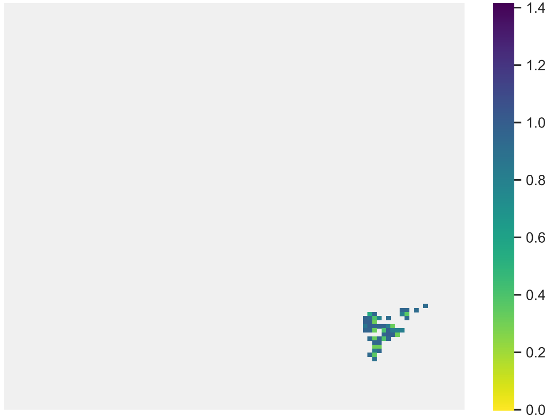
Sp. 3 (pop. size: 330, range size: 50)
