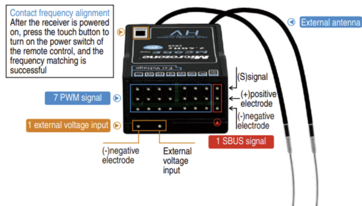
Slika 4: Shema priključkov sprejemnika iz dokumentacije, ki sem jo uporabil pri načrtovanju GPIO povezav.
