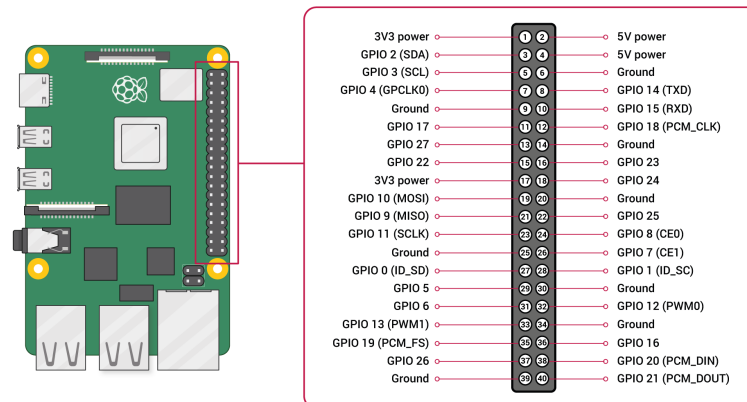
Slika 3: Skica Raspberry Pi z označenimi pini in navedenimi funkcijami pinov.
