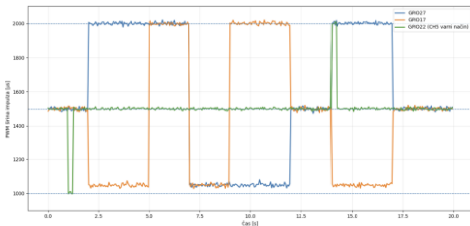
Slika 5: Graf meritev PWM-signalov posameznih kanalov, izmerjenih z Arduinom in Serial Plotterjem v Arduino IDE.
