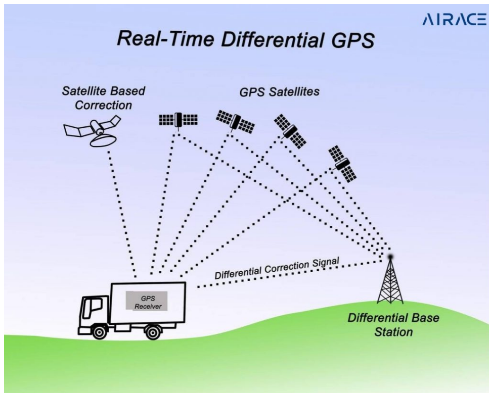
Slika 7: Prikaz principa delovanja diferencialnega GPS in popravkov NTRIP (AIRace, 2024).
