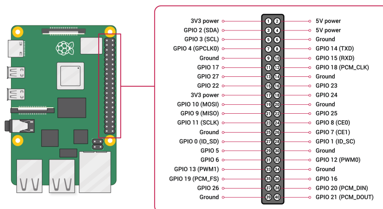
Slika 5: Skica Raspberry Pi z označenimi pini in navedenim funkcijami PINOV, ki sem jih uporabljal pri povezovanju sistema.
