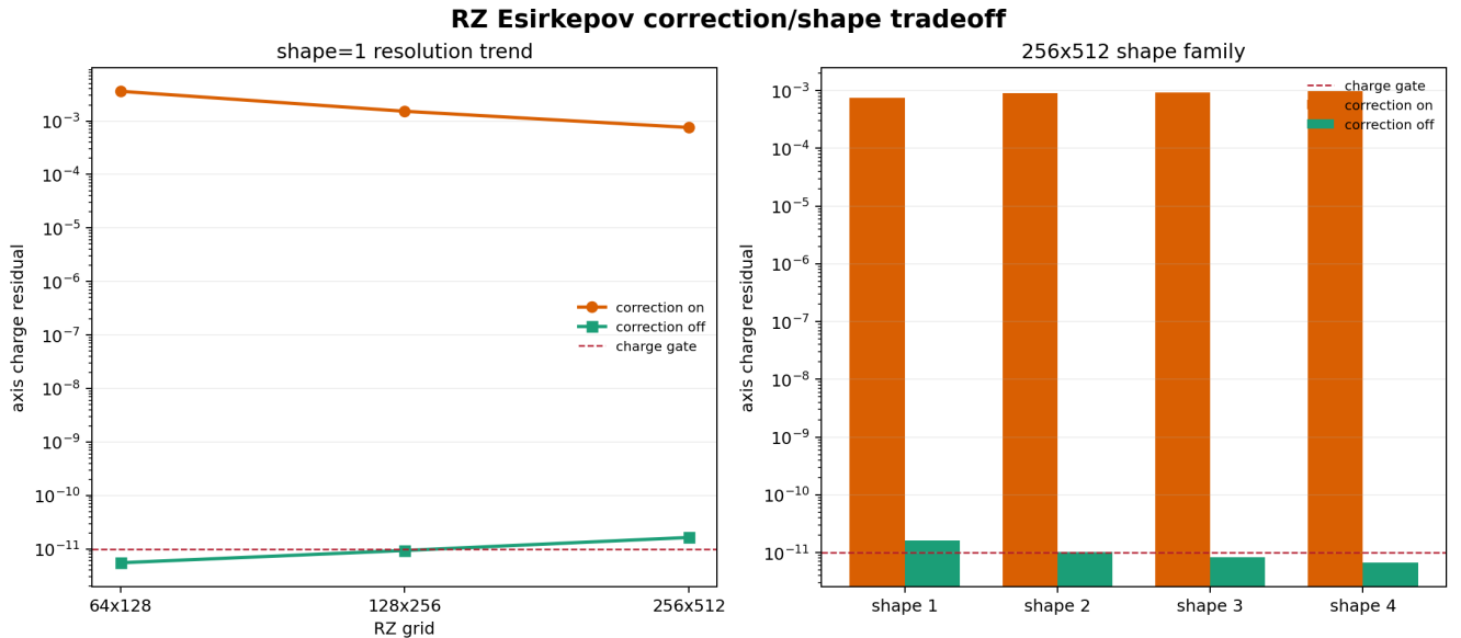
图 5-3: RZ Esirkepov axis-correction/shape tradeoff。左侧是 shape=1 的三档分辨率趋势, 右侧是 256x512 下 shape=1/2/3/4 的 correction-on/off 对照; 红色虚线是 1e-11 charge gate。所有 field gate 均通过, 但 correction-on 的 axis residual 仍约为 0(1e-3) , correction-off 的 charge 结果随 shape 变化, 不能据此修改全局默认值或宣称正式收敛阶。
