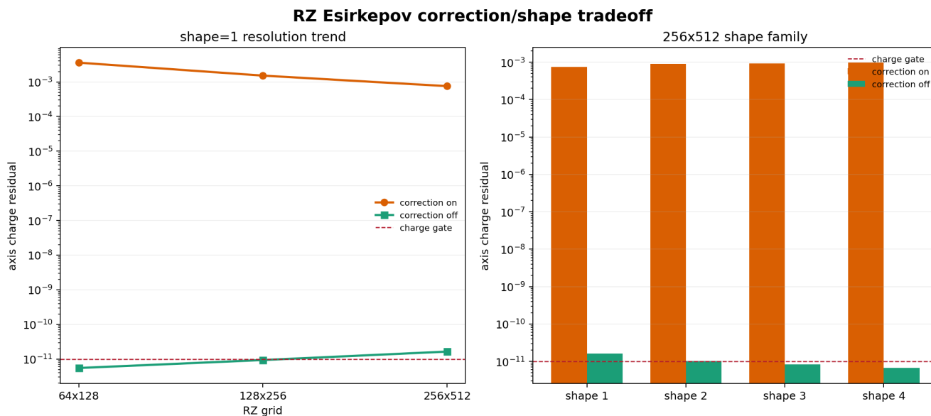
图 5-3: RZ Esirkepov axis-correction/shape tradeoff. 左侧是 shape=1 的三档分辨率趋势, 右侧是 256x512 下 shape=1/2/3/4 的 correction-on/off 对照; 红色虚线是 1e-11 charge gate. 所有 field gate 均通过, 但 correction-on 的 axis residual 仍约为 0(1e-3), correction-off 的 charge 结果随 shape 变化, 不能据此修改全局默认值或宣称正式收敛阶.
